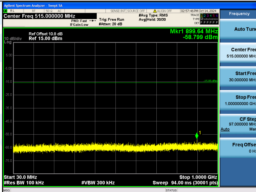
11G-Ant1-2437-30~1000-PASS
