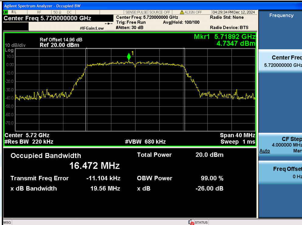
11A-Ant1-5720
