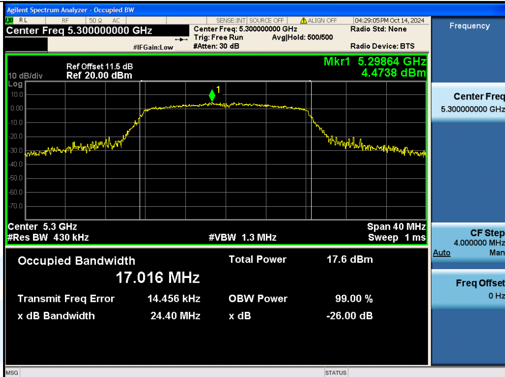
11A-Ant1-5300
