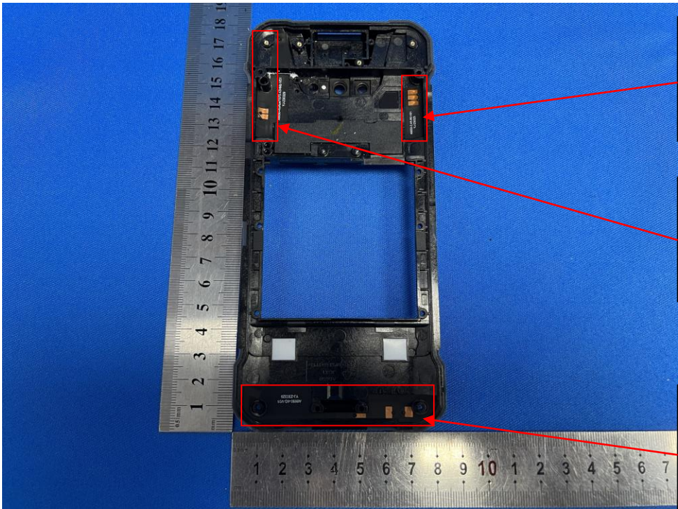
BT/WIFI antenna
