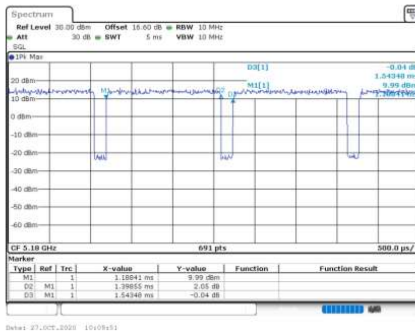
802.11a
