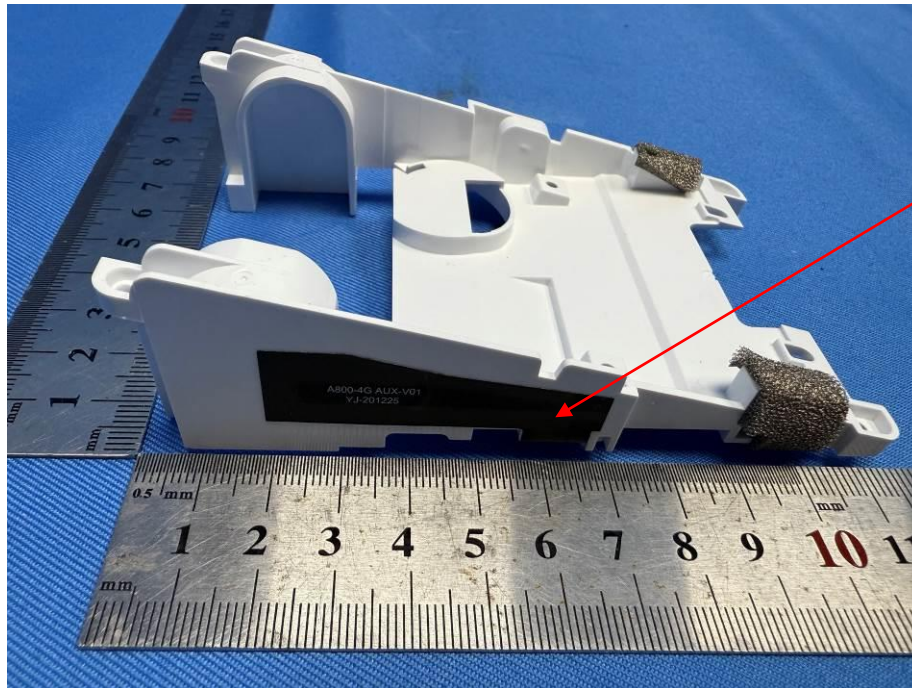
WWAN div antenna
