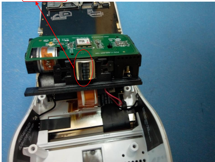
NFC ANT.
