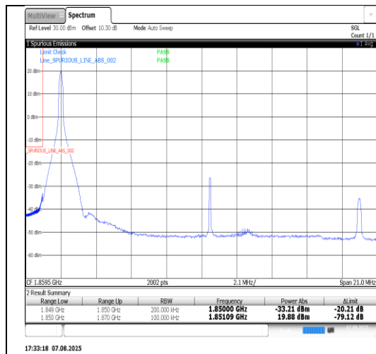
Band2-20MHz-16QAM-18700-100RB#0-PASS
