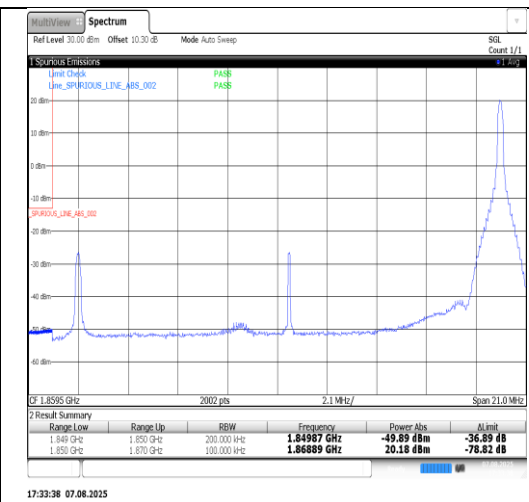
Band2-20MHz-16QAM-19100-1RB#0-PASS
