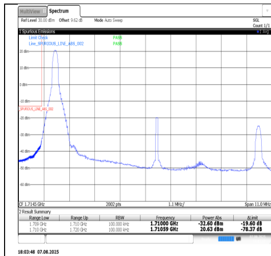
Band4-10MHz-QPSK-20000-50RB#0-PASS
