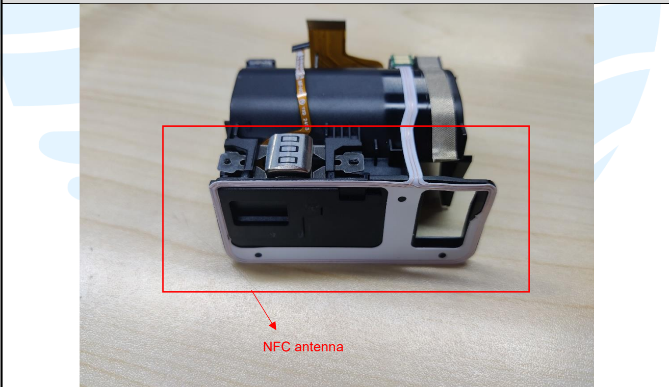
EUT Photo
