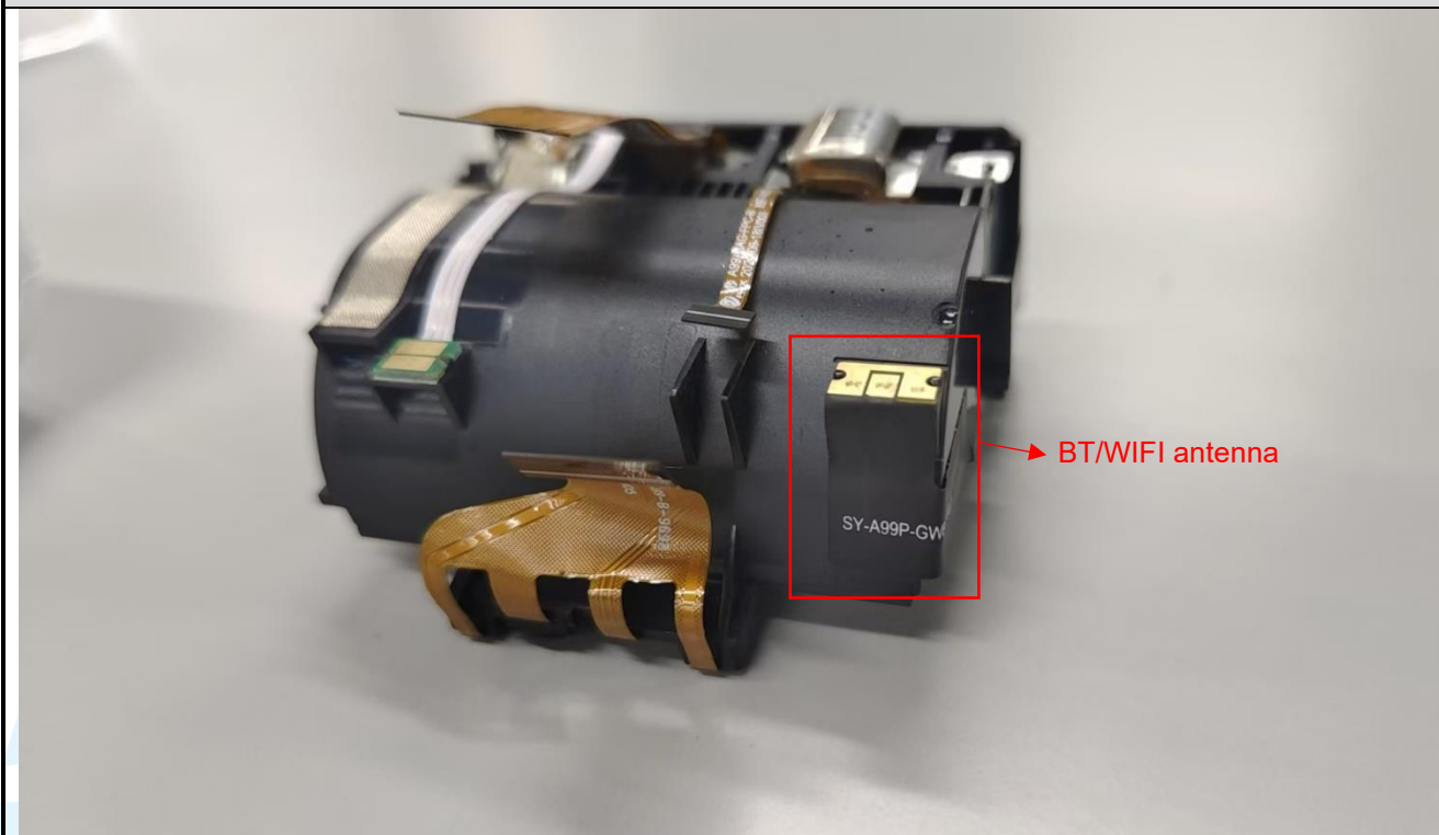
EUT Photo
