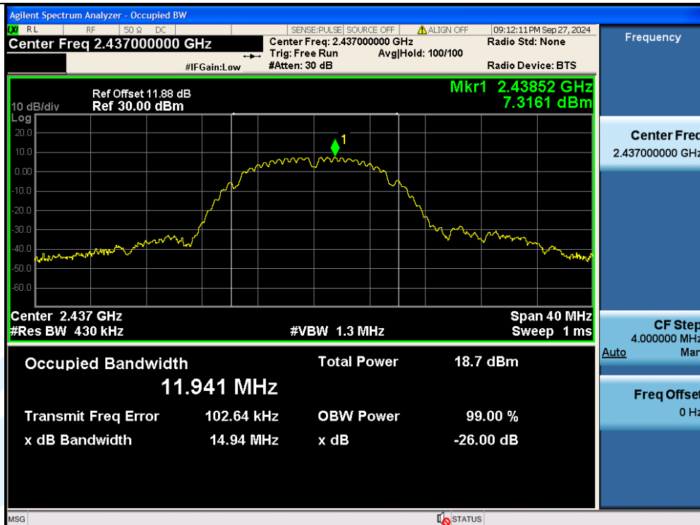
11B-Ant1-2437
