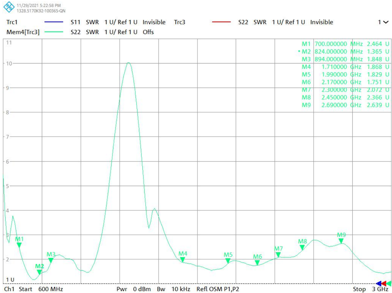
VSWR
