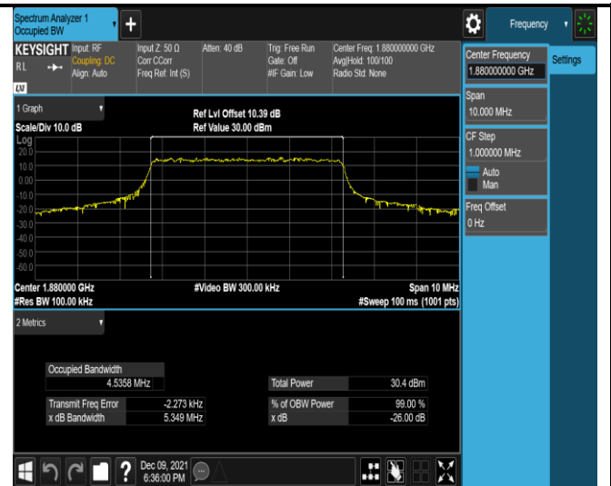
Band2-5MHz-QPSK-18900-25RB#0
