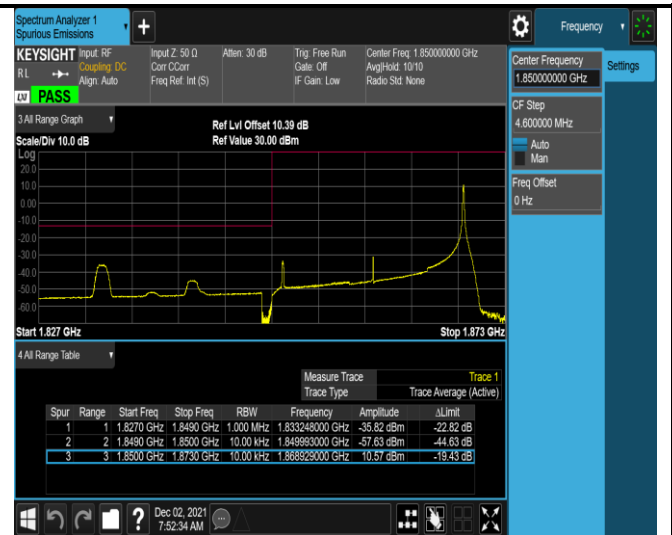
Band2-20MHz-QPSK-18700-1RB#99
