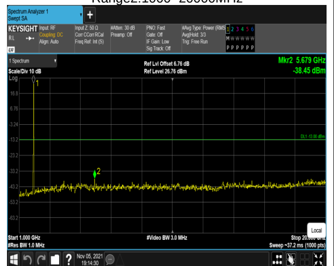
Band2-20MHz-QPSK-19100-1RB#0- Range2:1000~20000MHz
