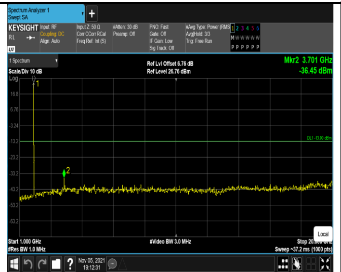
Band2-20MHz-QPSK-18700-1RB#0- Range2:1000~20000MHz
