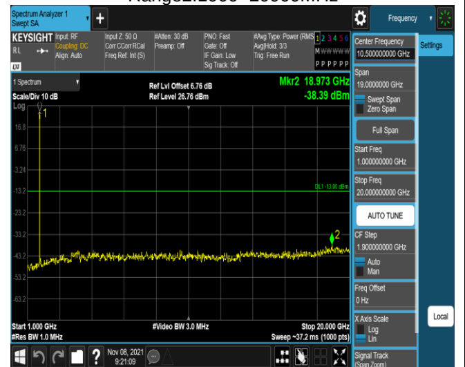
Band4-1.4MHz-QPSK-20175-1RB#0- Range2:1000~20000MHz
