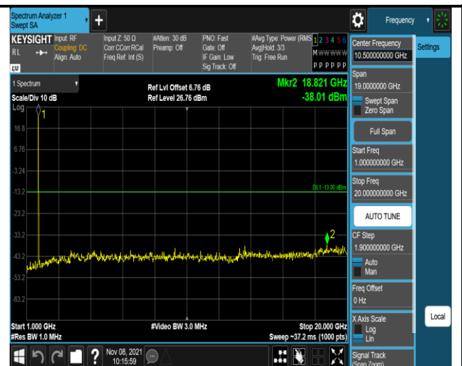
Band4-20MHz-QPSK-20050-1RB#0- Range2:1000~20000MHz
