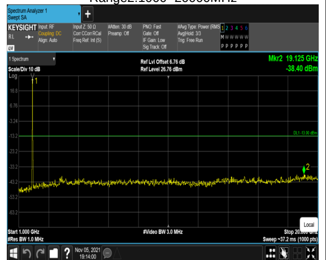
Band2-20MHz-16QAM-18900-1RB#0- Range2:1000~20000MHz
