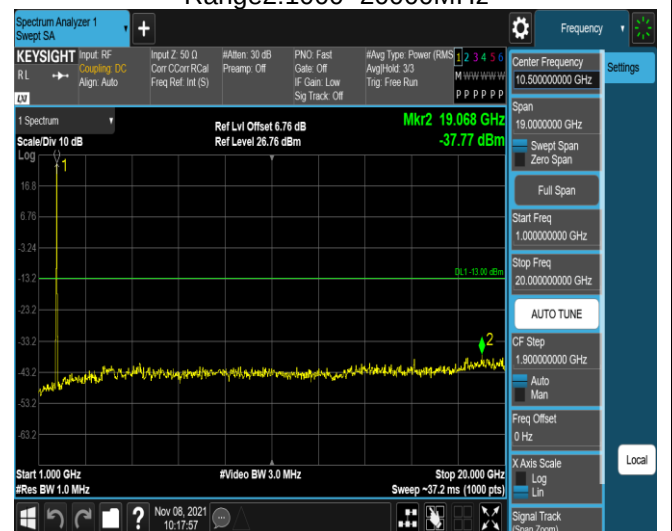
Band4-20MHz-QPSK-20300-1RB#0- Range2:1000~20000MHz
