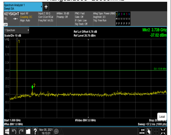
Band2-20MHz-QPSK-18900-1RB#0- Range2:1000~20000MHz
