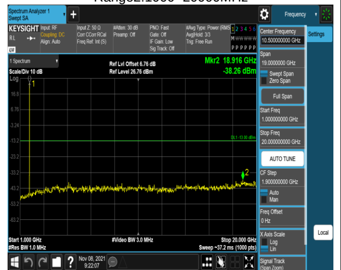
Band4-1.4MHz-QPSK-20393-1RB#0- Range2:1000~20000MHz
