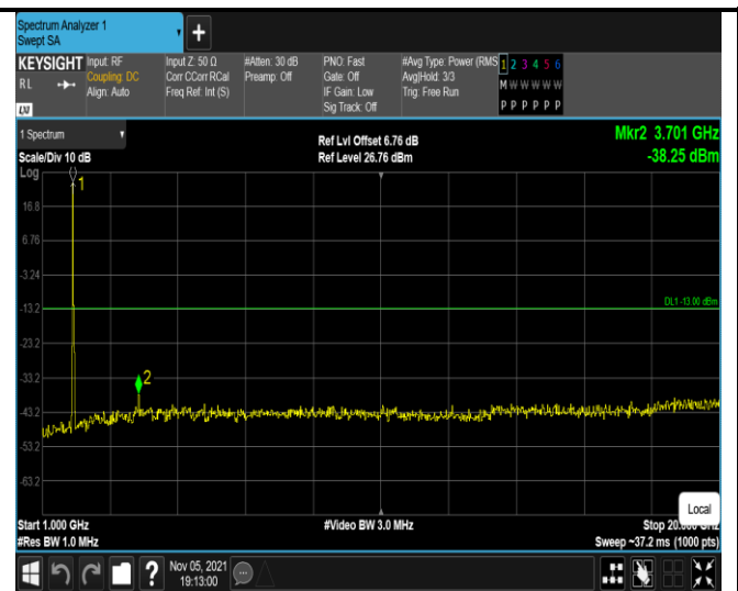
Band2-20MHz-16QAM-18700-1RB#0- Range2:1000~20000MHz
