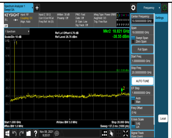
Band4-1.4MHz-QPSK-19957-1RB#0- Range2:1000~20000MHz
