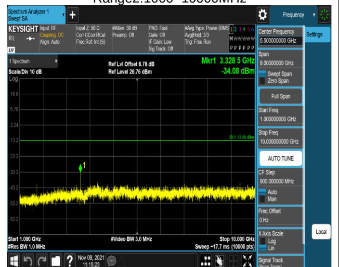
Band5-10MHz-QPSK-20525-1RB#0- Range2:1000~10000MHz
