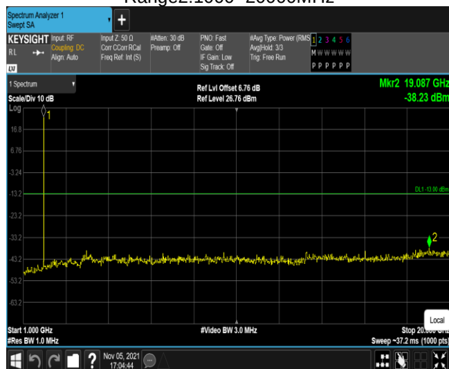
Band2-1.4MHz-QPSK-19193-1RB#0- Range2:1000~20000MHz
