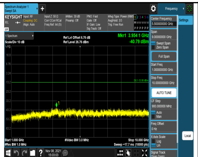
Band13-5MHz-QPSK-23255-1RB#0- Range2:1000~10000MHz
