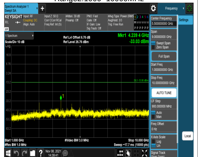
Band12-10MHz-QPSK-23130-1RB#0- Range2:1000~10000MHz
