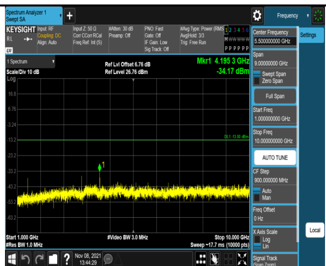
Band12-1.4MHz-QPSK-23017-1RB#0- Range2:1000~10000MHz
