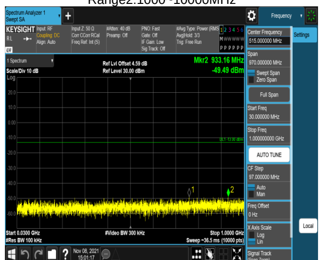
Band13-5MHz-QPSK-23230-1RB#0- Range1:30~1000MHz
