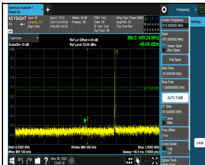
Band12-1.4MHz-QPSK-23017-1RB#0- Range1:30~1000MHz
