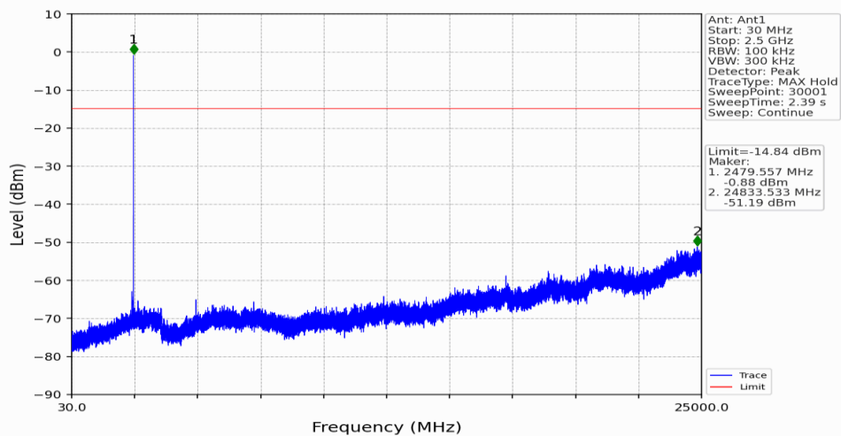
2M_HCH_2480MHz_Ant1_NTNV
