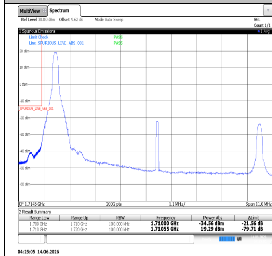
Band4-10MHz-QPSK-20000-50RB#0-PASS
