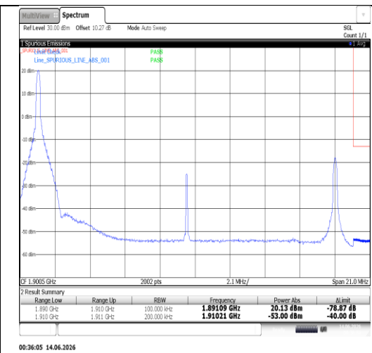
Band2-20MHz-QPSK-19100-100RB#0-PASS
