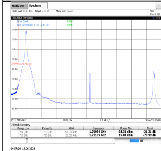
Band4-20MHz-QPSK-20050-100RB#0-PASS
