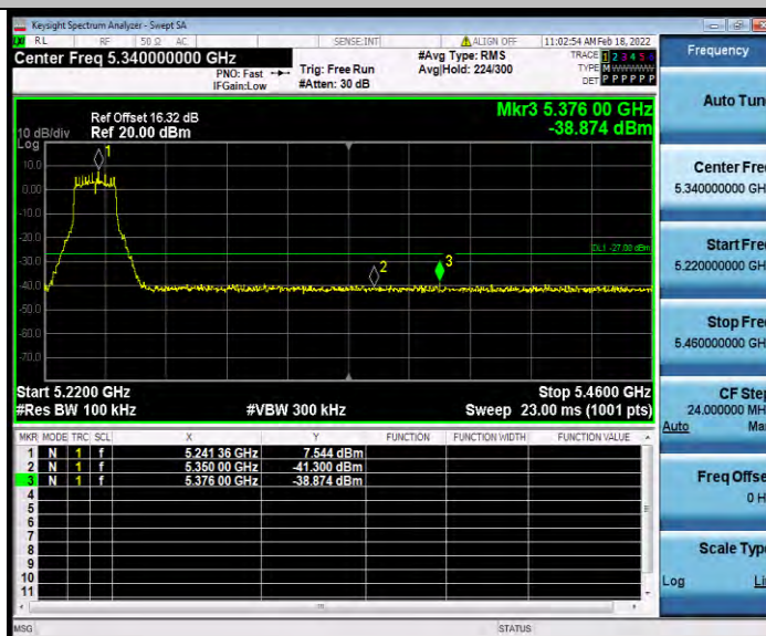
11A_Ant1_Low_5260
