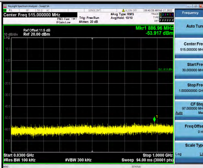
DH5_Ant1_2480_30~1000
