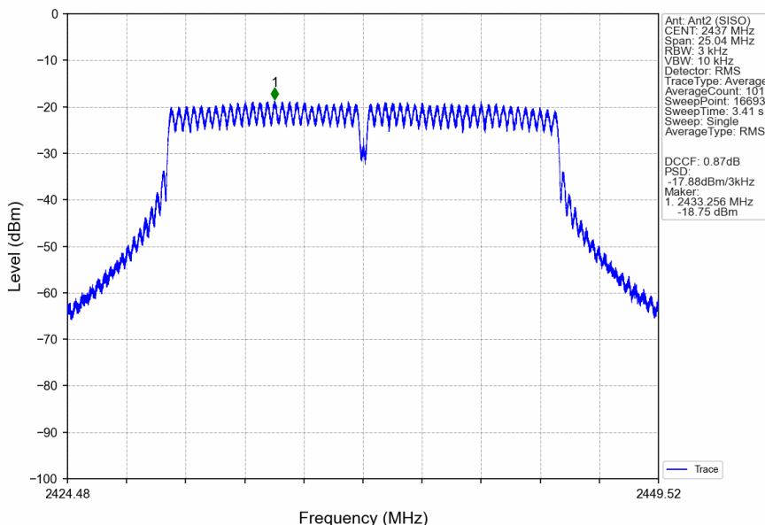
802.11g_MCH_2437MHz_Ant2 (SISO)_NTNV
