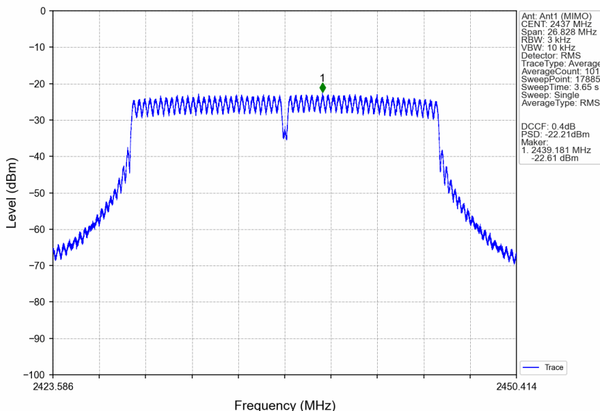
802.11n(HT20)_MCH_2437MHz_Ant1 (MIMO)_NTNV
