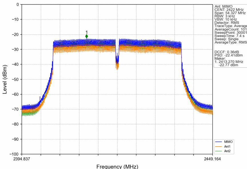
802.11n(HT40)_LCH_2422MHz_MIMO_NTNV
