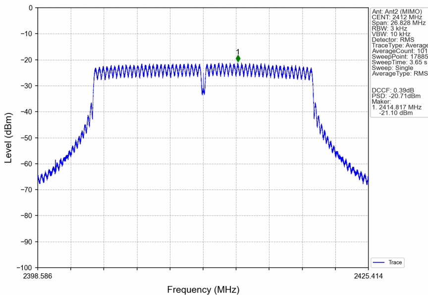
802.11n(HT20)_LCH_2412MHz_Ant2 (MIMO)_NTNV
