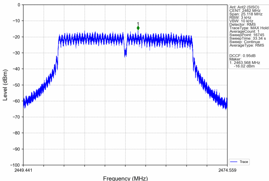
802.11g_HCH_2462MHz_Ant2 (SISO)_NTNV
