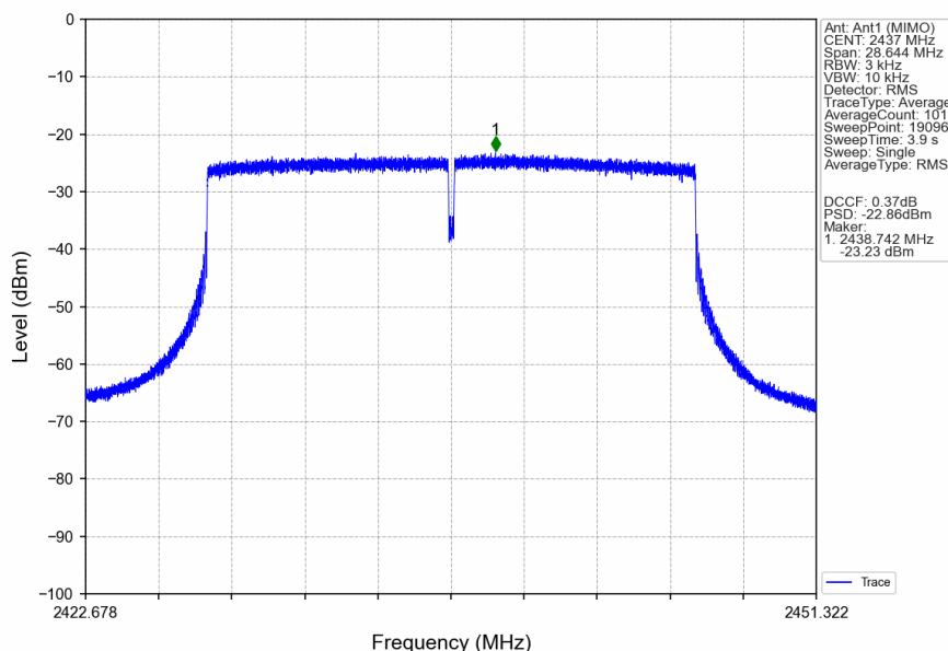
802.11ax(HEW20)_MCH_2437MHz_RU242_Left_Ant1 (MIMO)_NTNV
