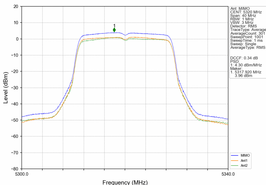
802.11n(HT20)_HCH_5320MHz_MIMO_NTNV
