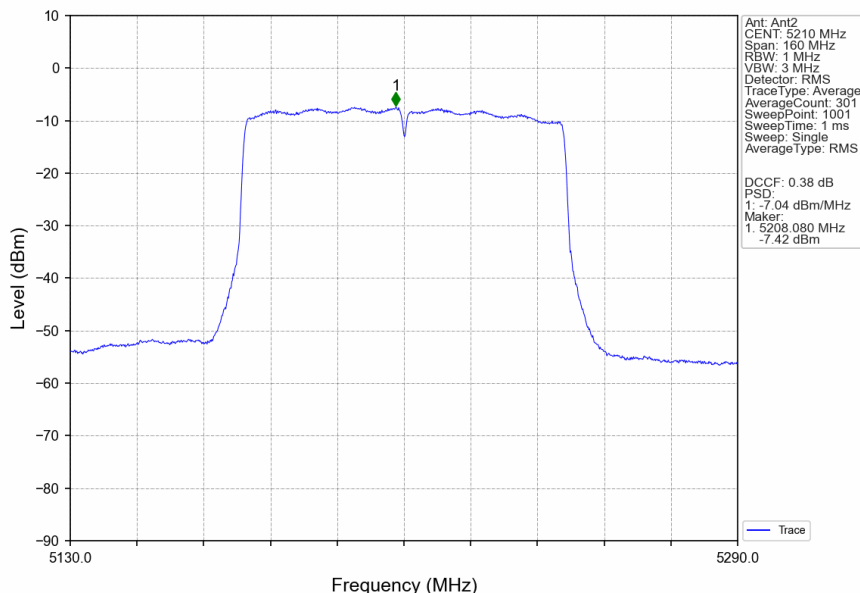
802.11ac(VHT80)_MCH_5210MHz_Ant2_NTNV
