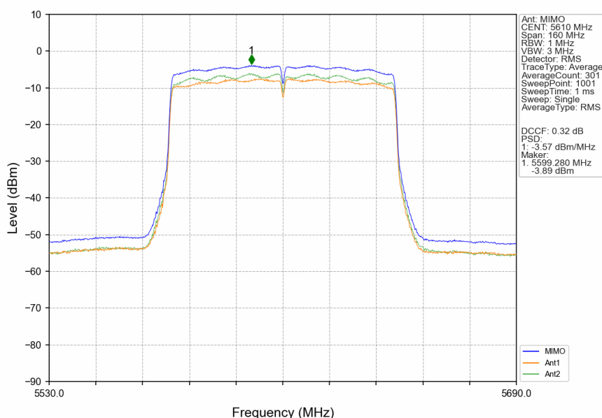
802.11ac(VHT80)_HCH_5610MHz_MIMO_NTNV
