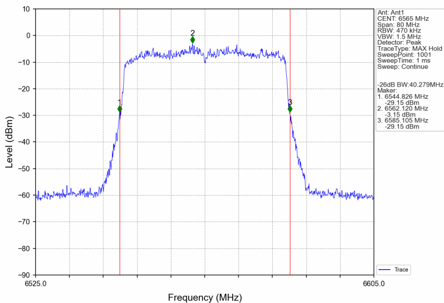
802.11ax(HEW40)_LCH_6565MHz_RU484_Left_Ant1_NTNV
