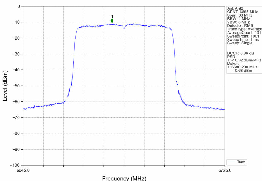
802.11ax(HEW40)_MCH_6685MHz_RU484_Left_Ant2_NTNV
