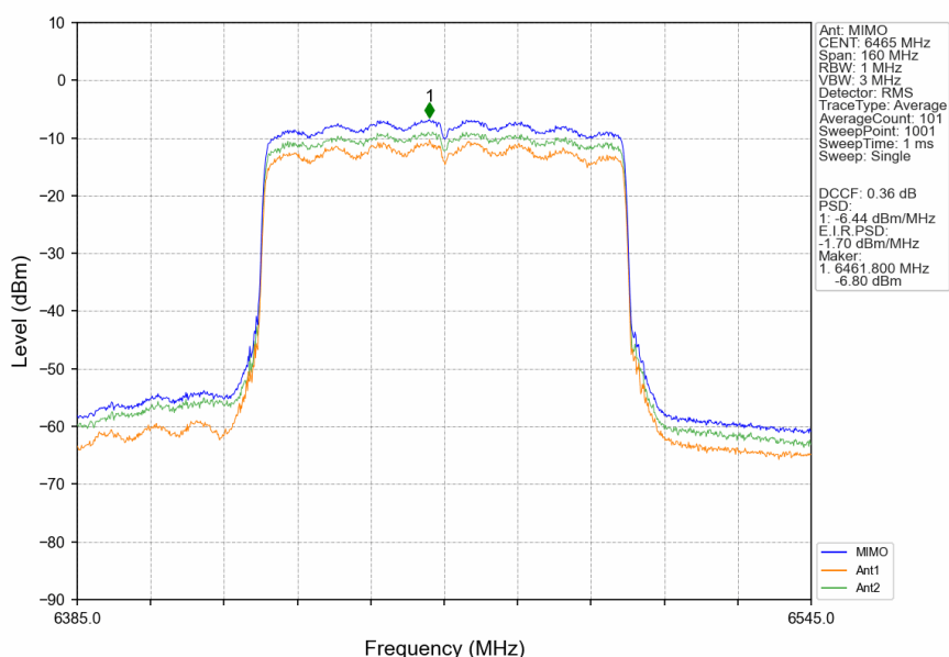
802.11ax(HEW80)_LCH_6465MHz_RU996_Left_MIMO_NTNV
