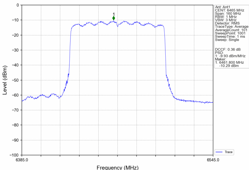
802.11ax(HEW80)_LCH_6465MHz_RU996_Left_Ant1_NTNV
