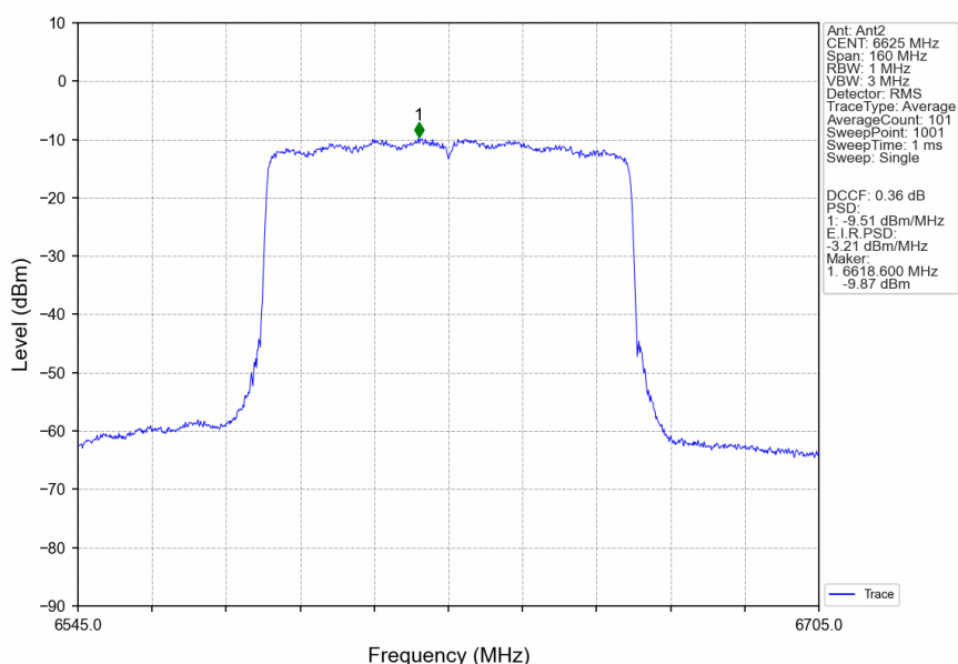
802.11ax(HEW80)_LCH_6625MHz_RU996_Left_Ant2_NTNV
