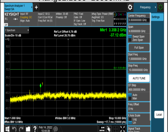
Band12-1.4MHz-QPSK-23017-1RB#0- Range2:1000~10000MHz
