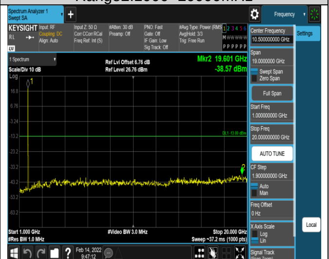
Band4-20MHz-QPSK-20300-1RB#0- Range2:1000~20000MHz
