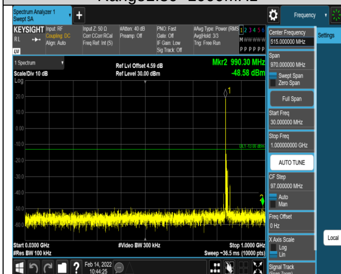
Band12-1.4MHz-QPSK-23017-1RB#0- Range1:30~1000MHz
