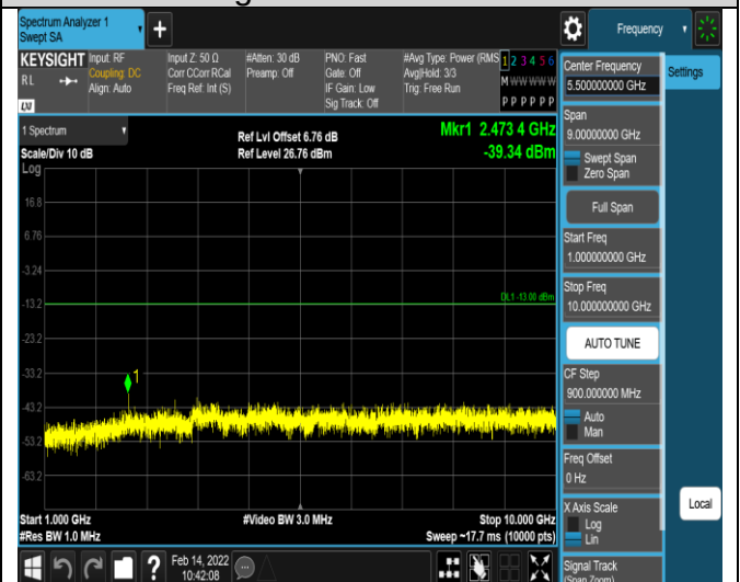
Band5-10MHz-QPSK-20525-1RB#0- Range2:1000~10000MHz
