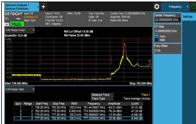
1RB (779.5MHz)
