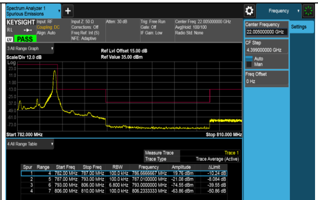
1RB (784.5MHz)
