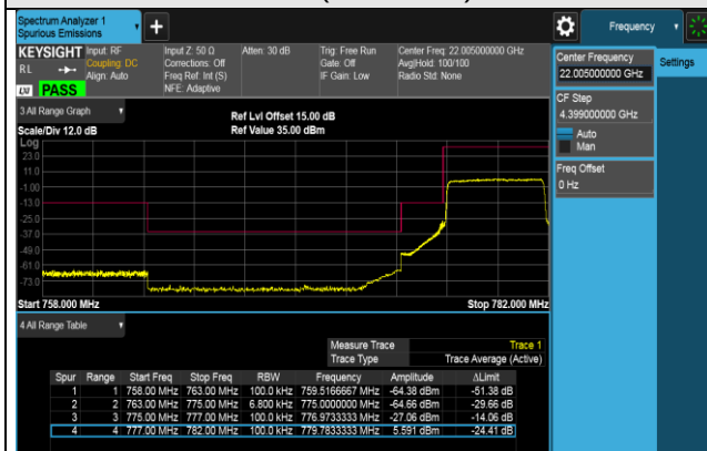
1RB (779.5MHz)
