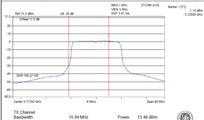
802.11ax (HE20) Full RU / Chain 0 : CH 144 (U-NII-2C)
