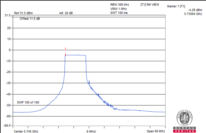
20 MHz Preamble 802.11ax (R106) / Chain 1 : CH 149
