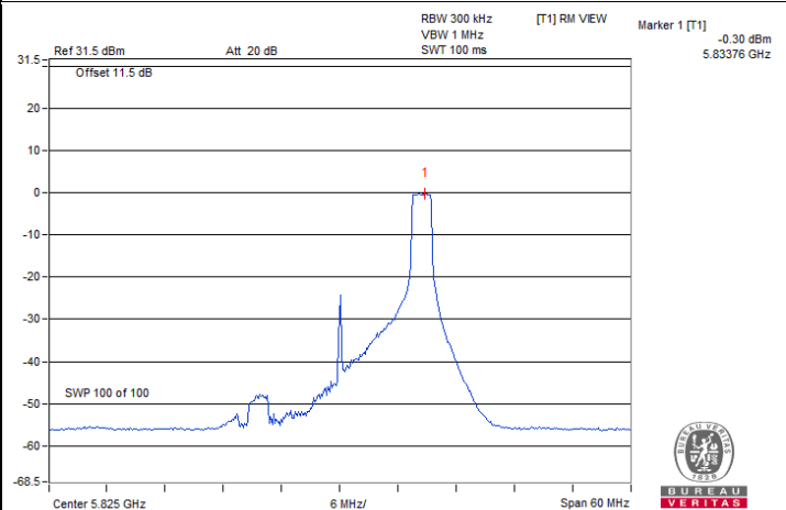
20 MHz Preamble 802.11ax (RU26) / Chain 1 : CH 165
