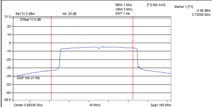
802.11ax (HE80) Full RU / Chain 0 : CH 138 (U-NII-2C)
