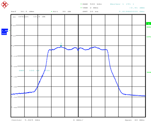
802.11ac20_5825MHz_Chain 0
