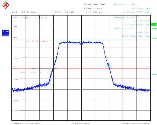
802.11ac20_5180MHz_Chain 0
