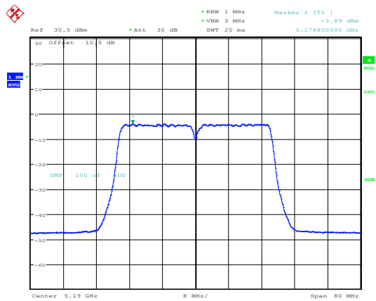
802.11ac40_5190MHz_Chain 1
