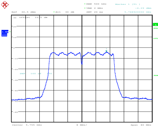
802.11ac40_5755MHz_Chain 0
