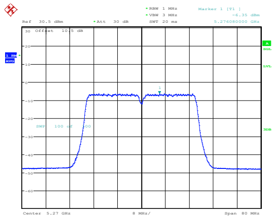
802.11ac40_5270MHz_Chain 1
