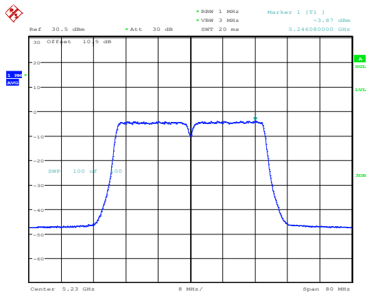
802.11ac40_5230MHz_Chain 1
