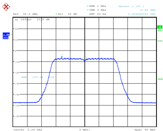
802.11ac20_5260MHz_Chain 1
