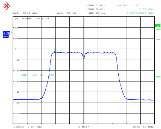
802.11ac40_5270MHz_Chain 0
