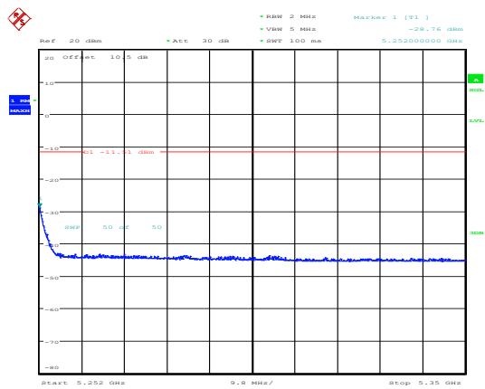
802.11ac80_5210MHz_Chain 0
