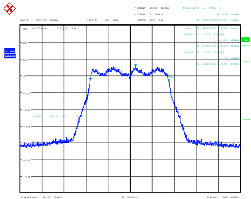
802.11ac20_5200MHz_Chain 0
