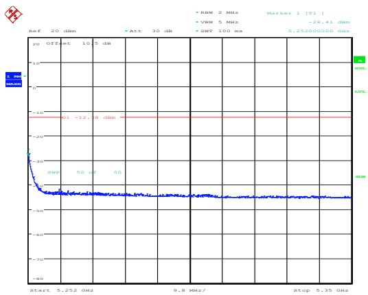
802.11ac80_5210MHz_Chain 1
