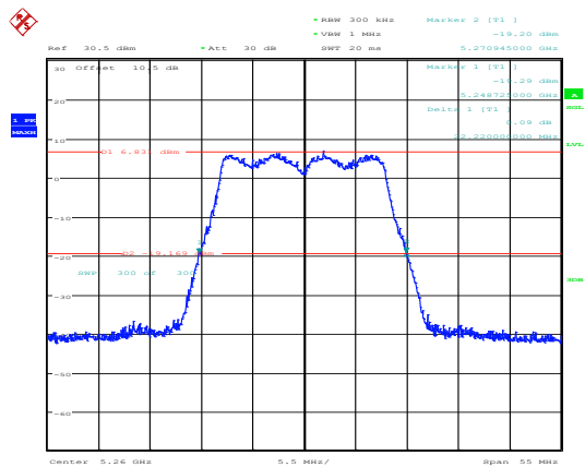
802.11ac20_5260MHz_Chain 0
