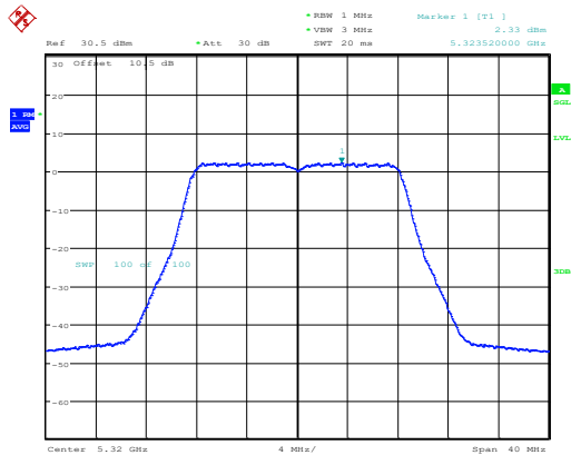
802.11a_5320MHz_Chain 0
