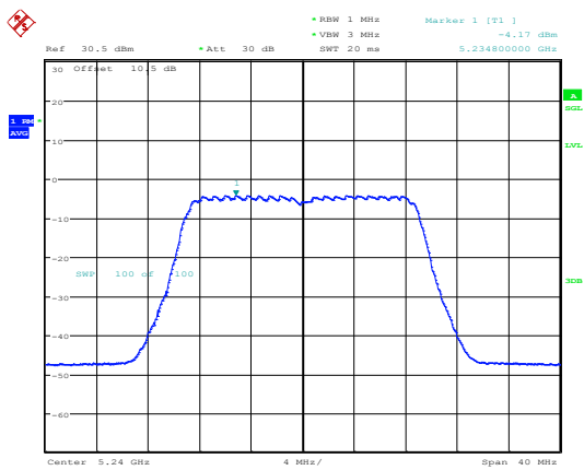
802.11ac20_5240MHz_Chain 1
