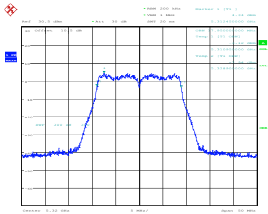
802.11ac20_5320MHz_Chain 0
