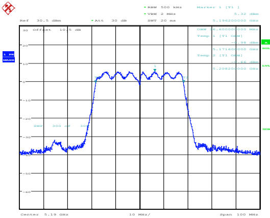
802.11ac40_5190MHz_Chain 0
