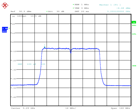
802.11ac80_5290MHz_Chain 1
