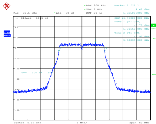
802.11a_5320MHz_Chain 0
