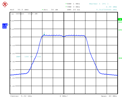
802.11a_5320MHz_Chain 1
