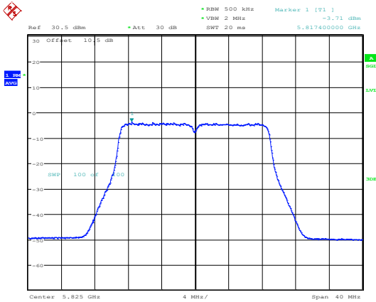
802.11ac20_5825MHz_Chain 1
