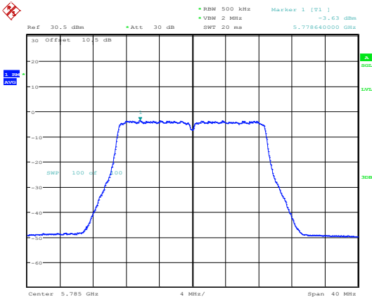
802.11ac20_5785MHz_Chain 1
