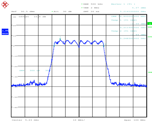
802.11ac40_5230MHz_Chain 0
