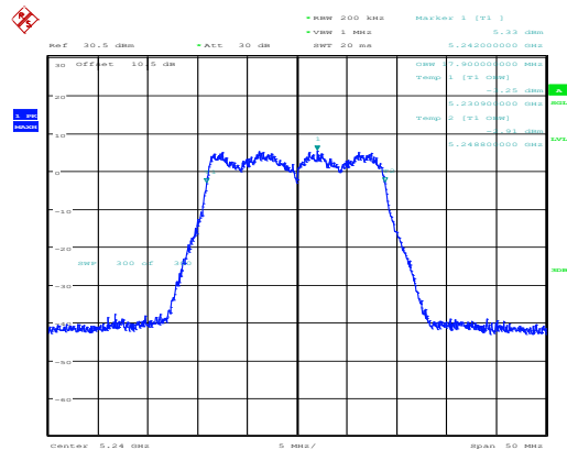
802.11ac20_5240MHz_Chain 0
