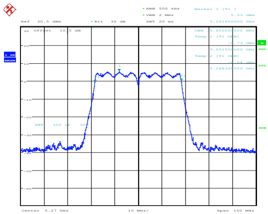
802.11ac40_5270MHz_Chain 0
