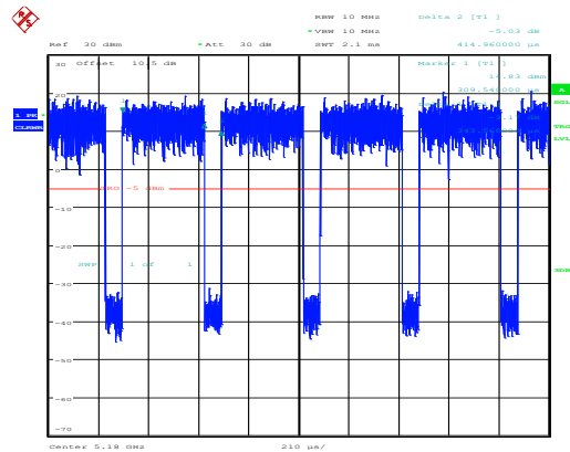
802.11ac20_5180MHz_Chain 0
