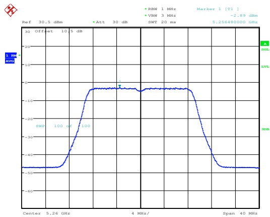
802.11ac20_5260MHz_Chain 0
