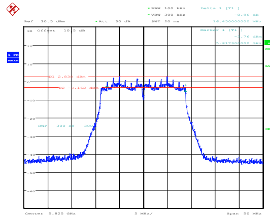
802.11ac20_5825MHz_Chain 0
