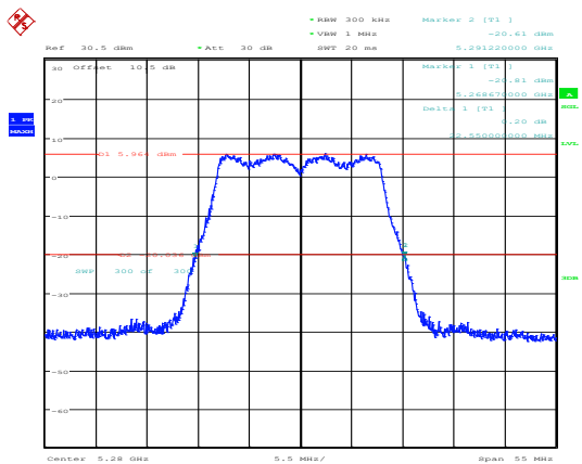
802.11ac20_5280MHz_Chain 0
