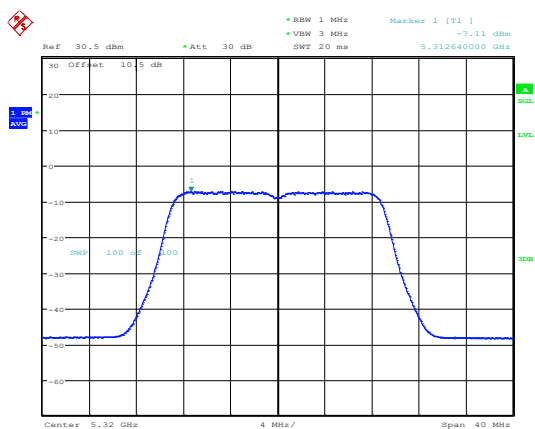
802.11ac20_5320MHz_Chain 1
