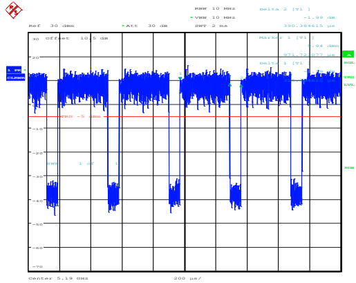
802.11ac40_5190MHz_Chain 0
