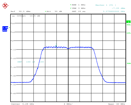
802.11ac20_5280MHz_Chain 1
