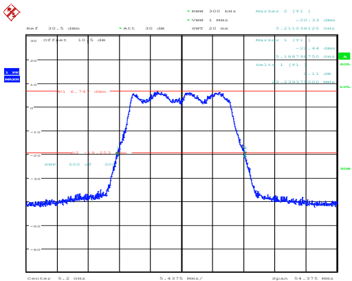
802.11ac20_5200MHz_Chain 0
