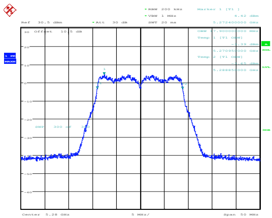
802.11ac20_5280MHz_Chain 0
