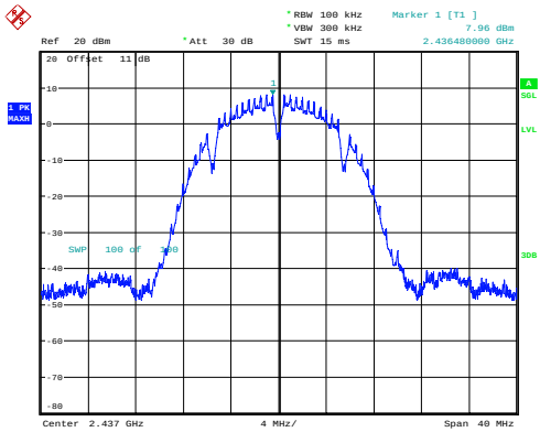
802.11b_2437MHz_Chain 0
