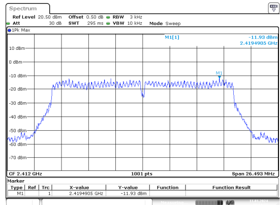
n20_2412MHz_Chain 1
