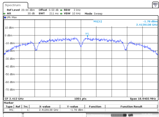
b_2412MHz_Chain 1
