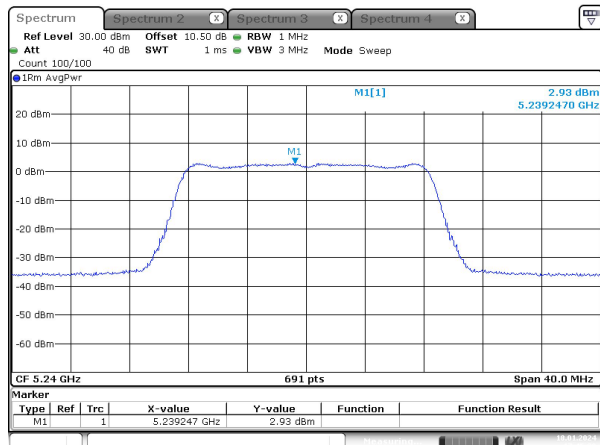
a_ 5240MHz_Chain 0
