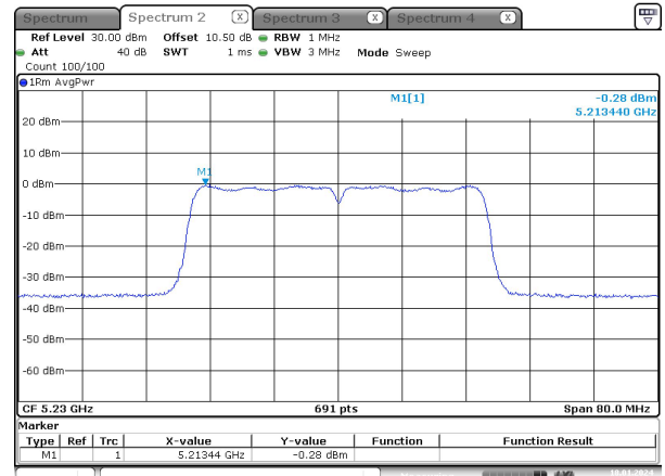
n40_5230MHz_Chain 0
