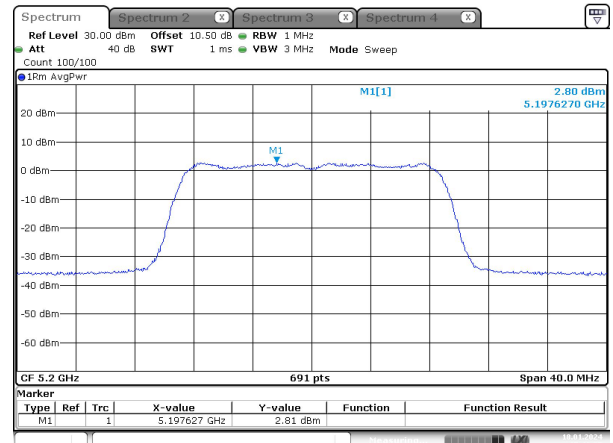
ac20_5200MHz_Chain 0
