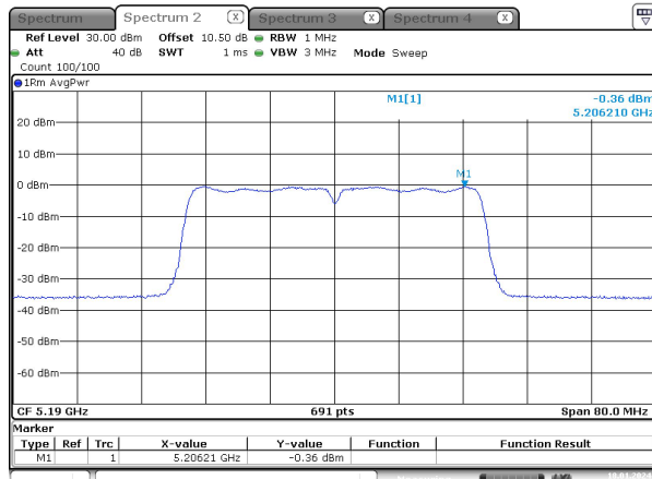
n40_5190MHz_Chain 0
