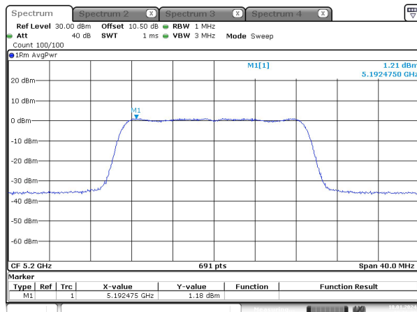
n20_ 5200MHz_Chain 1
