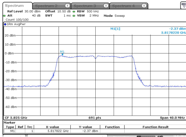
a_ 5825MHz_Chain 0
