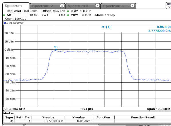
n20_ 5785MHz_Chain 0
