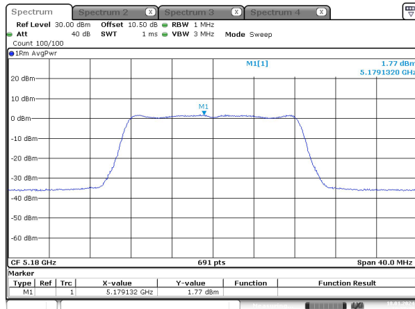
a_ 5180 MHz_Chain 1
