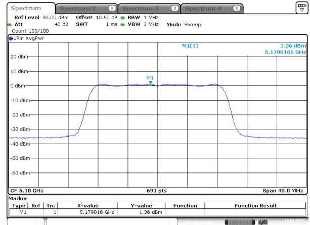
n20_ 5180MHz_Chain 1
