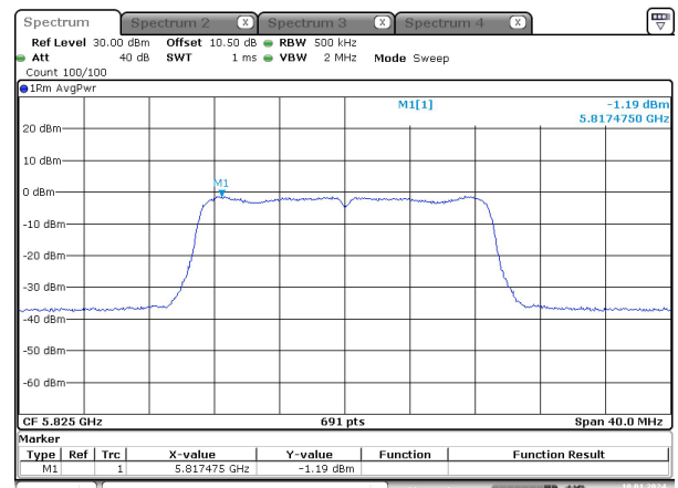
n20_ 5825MHz_Chain 0
