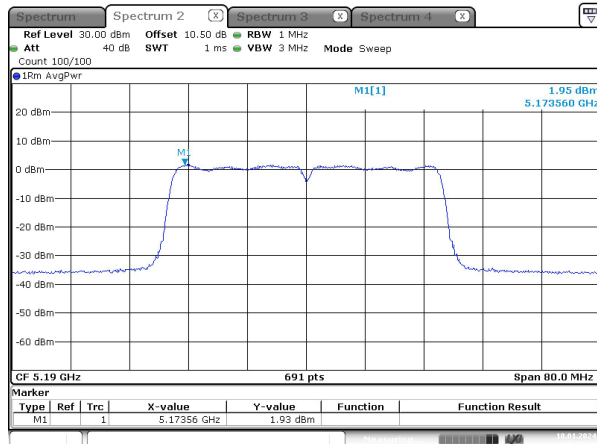
n40_5190MHz_Chain 1
