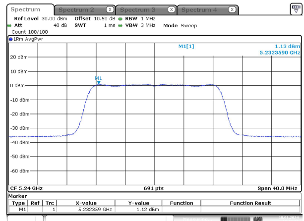
n20_ 5240MHz_Chain 1
