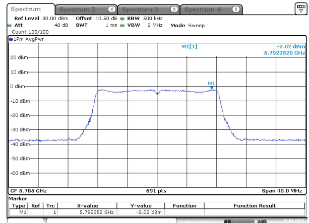
a_ 5785MHz_Chain 0
