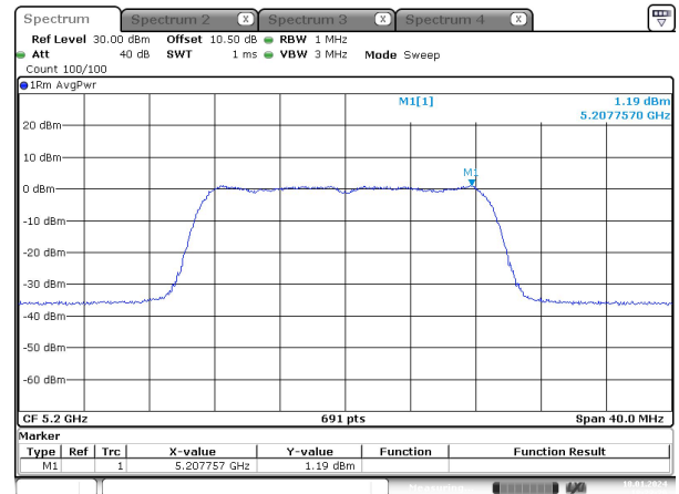
ac20_5200MHz_Chain 1
