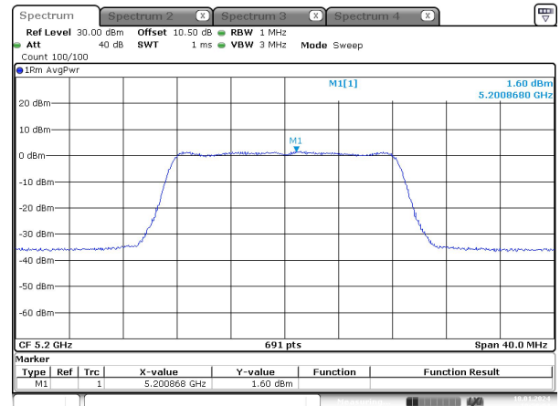
a_ 5200MHz_Chain 1
