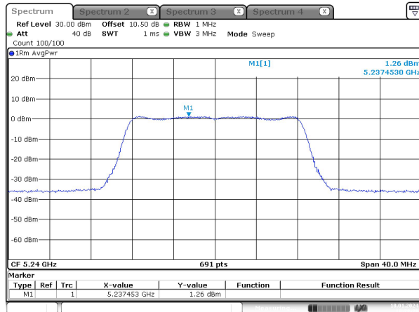
a_ 5240MHz_Chain 1
