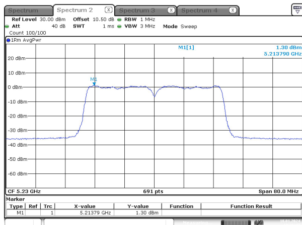
ac40_5230MHz_Chain 1
