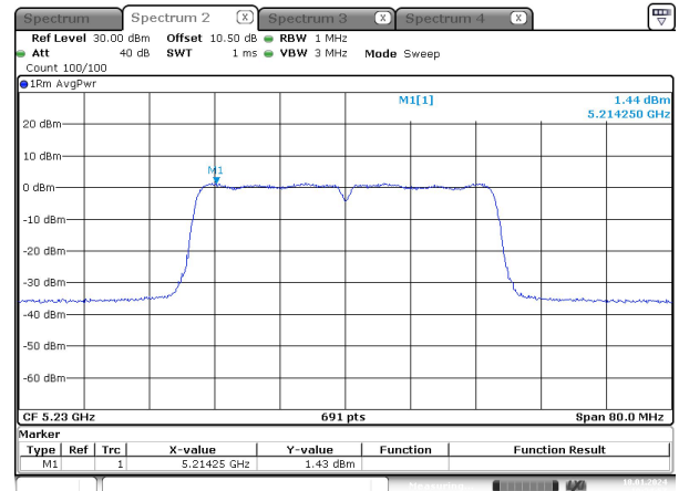
n40_5230MHz_Chain 1
