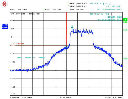
802.11n20_2412MHz_Chain 0
