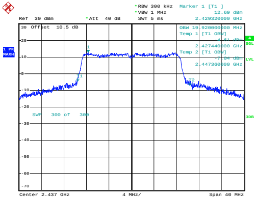
802.11n20_2437MHz_Chain 0
