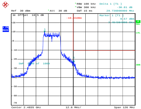
802.11n20_2462MHz_Chain 1
