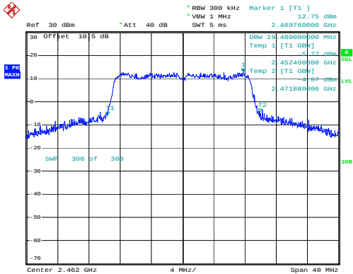
802.11n20_2462MHz_Chain 0
