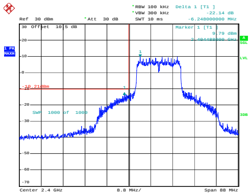
802.11n20_2412MHz_Chain 1
