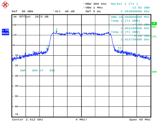
802.11n20_2412MHz_Chain 0
