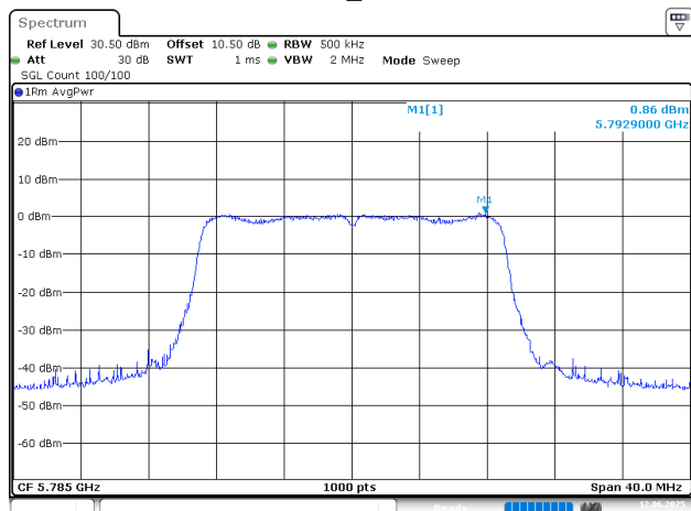
802.11n20_5785MHz
