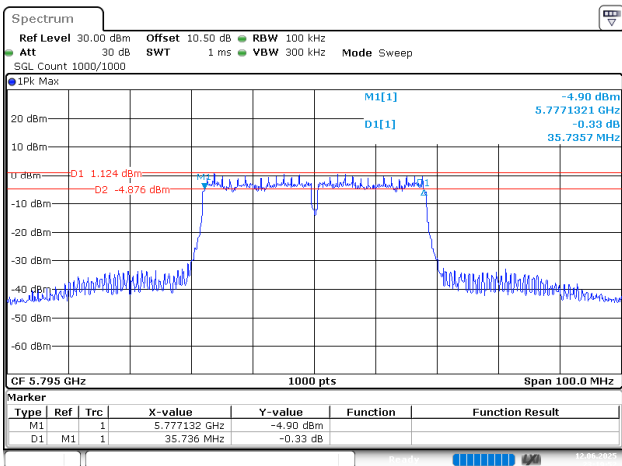
802.11n40_5795MHz
