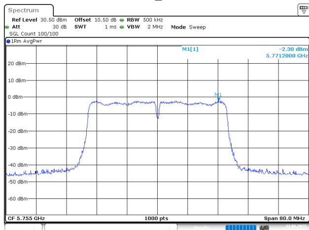
802.11n40_5755MHz
