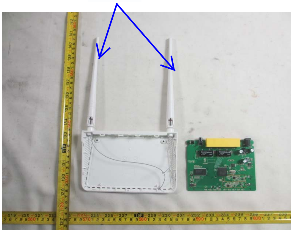
Antenna
