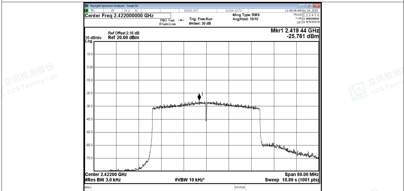
PSD NVNT ax40 2422MHz Ant4
