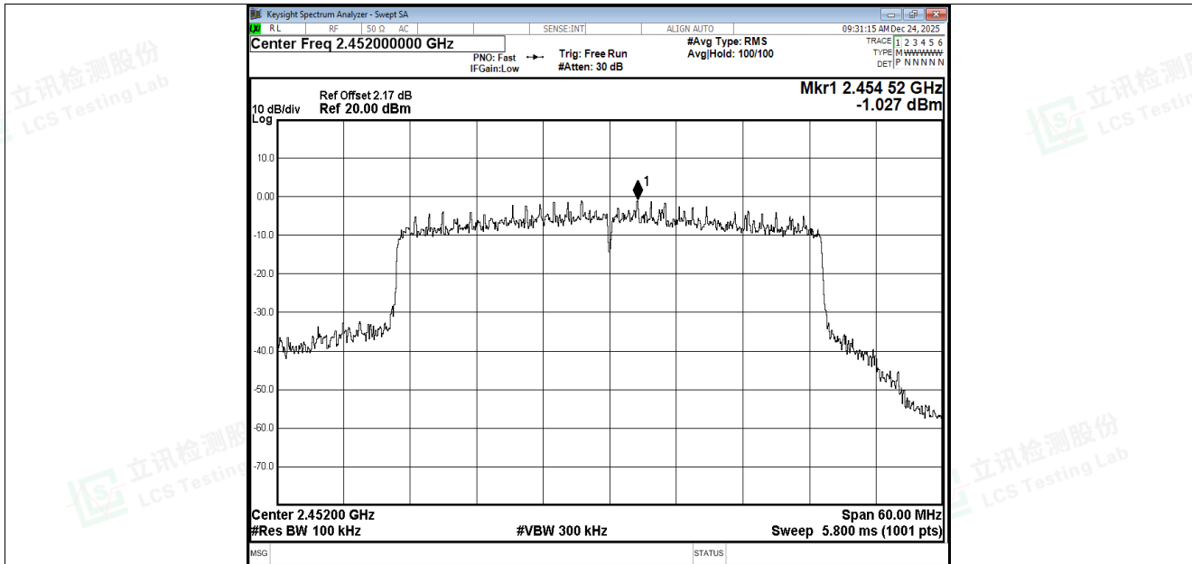
Band Edge NVNT ax40 2452MHz Ant2 Ref
