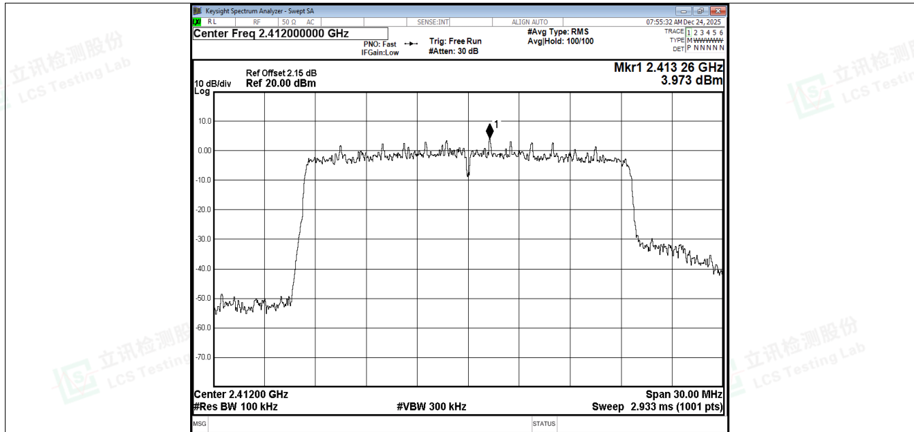
Band Edge NVNT ax20 2412MHz Ant1 Ref
