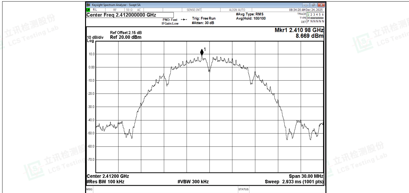
Band Edge NVNT b 2412MHz Ant2 Ref
