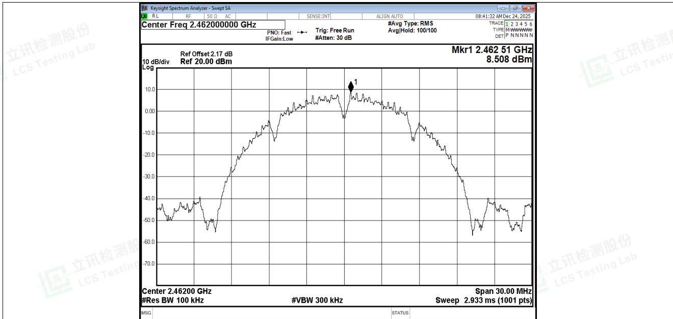
Band Edge NVNT b 2462MHz Ant2 Ref
