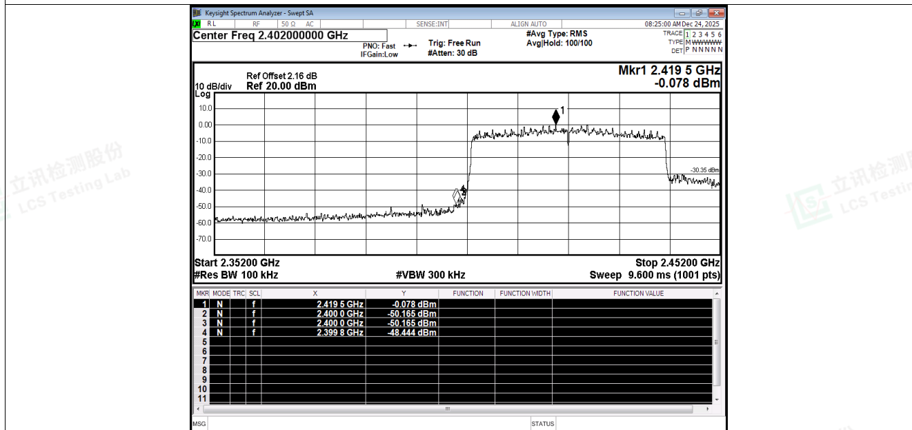
Band Edge NVNT be40 2422MHz Ant1 Emission
