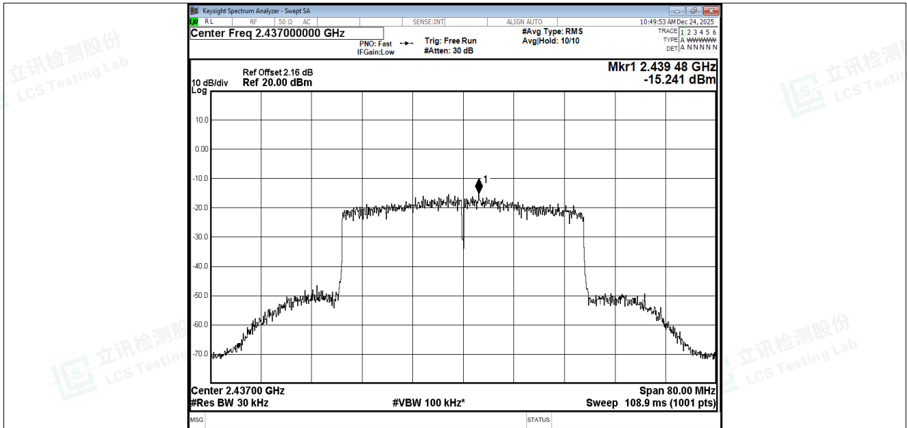
PSD NVNT be40 2437MHz Ant3
