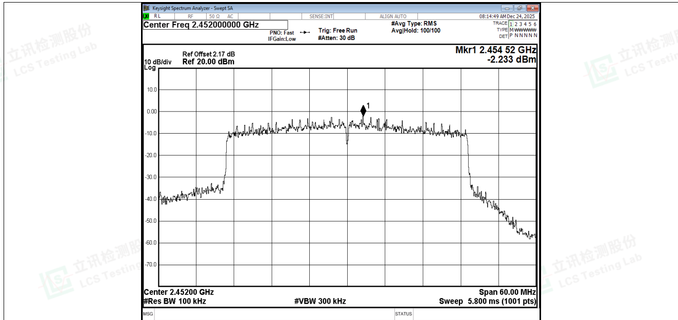
Band Edge NVNT ax40 2452MHz Ant1 Ref
