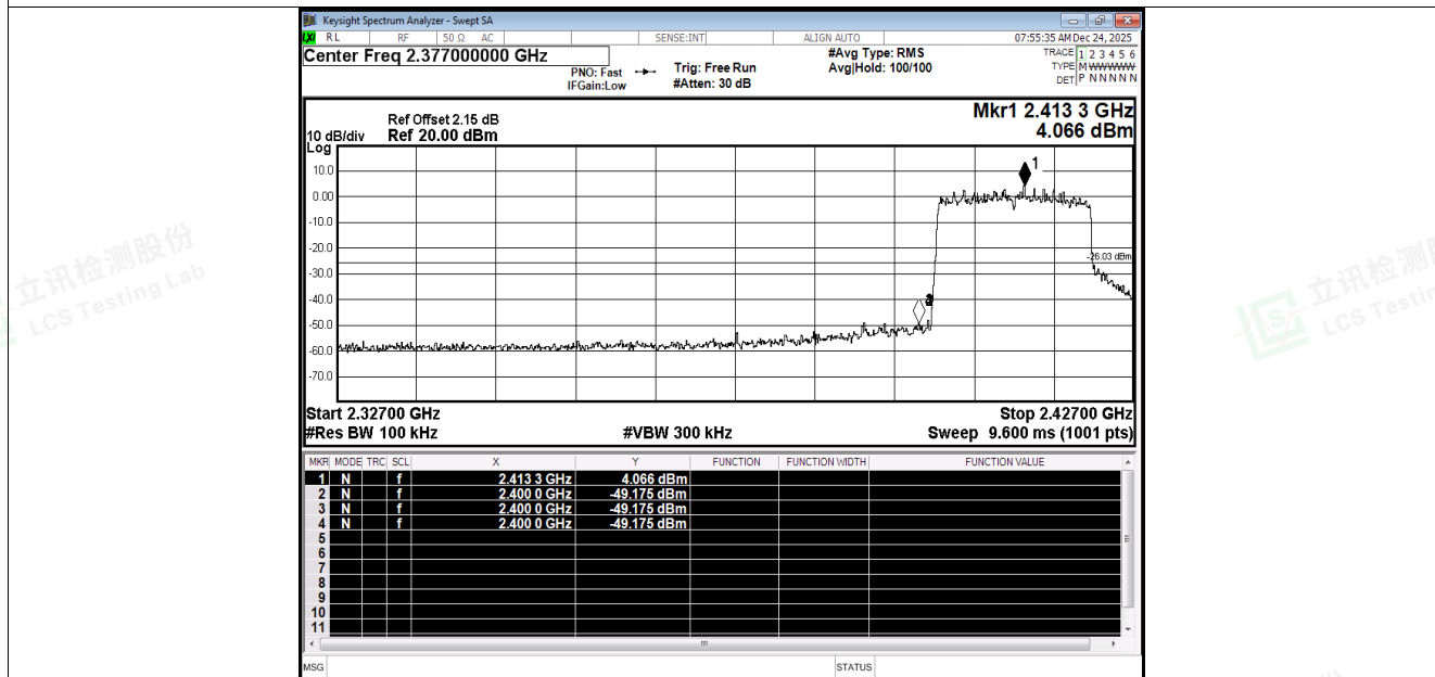
Band Edge NVNT ax20 2412MHz Ant1 Emission
