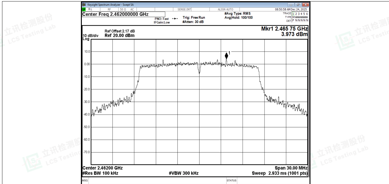
Band Edge NVNT g 2462MHz Ant2 Ref
