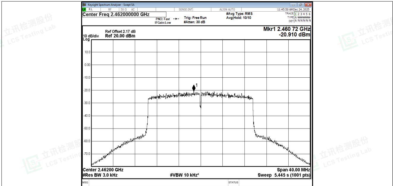
PSD NVNT ax20 2462MHz Ant4
