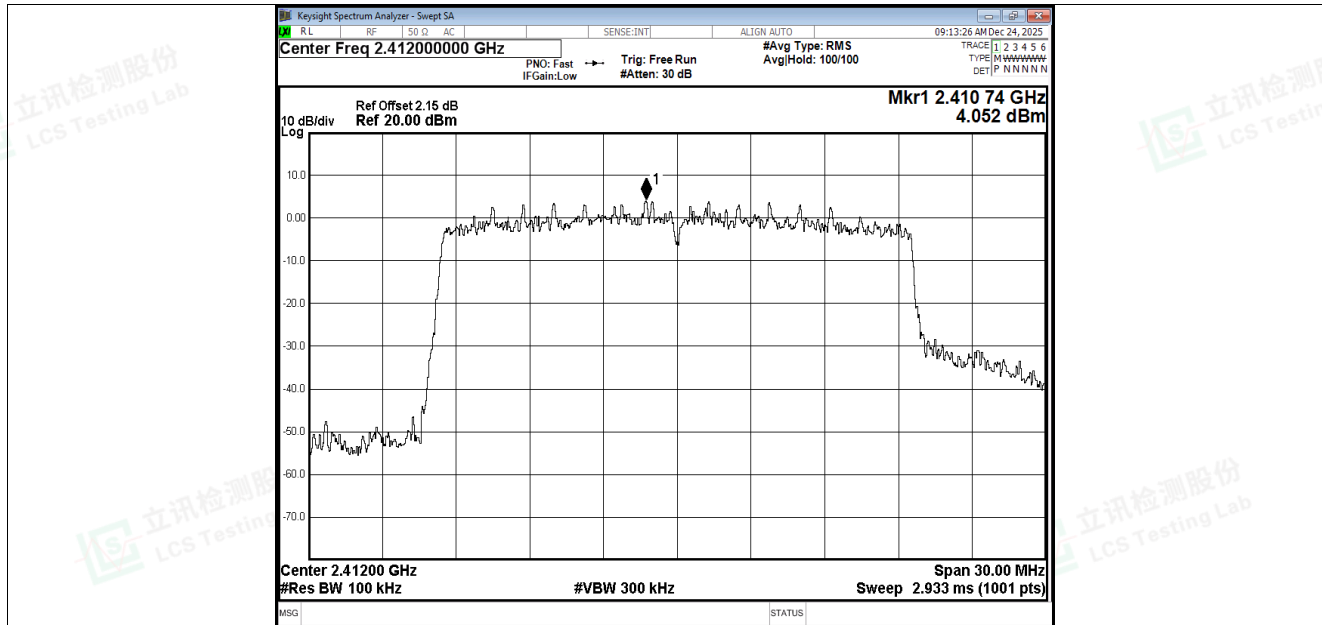
Band Edge NVNT ax20 2412MHz Ant2 Ref
