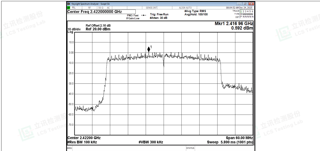
Band Edge NVNT ax40 2422MHz Ant1 Ref
