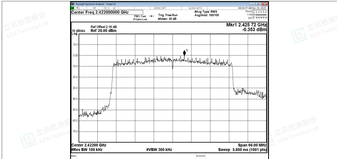
Band Edge NVNT be40 2422MHz Ant1 Ref
