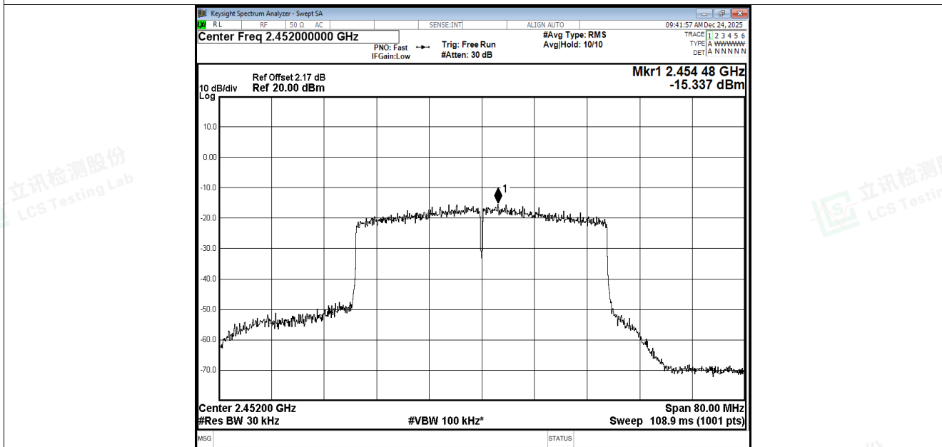
PSD NVNT be40 2452MHz Ant2
