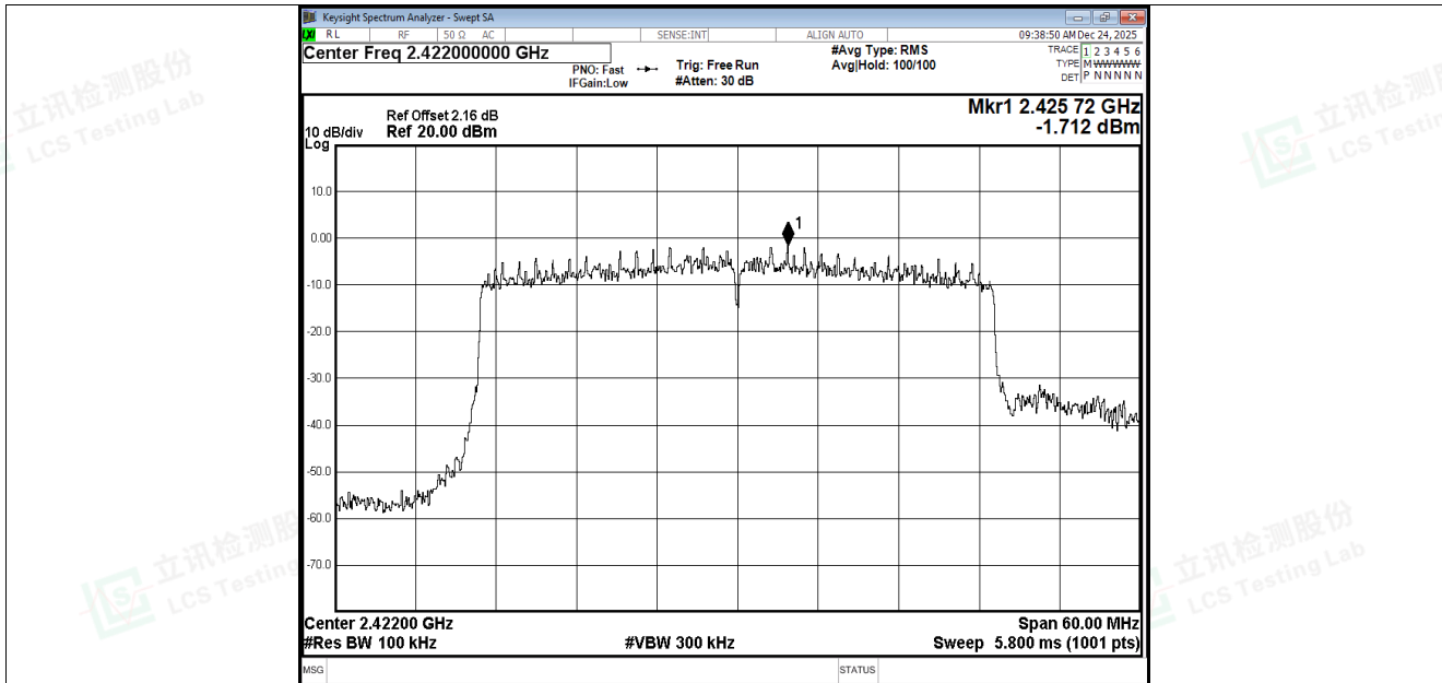
Band Edge NVNT be40 2422MHz Ant2 Ref
