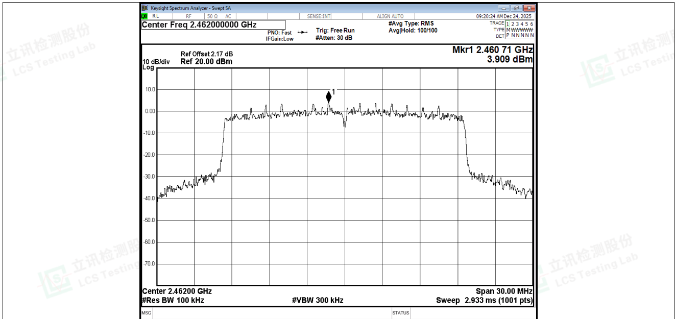
Band Edge NVNT ax20 2462MHz Ant2 Ref
