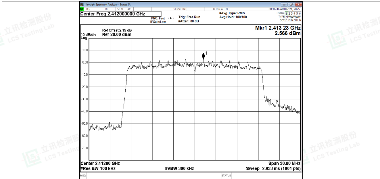
Band Edge NVNT be20 2412MHz Ant1 Ref
