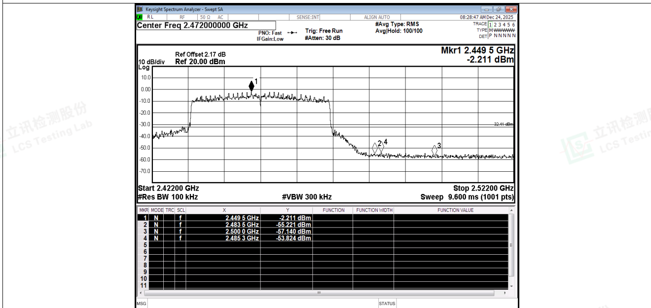
Band Edge NVNT be40 2452MHz Ant1 Emission
