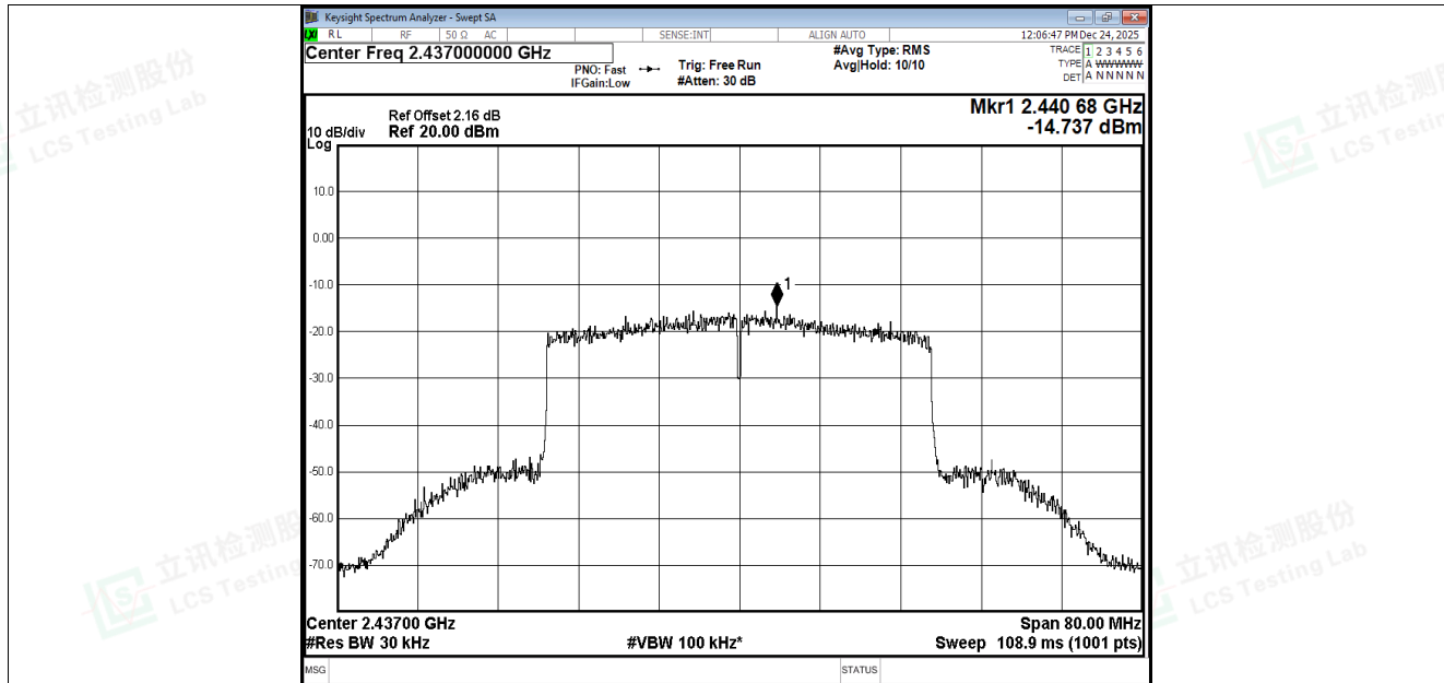
PSD NVNT be40 2437MHz Ant4
