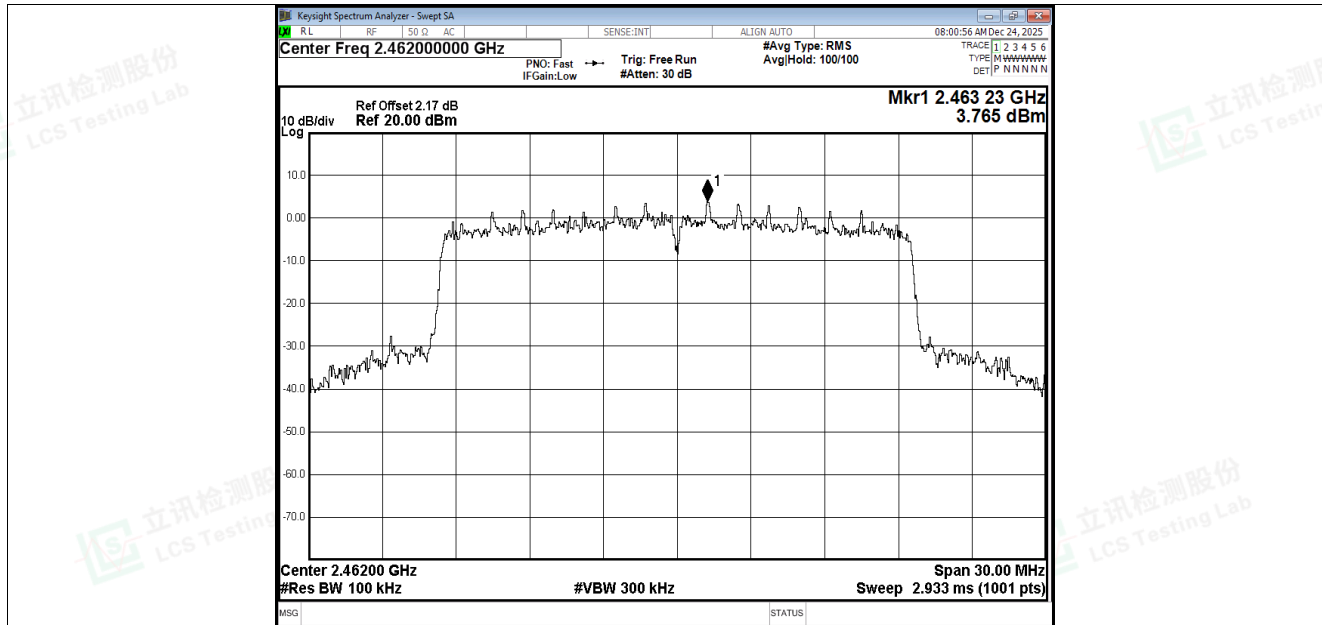
Band Edge NVNT ax20 2462MHz Ant1 Ref
