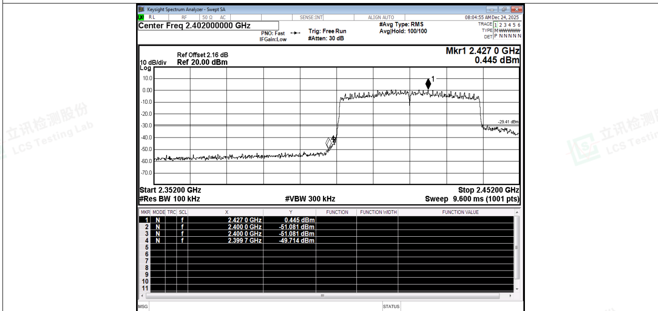
Band Edge NVNT ax40 2422MHz Ant1 Emission
