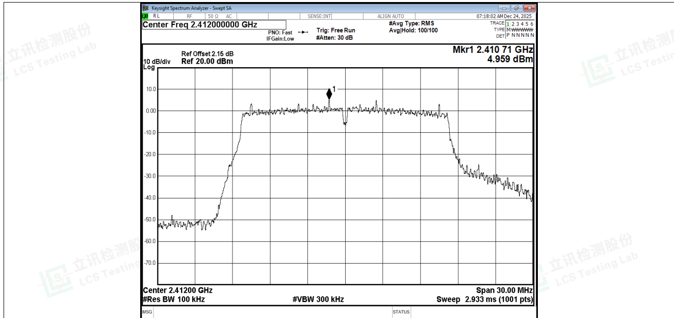
Band Edge NVNT g 2412MHz Ant1 Ref
