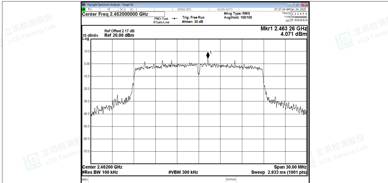
Band Edge NVNT n20 2462MHz Ant1 Ref
