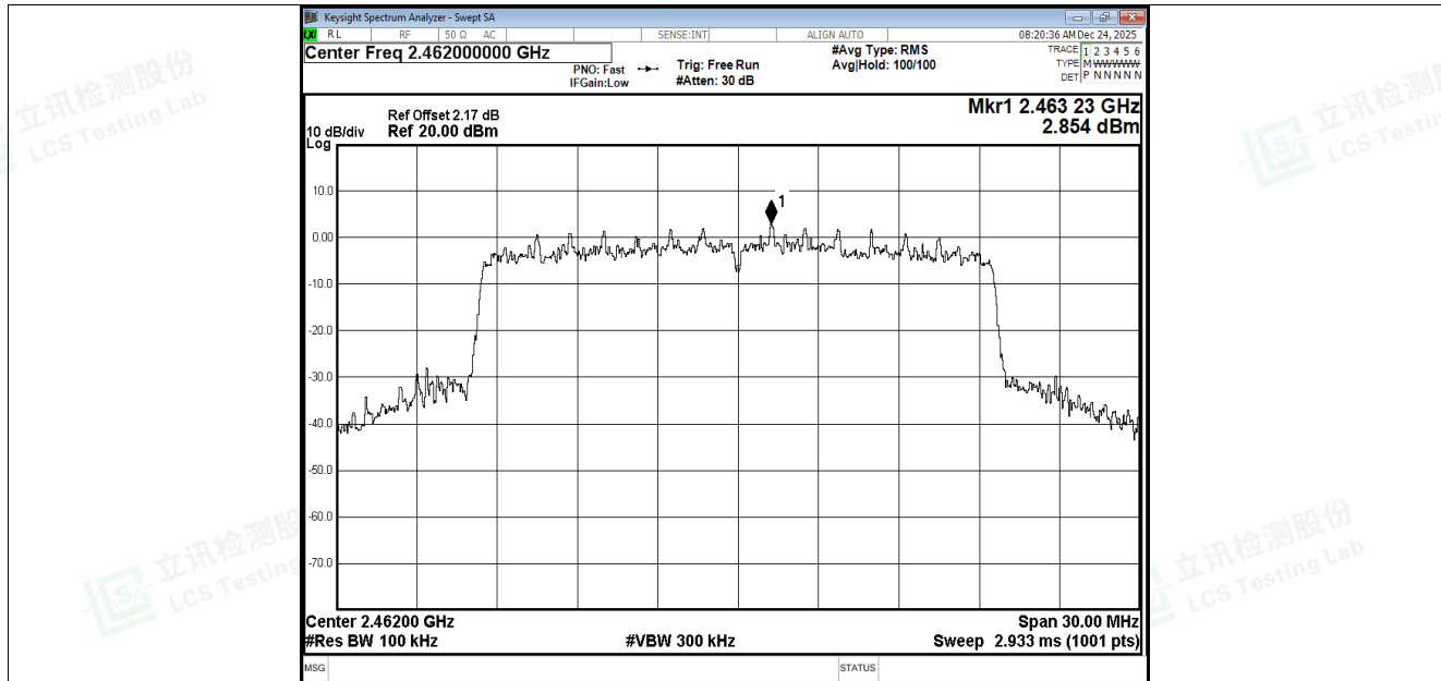
Band Edge NVNT be20 2462MHz Ant1 Ref
