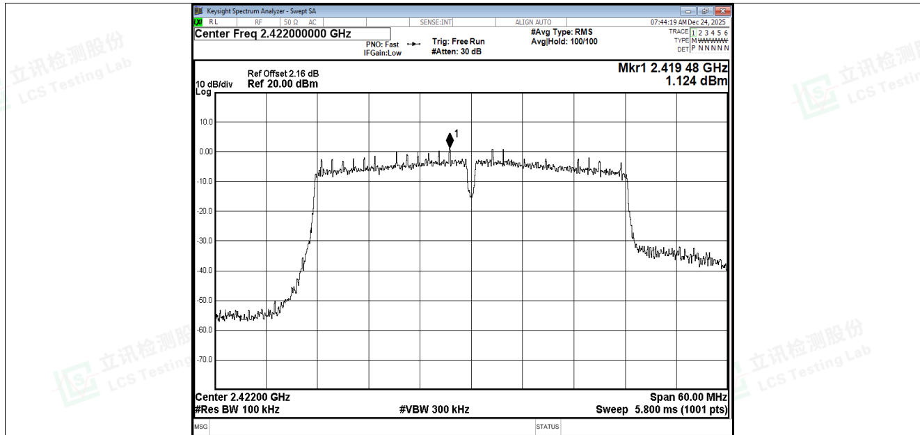
Band Edge NVNT n40 2422MHz Ant1 Ref
