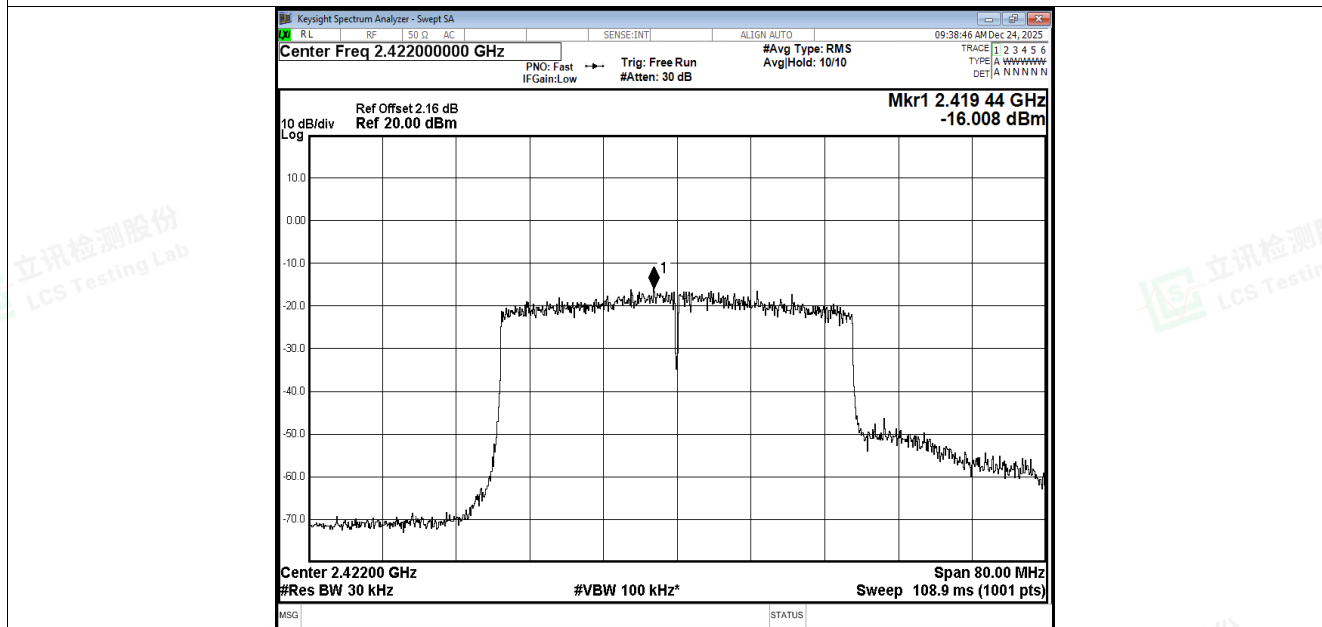
PSD NVNT be40 2422MHz Ant2
