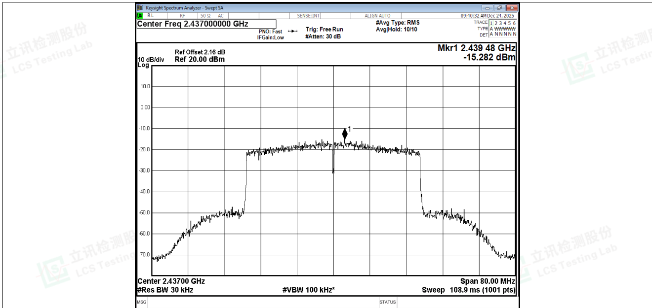
PSD NVNT be40 2437MHz Ant2
