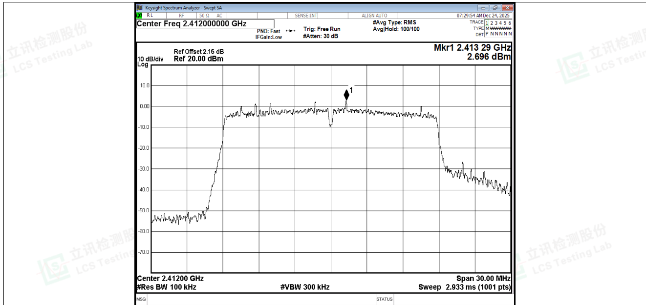
Band Edge NVNT n20 2412MHz Ant1 Ref
