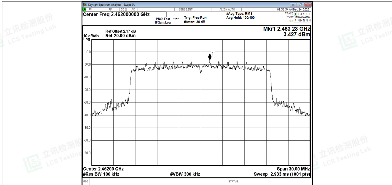
Band Edge NVNT be20 2462MHz Ant2 Ref
