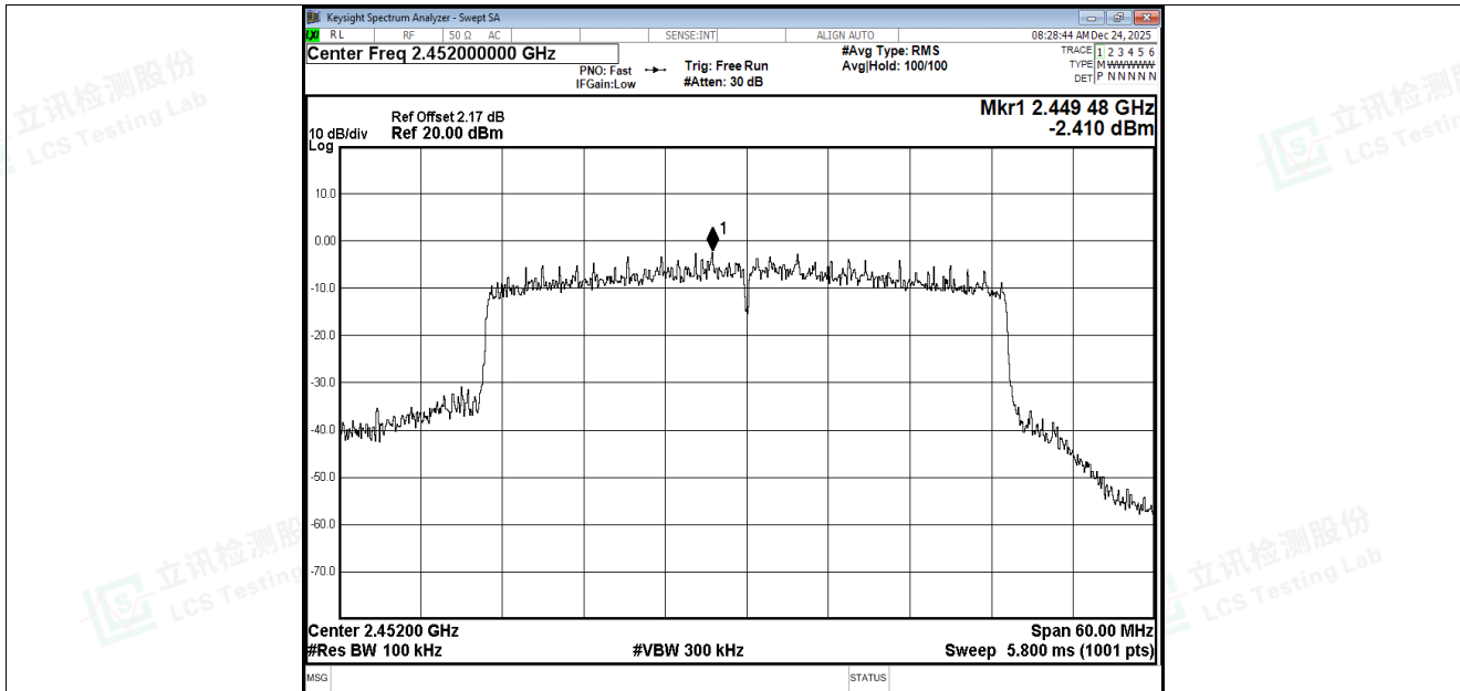
Band Edge NVNT be40 2452MHz Ant1 Ref
