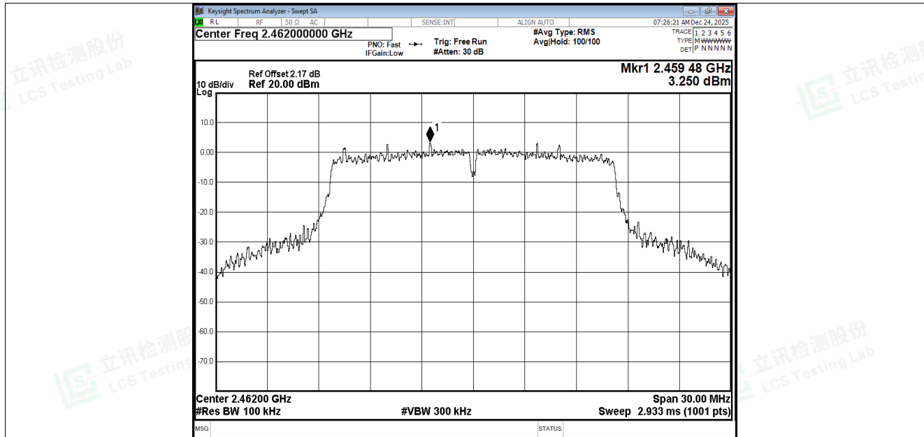
Band Edge NVNT g 2462MHz Ant1 Ref
