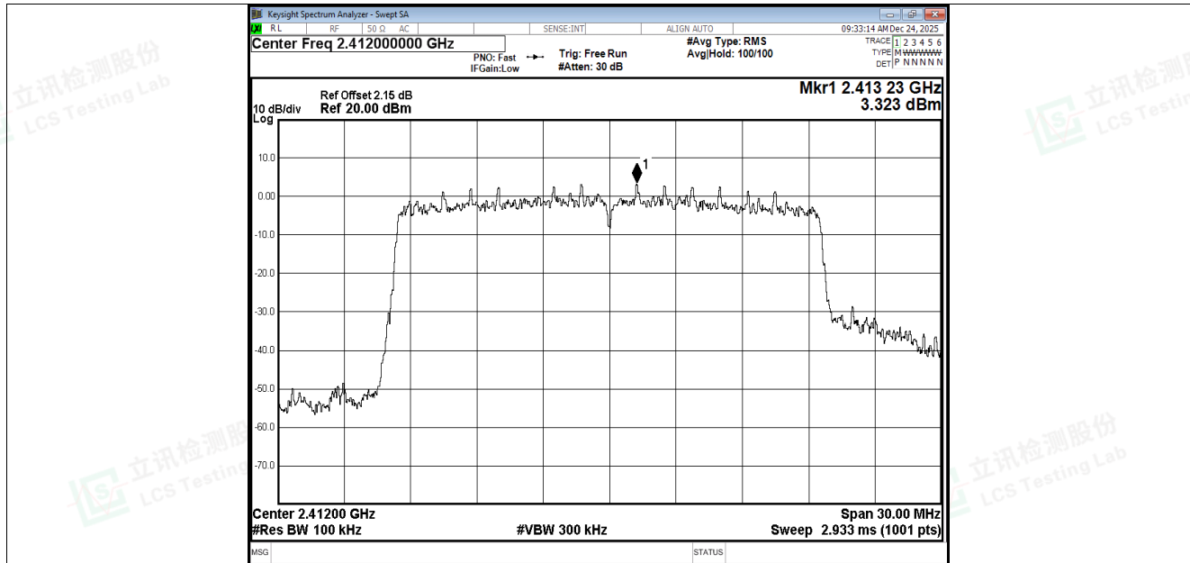
Band Edge NVNT be20 2412MHz Ant2 Ref
