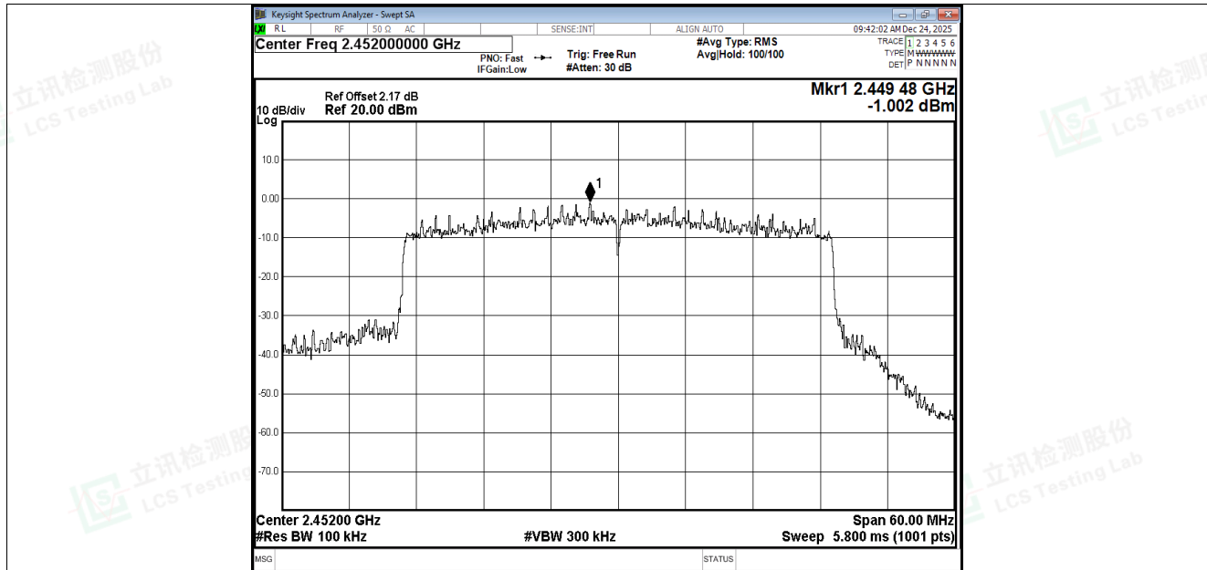
Band Edge NVNT be40 2452MHz Ant2 Ref
