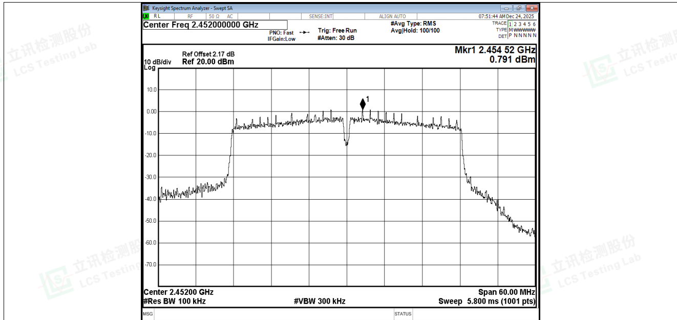
Band Edge NVNT n40 2452MHz Ant1 Ref
