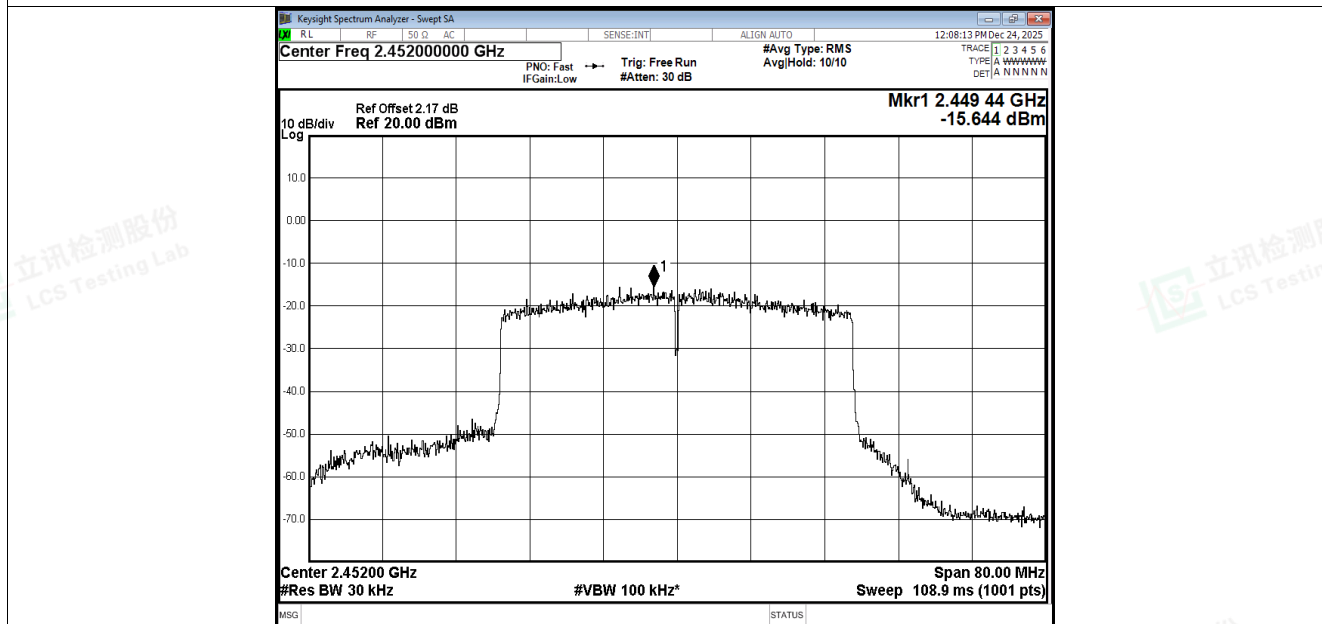
PSD NVNT be40 2452MHz Ant4
