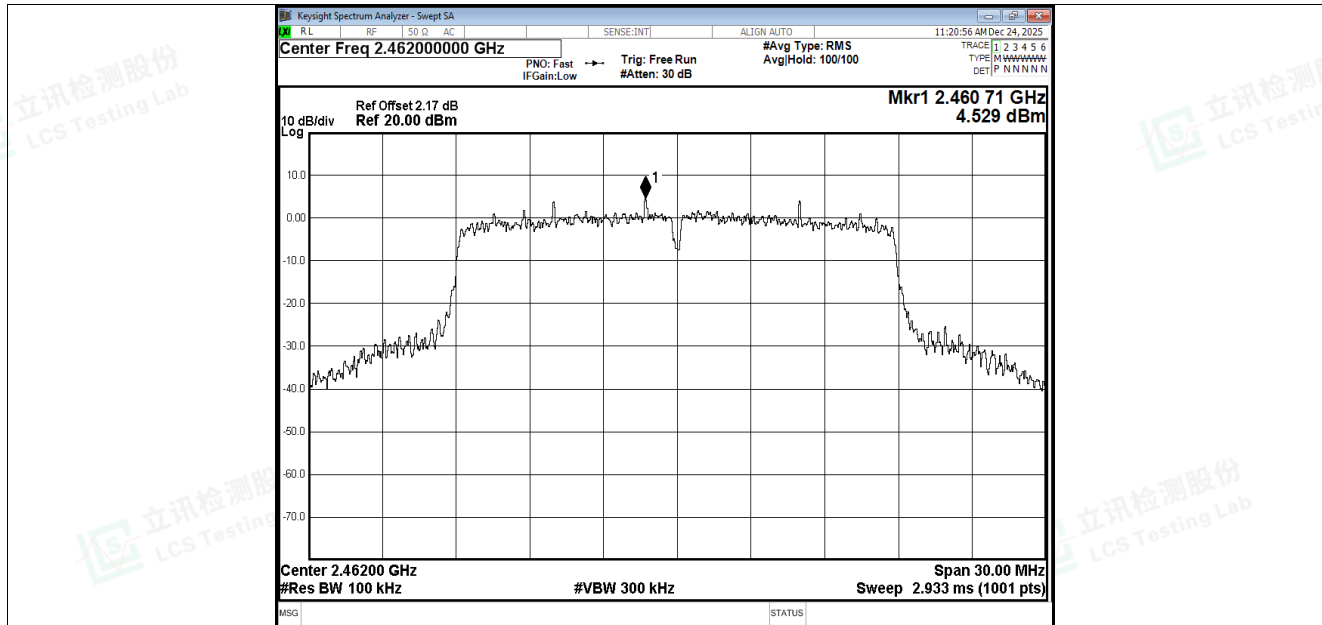
Band Edge NVNT n20 2462MHz Ant4 Ref
