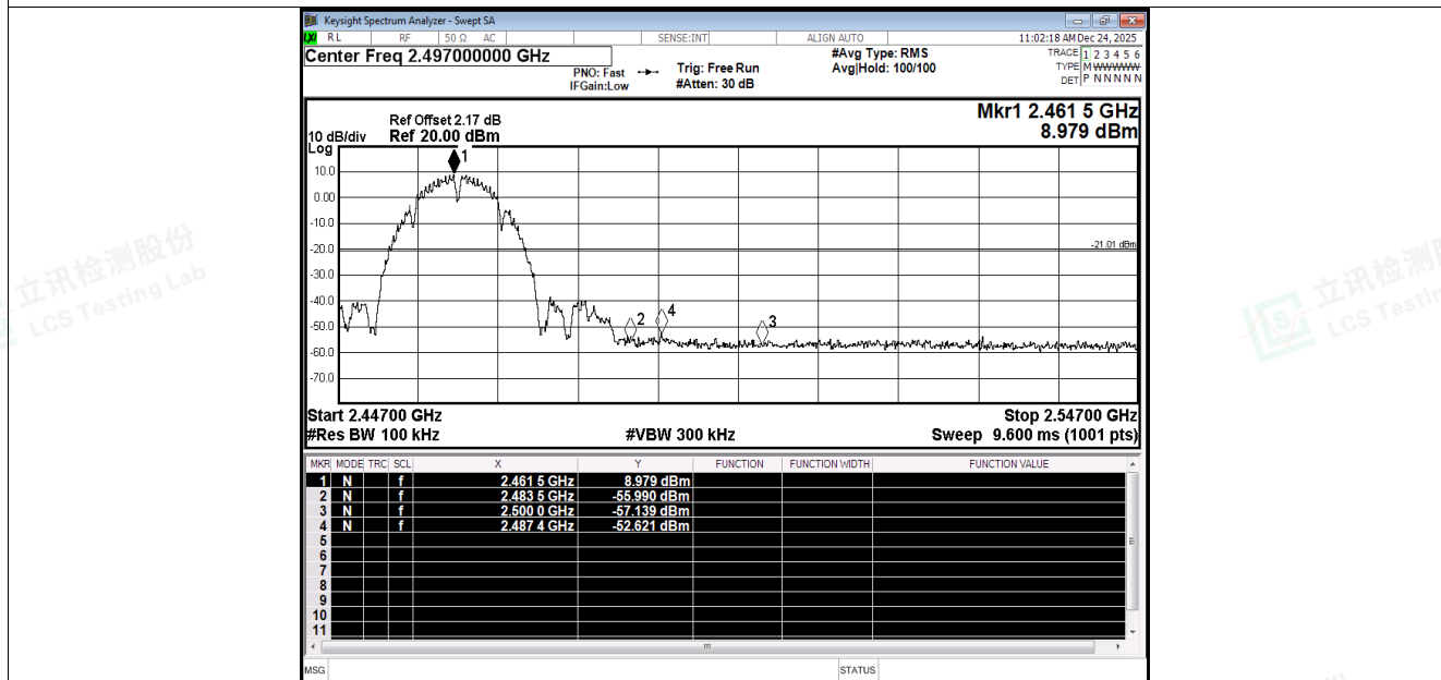
Band Edge NVNT b 2462MHz Ant4 Emission
