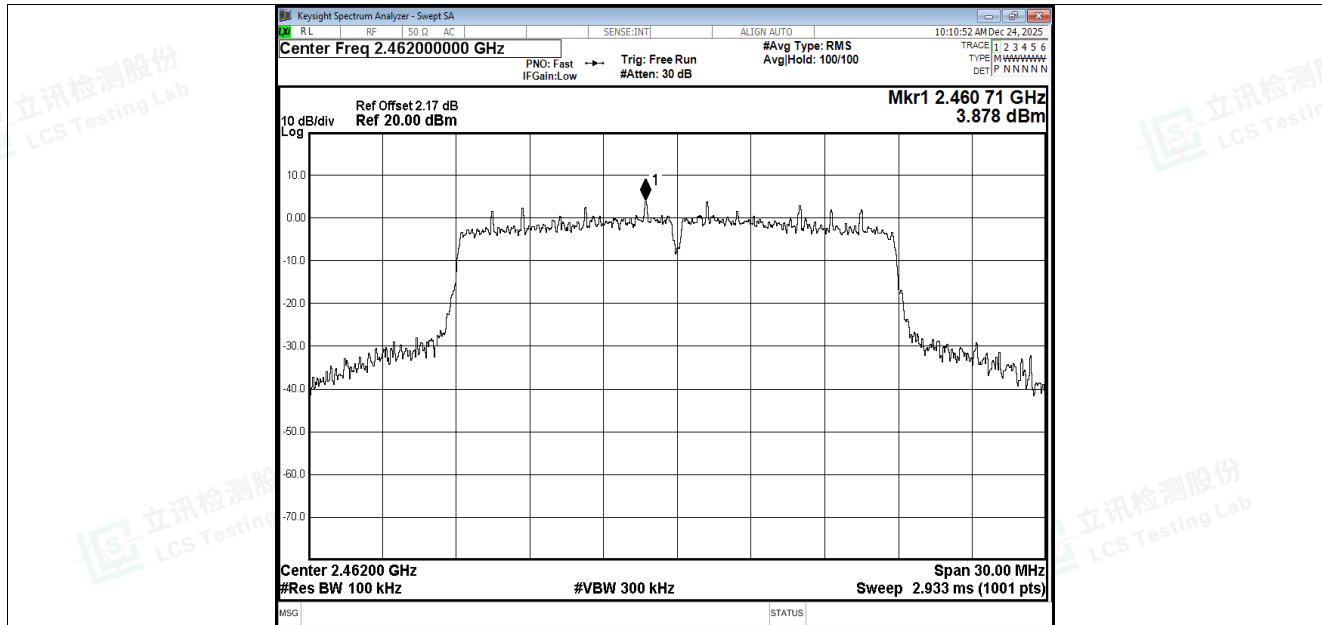
Band Edge NVNT n20 2462MHz Ant3 Ref
