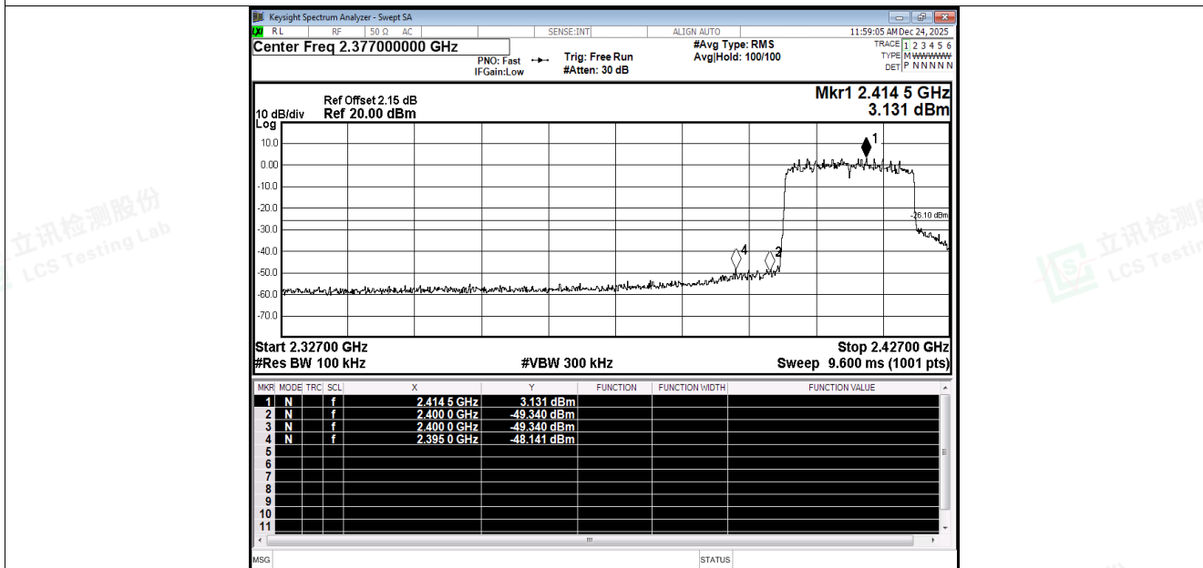
Band Edge NVNT be20 2412MHz Ant4 Emission
