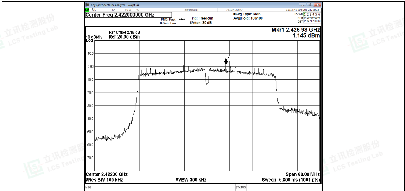
Band Edge NVNT n40 2422MHz Ant3 Ref
