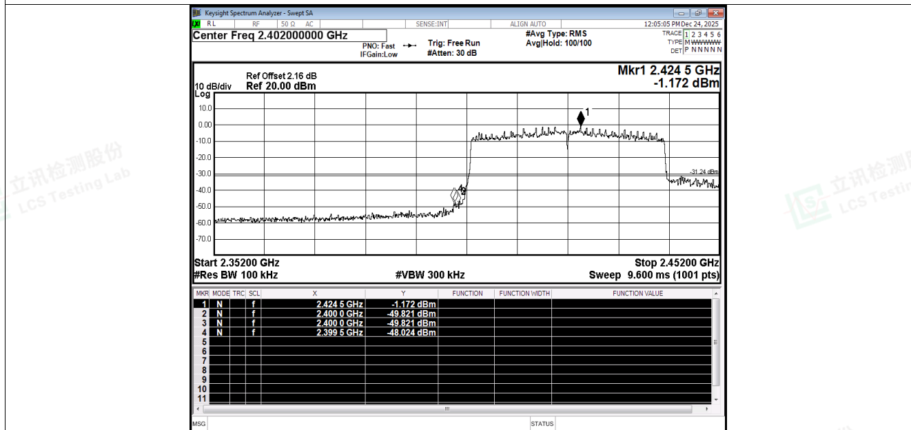
Band Edge NVNT be40 2422MHz Ant4 Emission
