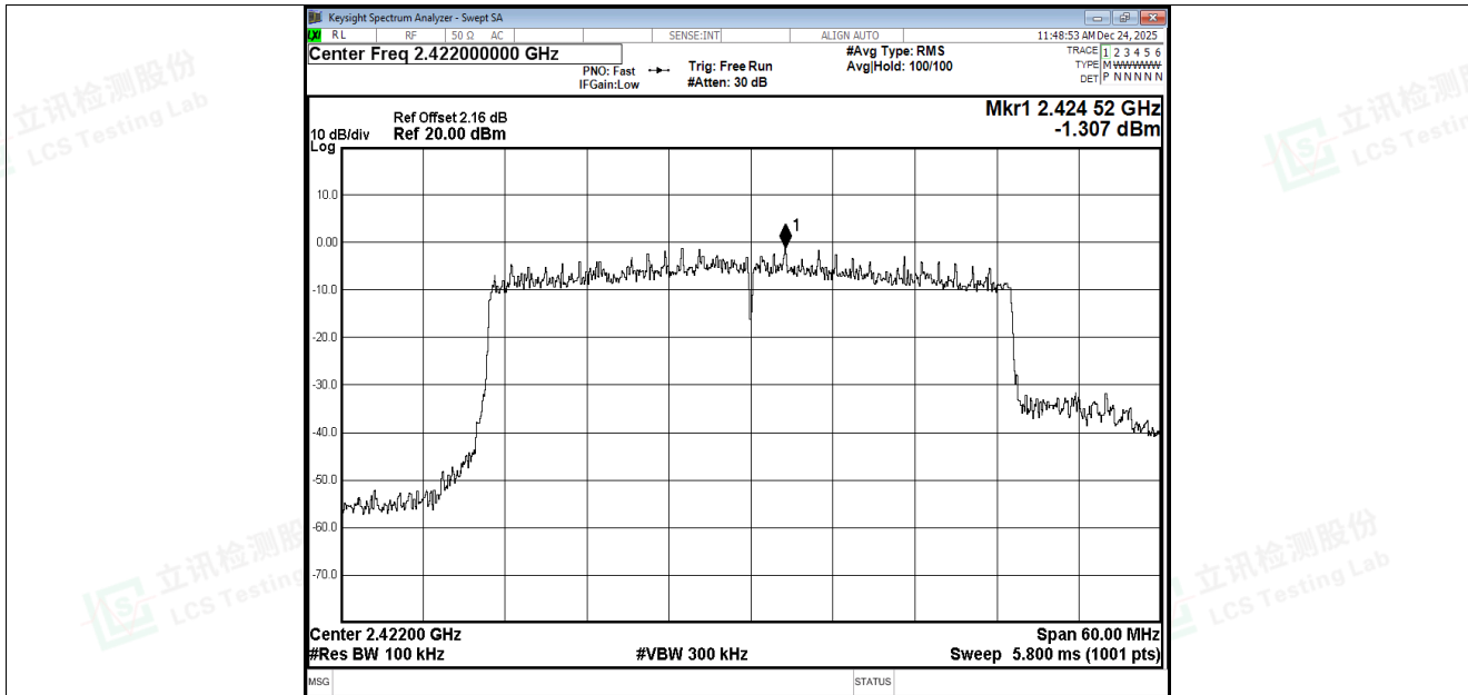
Band Edge NVNT ax40 2422MHz Ant4 Ref
