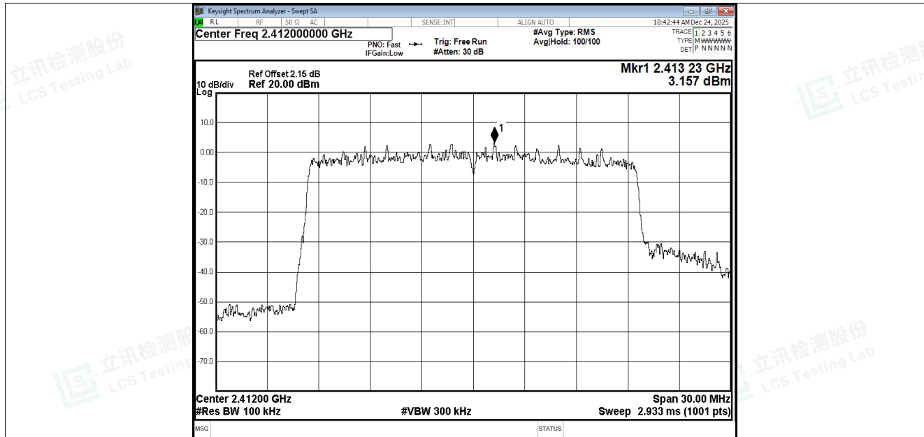
Band Edge NVNT be20 2412MHz Ant3 Ref
