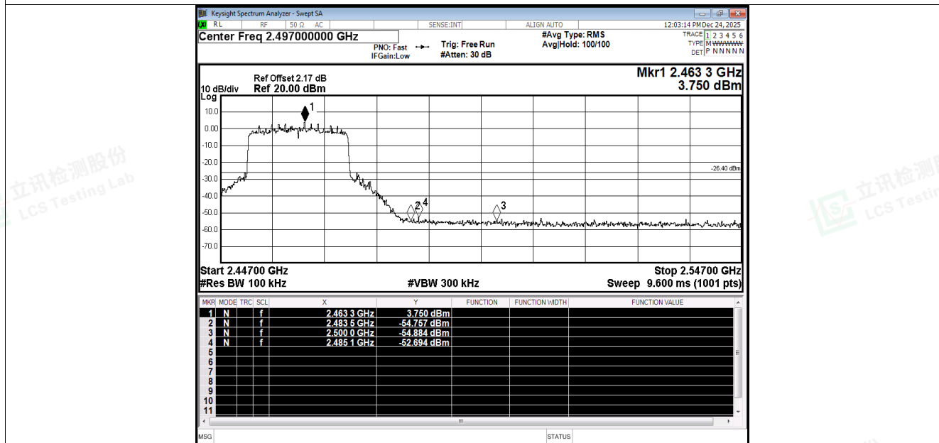
Band Edge NVNT be20 2462MHz Ant4 Emission
