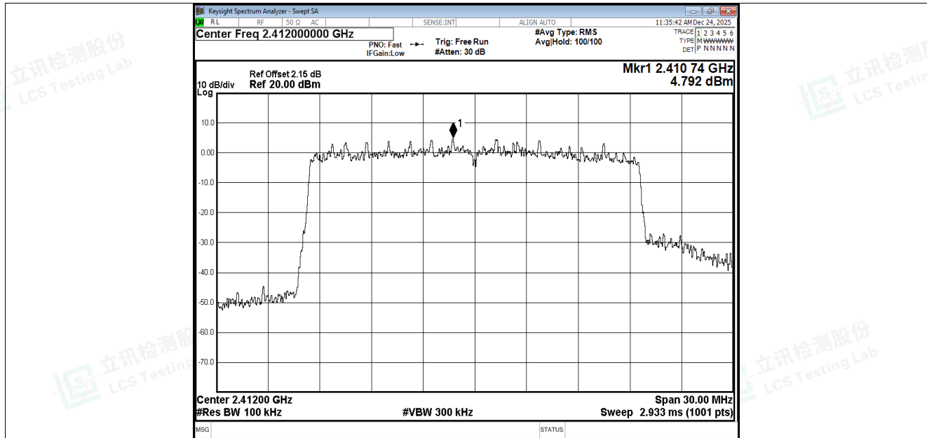
Band Edge NVNT ax20 2412MHz Ant4 Ref
