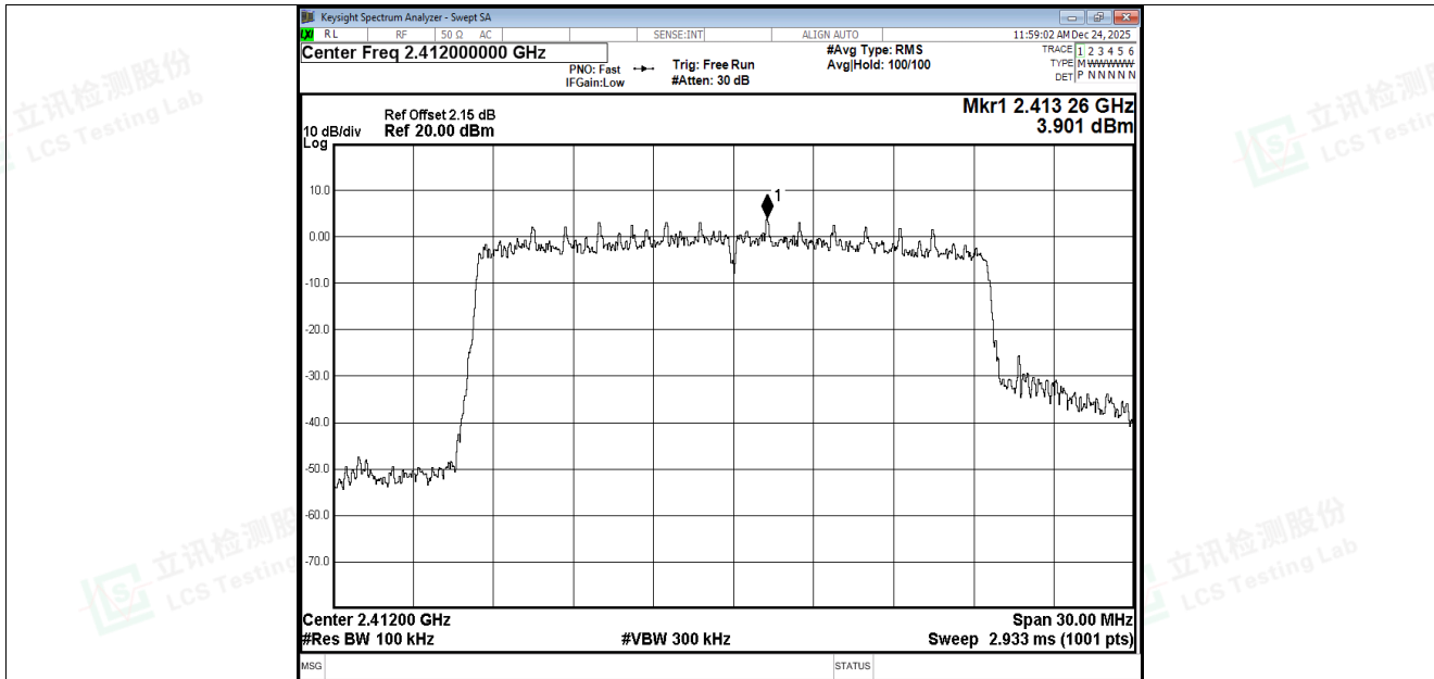
Band Edge NVNT be20 2412MHz Ant4 Ref
