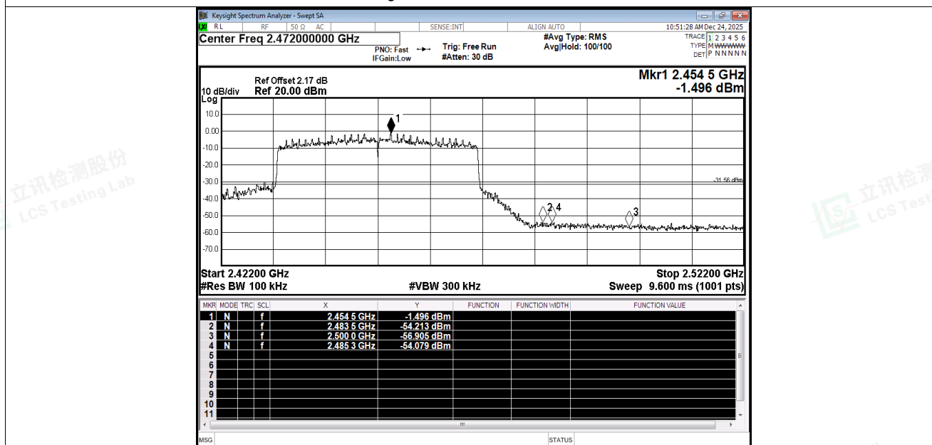
Band Edge NVNT be40 2452MHz Ant3 Emission
