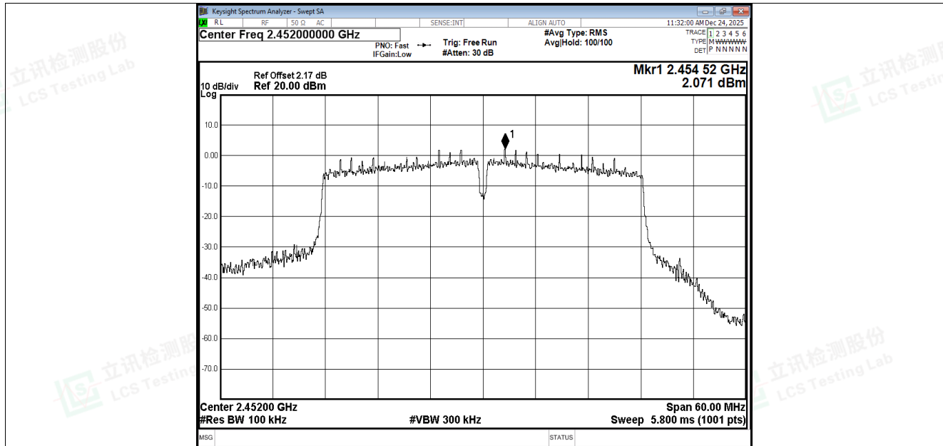
Band Edge NVNT n40 2452MHz Ant4 Ref
