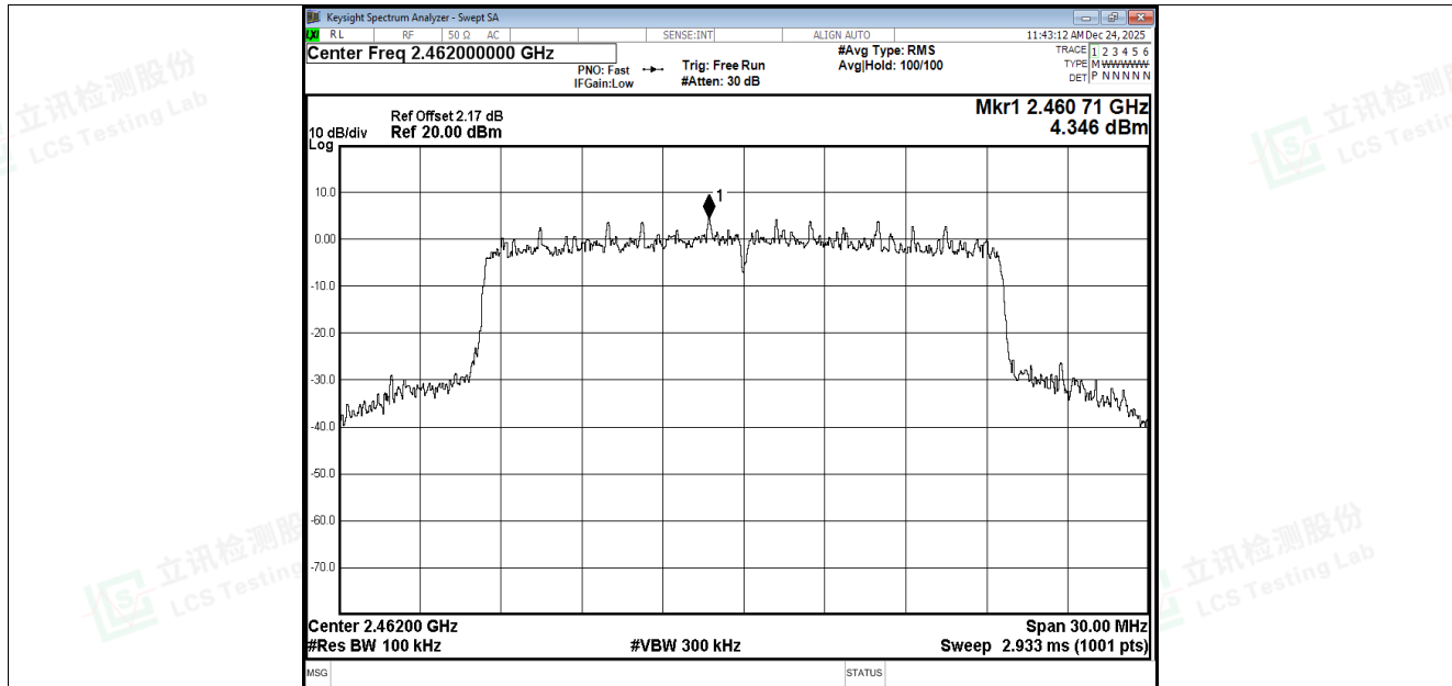
Band Edge NVNT ax20 2462MHz Ant4 Ref
