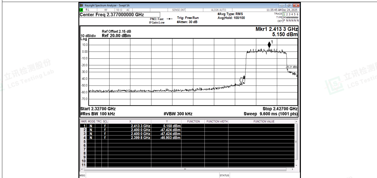
Band Edge NVNT ax20 2412MHz Ant4 Emission
