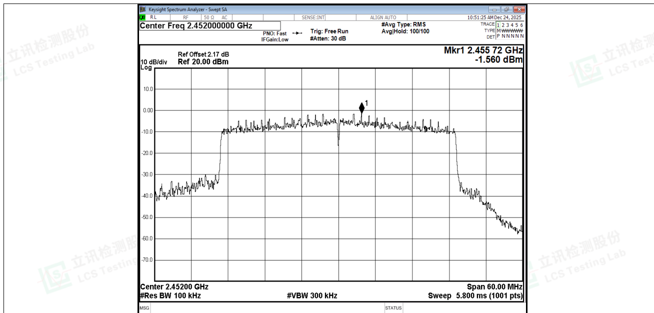
Band Edge NVNT be40 2452MHz Ant3 Ref
