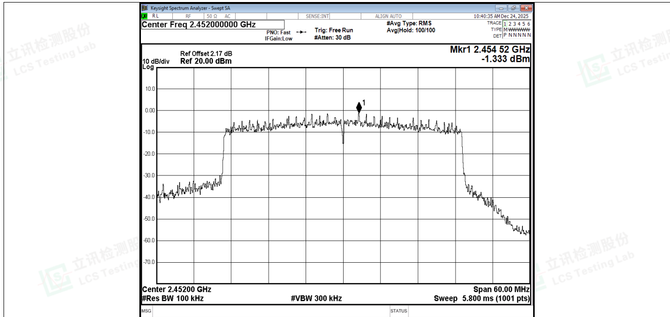
Band Edge NVNT ax40 2452MHz Ant3 Ref
