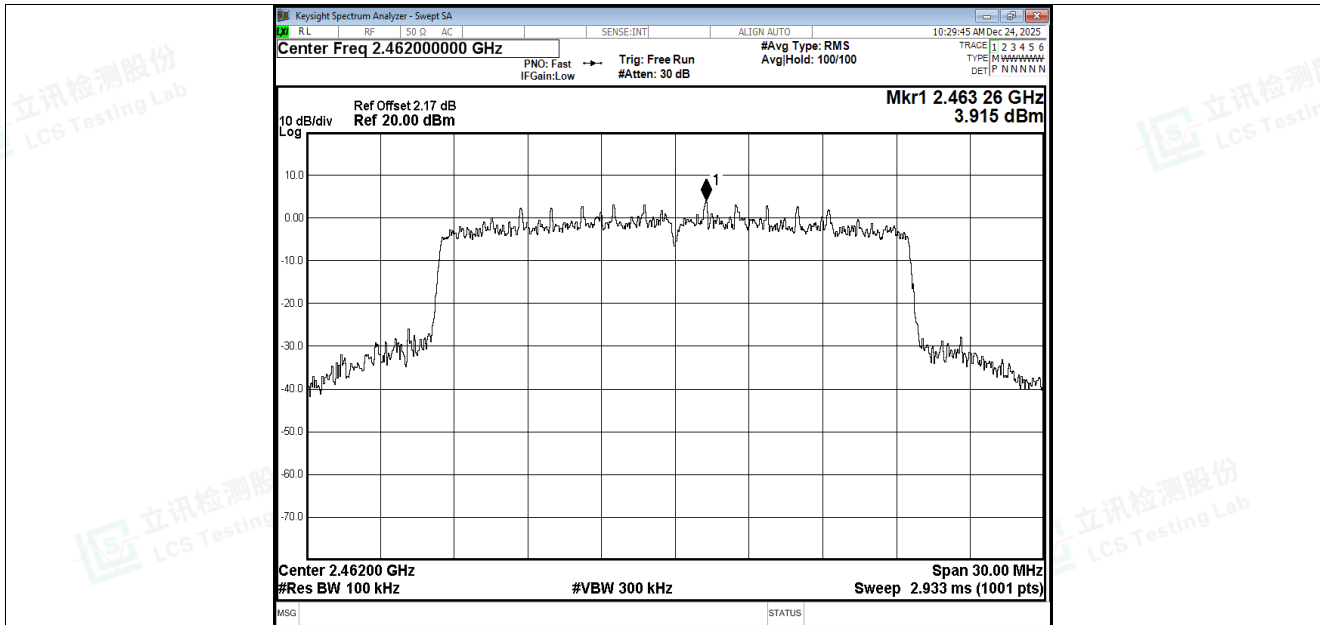
Band Edge NVNT ax20 2462MHz Ant3 Ref
