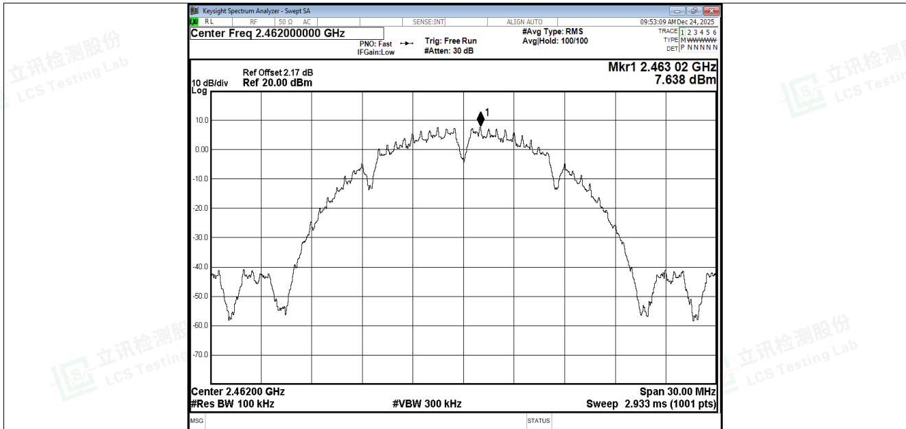
Band Edge NVNT b 2462MHz Ant3 Ref
