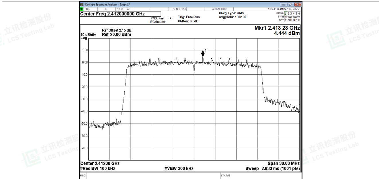
Band Edge NVNT ax20 2412MHz Ant3 Ref
