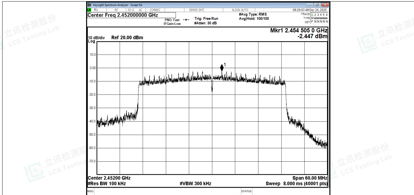
Tx. Spurious NVNT be40 2452MHz Ant1 Ref
