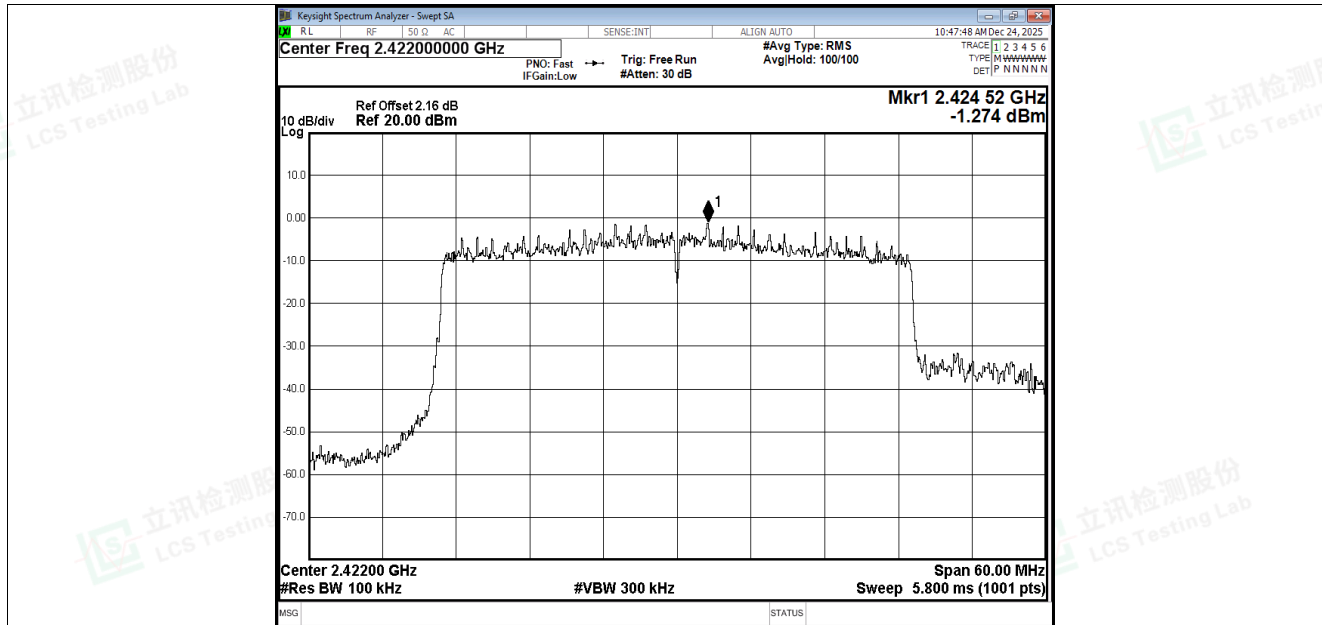
Band Edge NVNT be40 2422MHz Ant3 Ref
