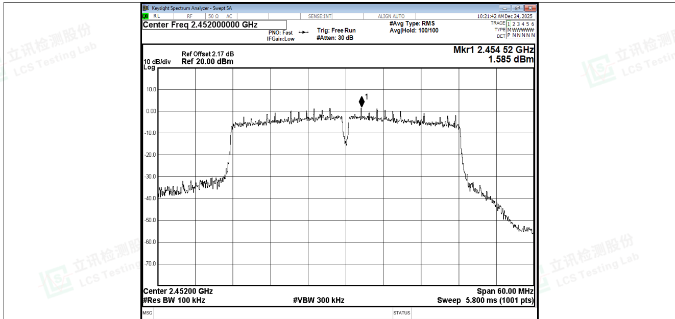
Band Edge NVNT n40 2452MHz Ant3 Ref
