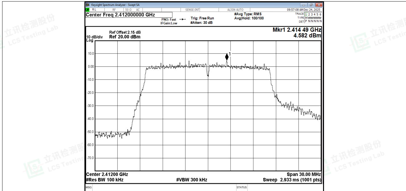
Band Edge NVNT g 2412MHz Ant3 Ref
