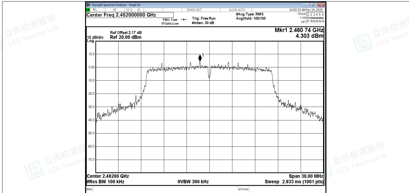
Band Edge NVNT g 2462MHz Ant3 Ref
