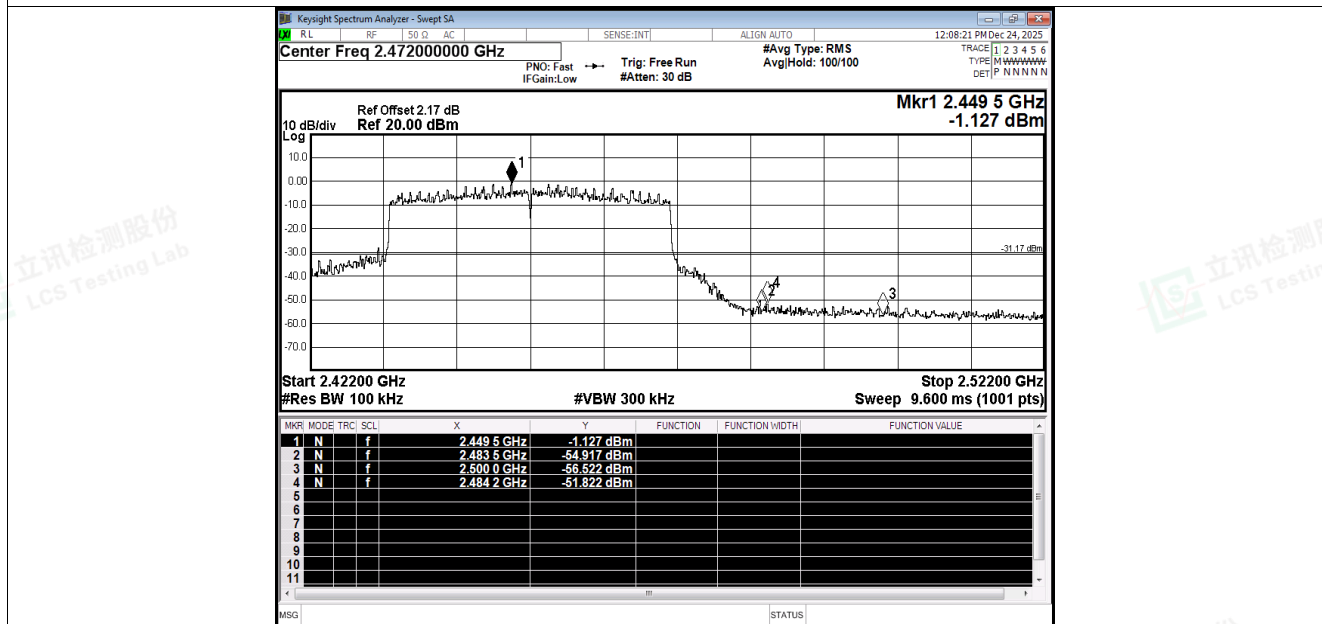
Band Edge NVNT be40 2452MHz Ant4 Emission
