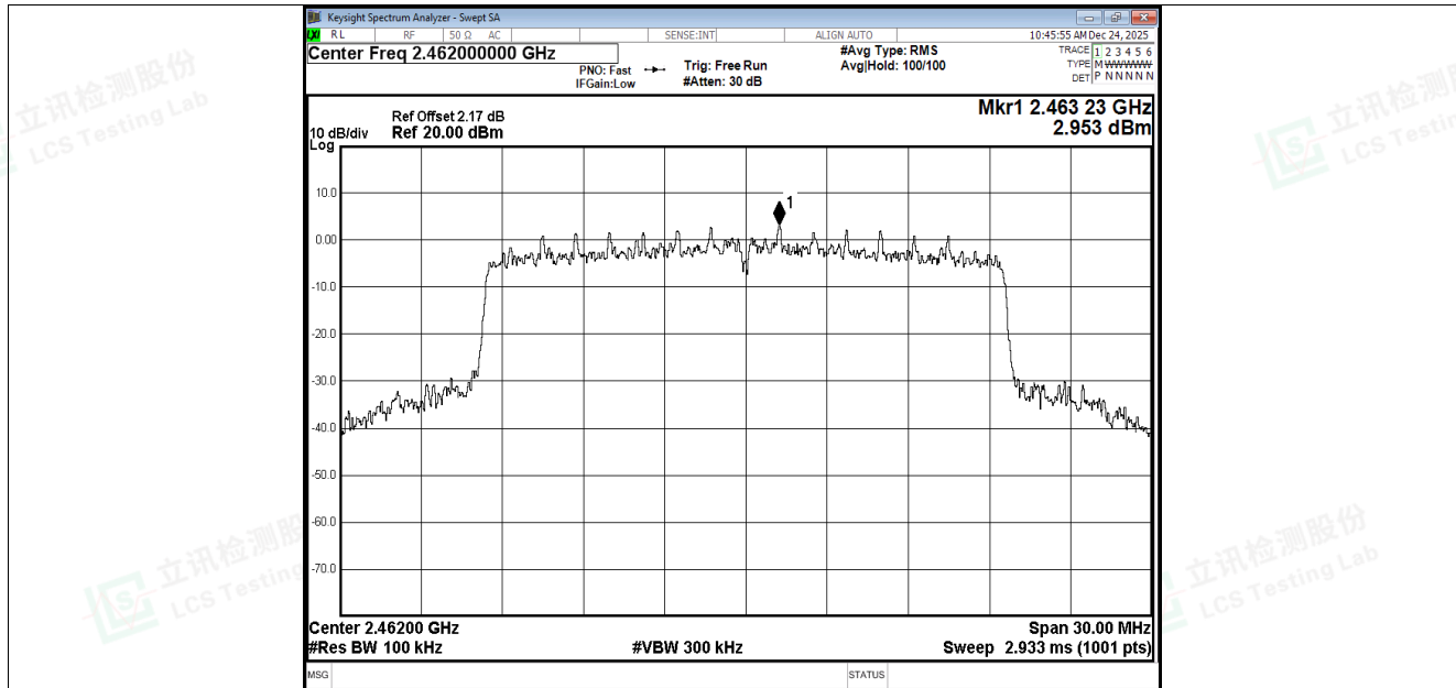
Band Edge NVNT be20 2462MHz Ant3 Ref
