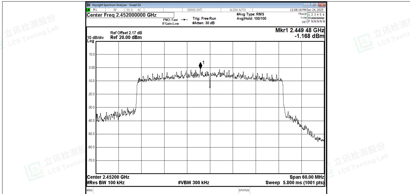
Band Edge NVNT be40 2452MHz Ant4 Ref
