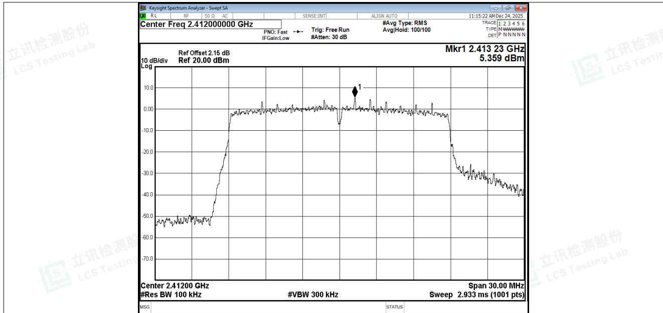
Band Edge NVNT n20 2412MHz Ant4 Ref
