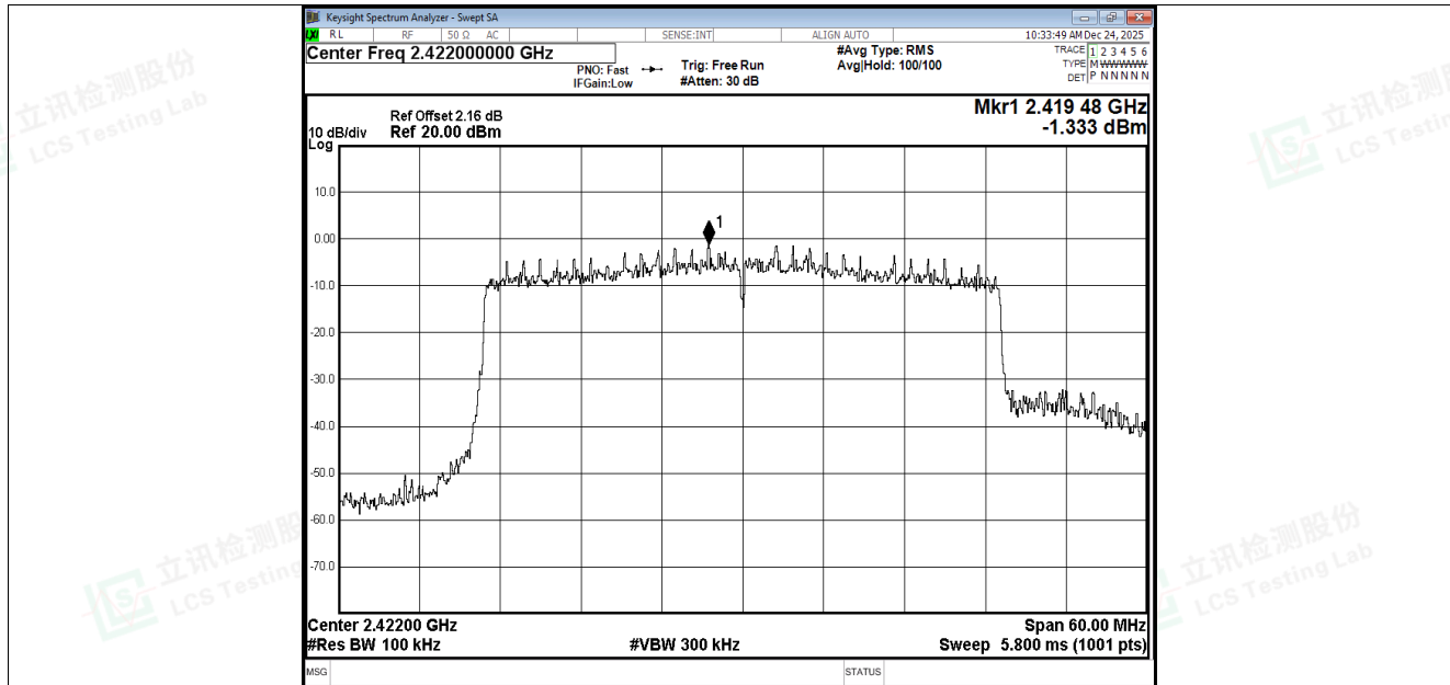
Band Edge NVNT ax40 2422MHz Ant3 Ref
