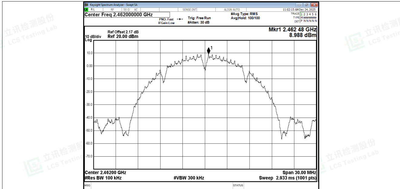
Band Edge NVNT b 2462MHz Ant4 Ref
