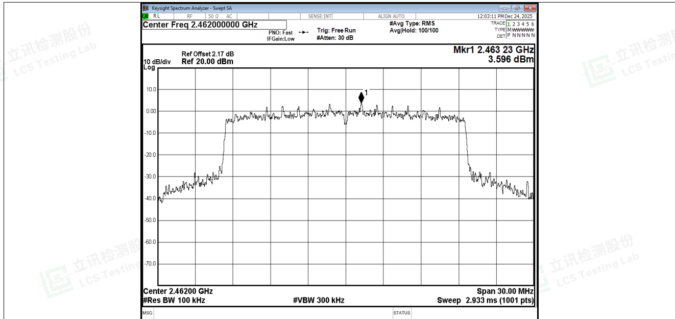
Band Edge NVNT be20 2462MHz Ant4 Ref
