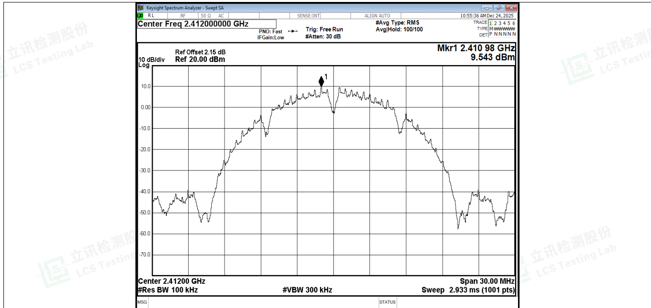
Band Edge NVNT b 2412MHz Ant4 Ref
