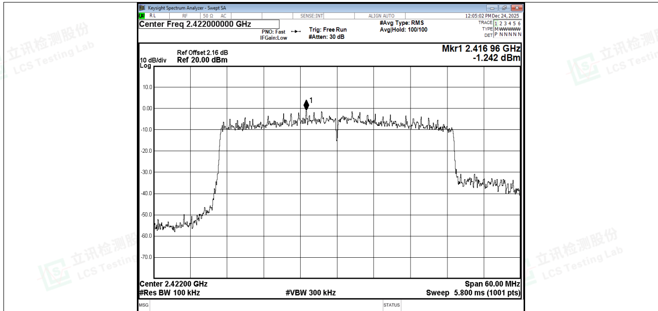
Band Edge NVNT be40 2422MHz Ant4 Ref
