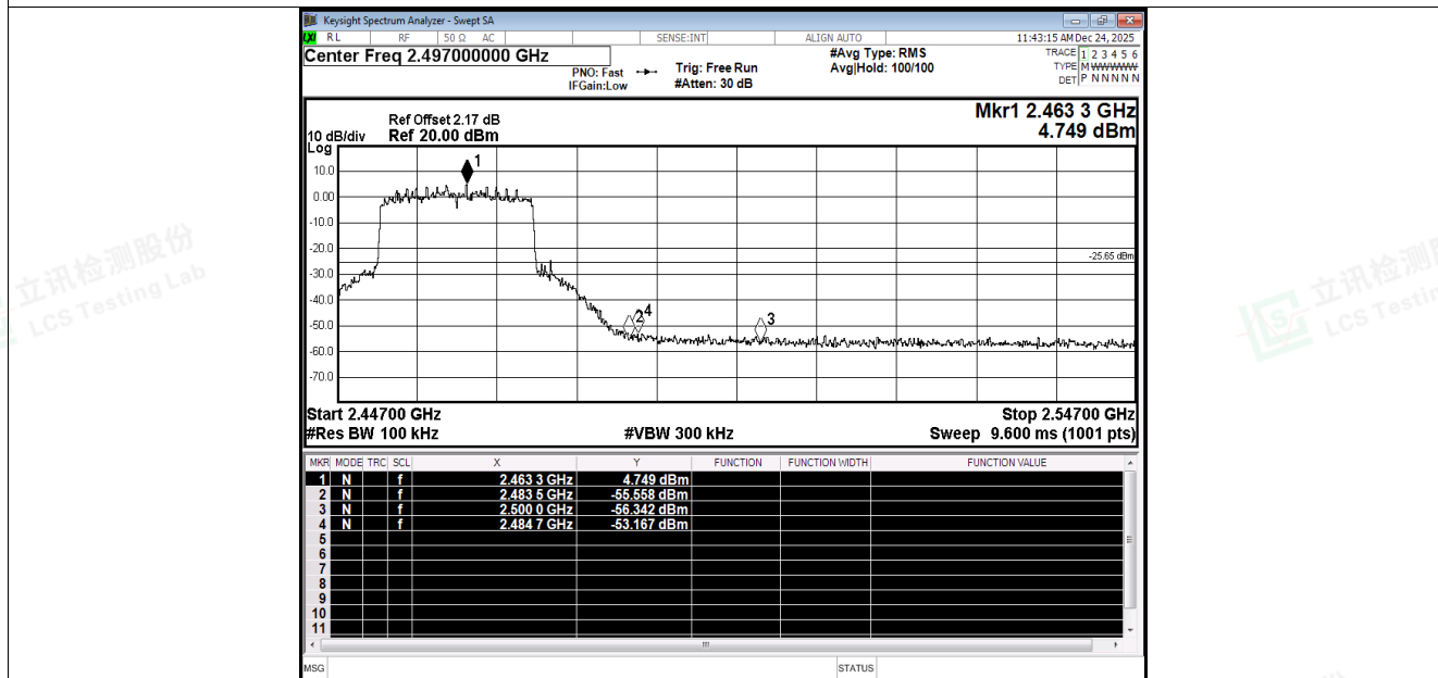
Band Edge NVNT ax20 2462MHz Ant4 Emission
