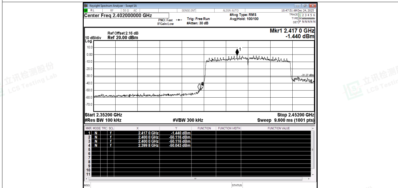
Band Edge NVNT be40 2422MHz Ant3 Emission
