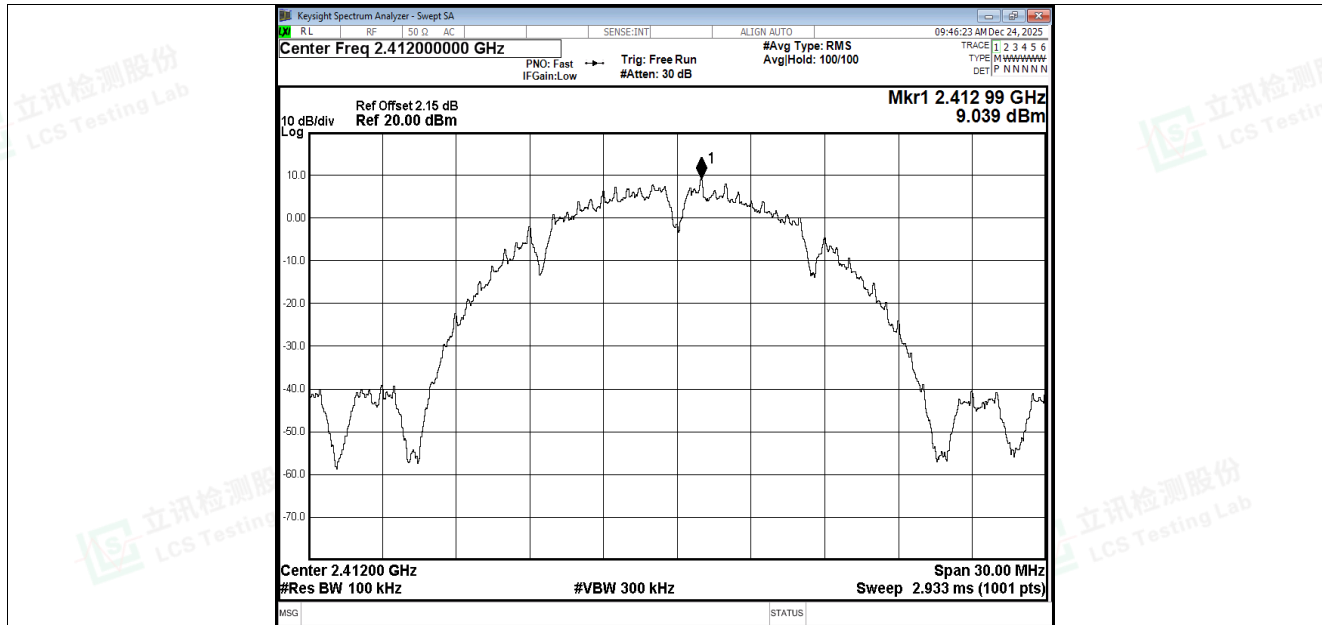
Band Edge NVNT b 2412MHz Ant3 Ref
