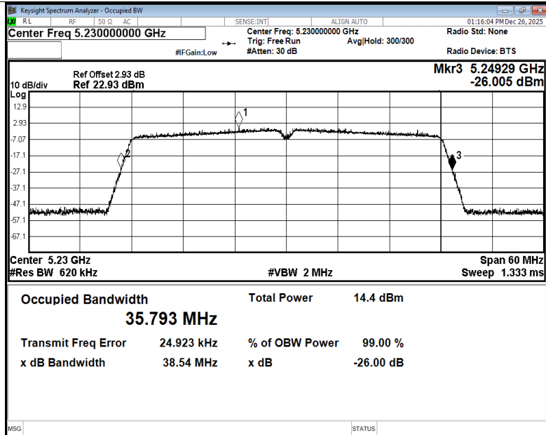
-26dB Bandwidth NVNT n40 5230MHz Ant5
