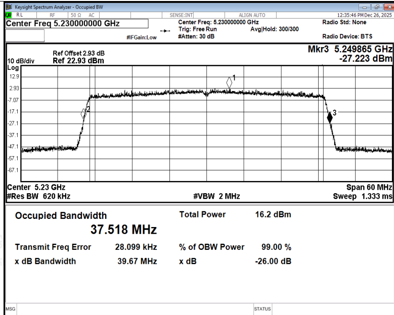
-26dB Bandwidth NVNT be40 5230MHz Ant4
