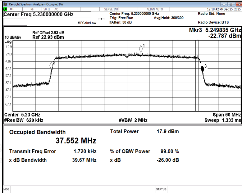
-26dB Bandwidth NVNT be40 5230MHz Ant1
