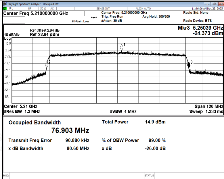
-26dB Bandwidth NVNT ax80 5210MHz Ant1
