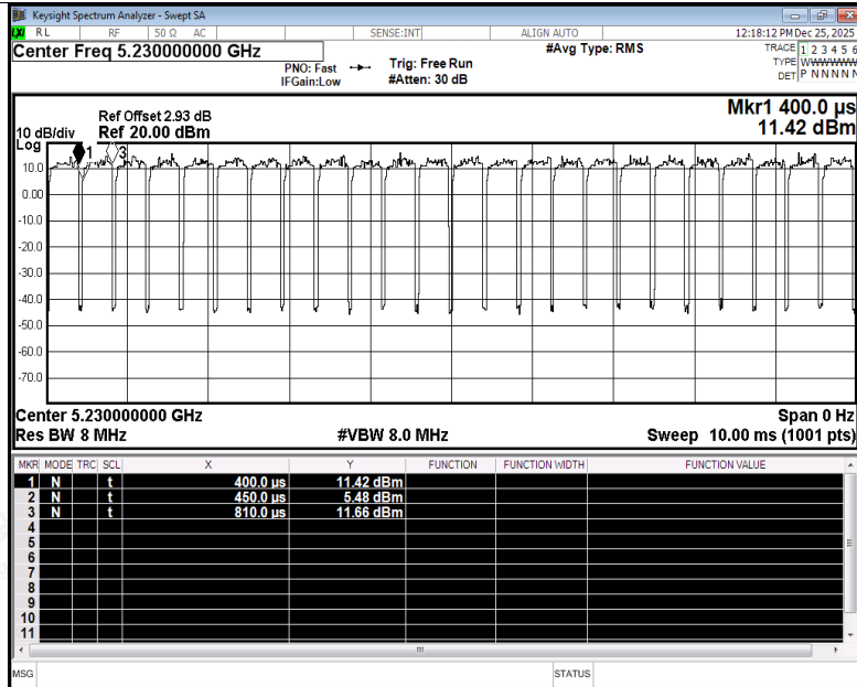
Duty Cycle NVNT be40 5230MHz Ant1
