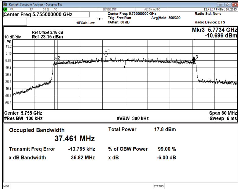
-6dB Bandwidth NVNT be40 5755MHz Ant4
