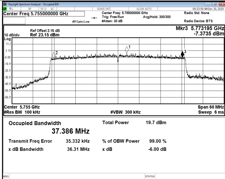
-6dB Bandwidth NVNT be40 5755MHz Ant1
