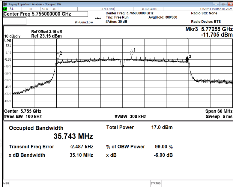
-6dB Bandwidth NVNT n40 5755MHz Ant4
