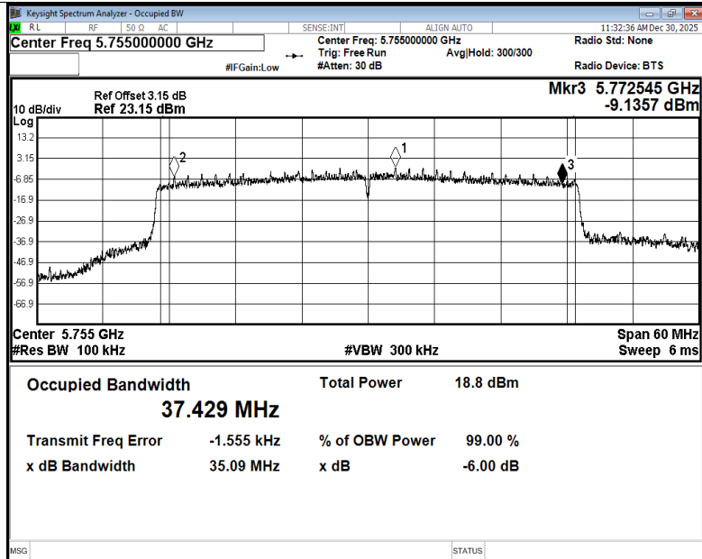
-6dB Bandwidth NVNT be40 5755MHz Ant3
