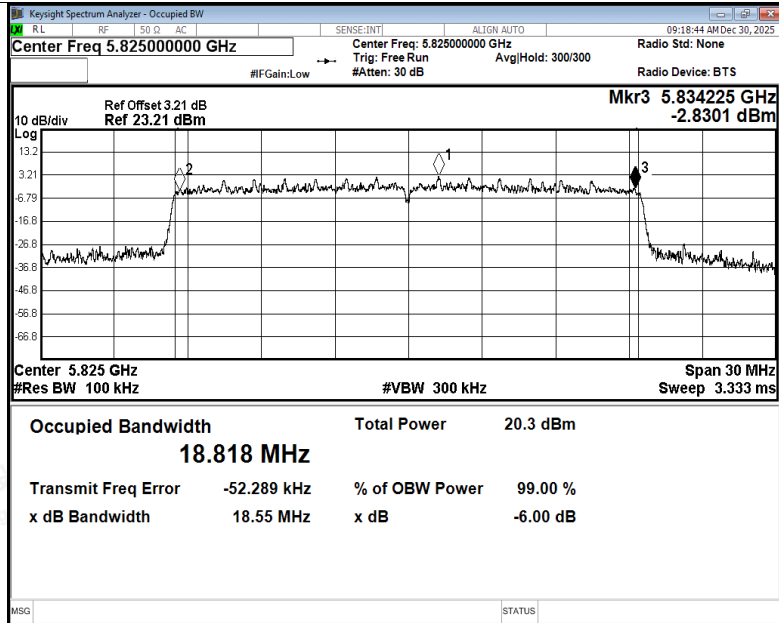
-6dB Bandwidth NVNT be20 5825MHz Ant1
