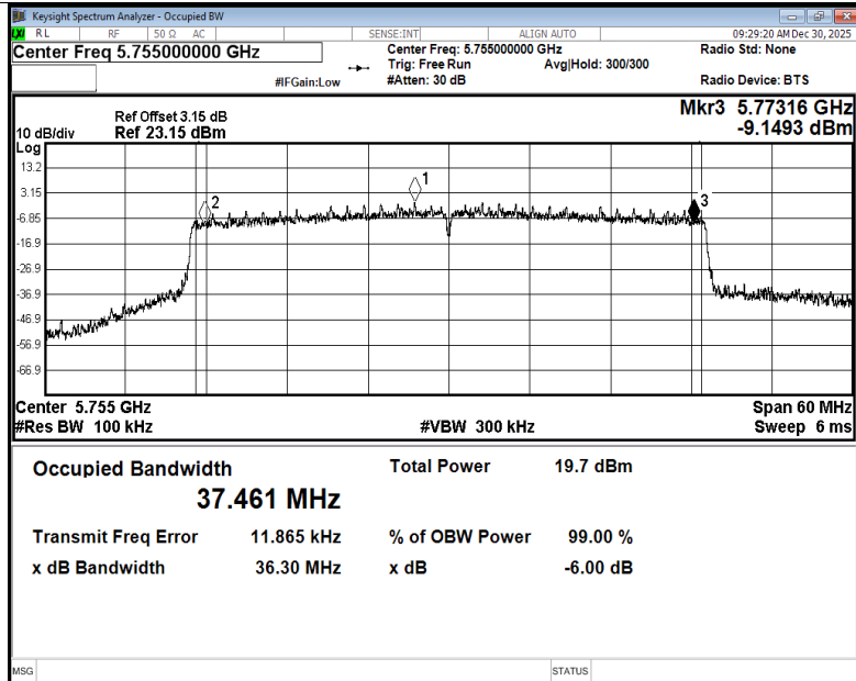
-6dB Bandwidth NVNT ax40 5755MHz Ant1
