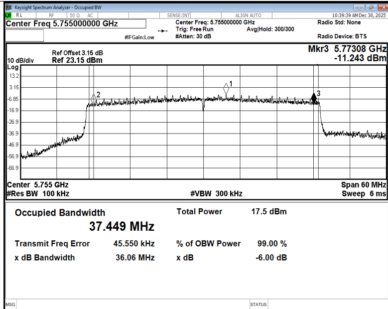
-6dB Bandwidth NVNT be40 5755MHz Ant2
