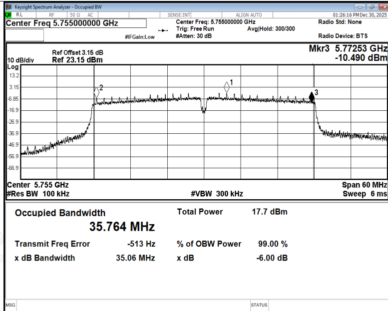
-6dB Bandwidth NVNT n40 5755MHz Ant5
