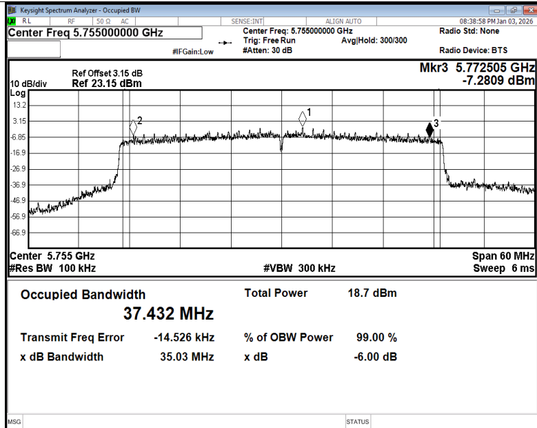
-6dB Bandwidth NVNT be40 5755MHz Ant5
