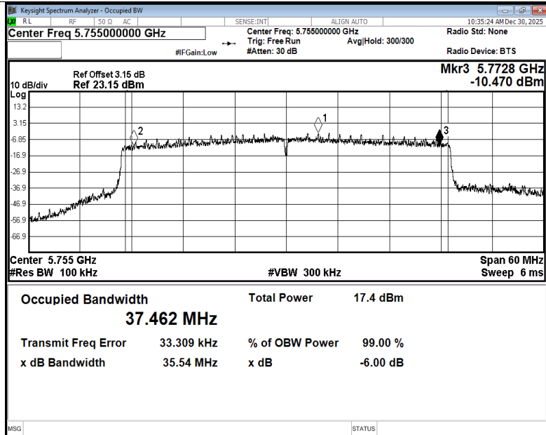
-6dB Bandwidth NVNT ax40 5755MHz Ant2
