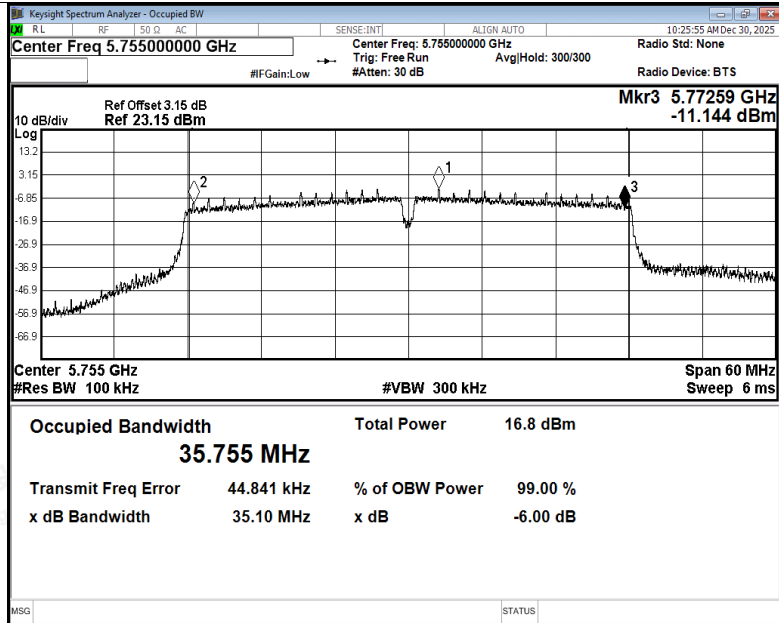
-6dB Bandwidth NVNT n40 5755MHz Ant2
