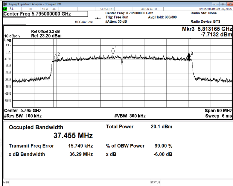
-6dB Bandwidth NVNT be40 5795MHz Ant1
