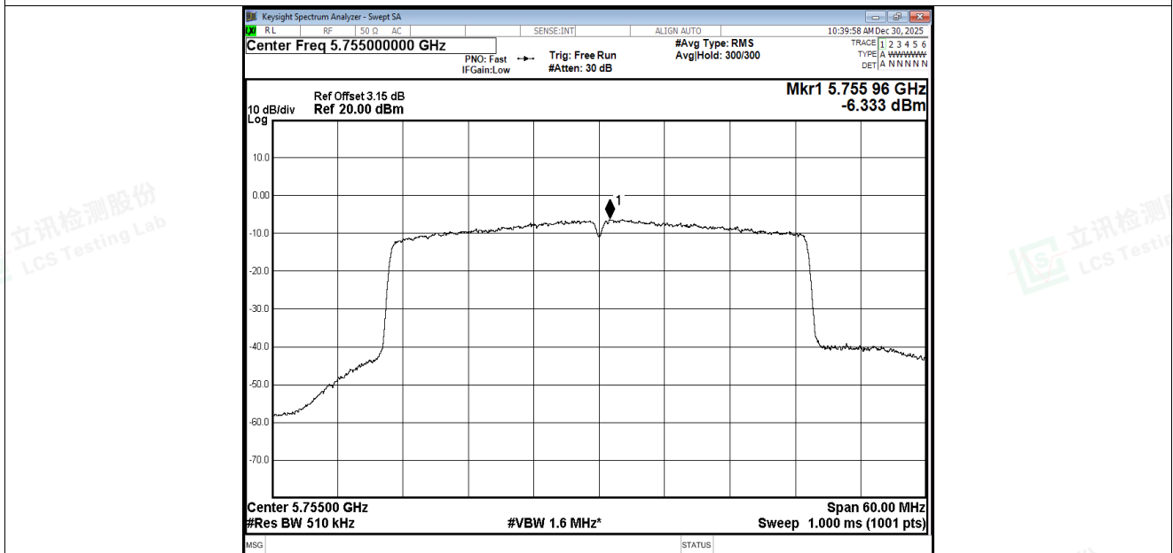
PSD NVNT be40 5755MHz Ant2
