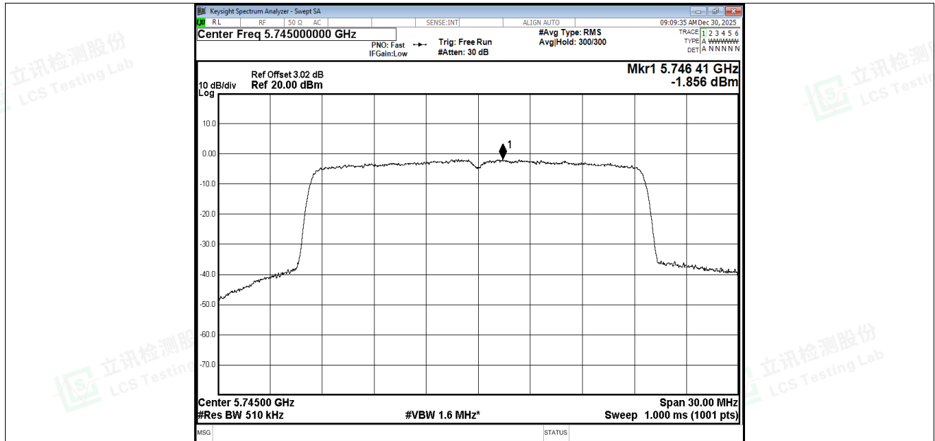
PSD NVNT ax20 5745MHz Ant1
