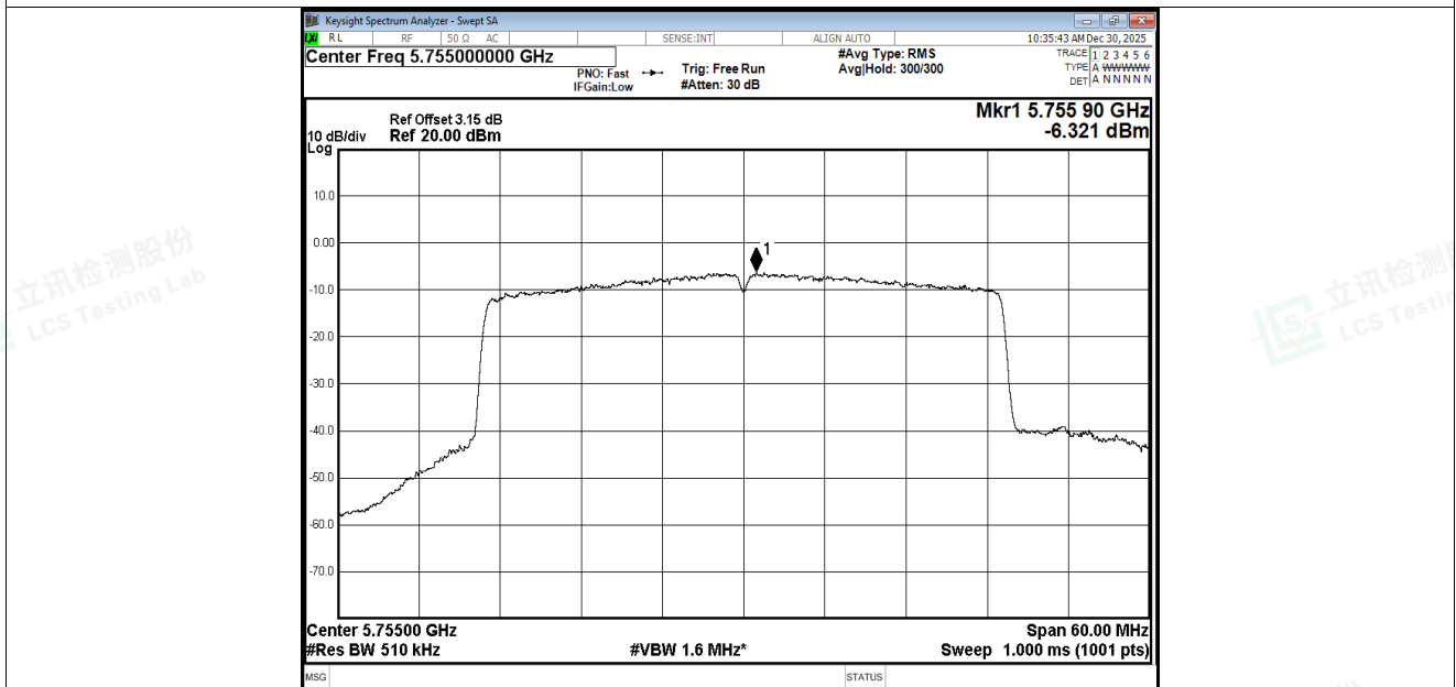
PSD NVNT ax40 5755MHz Ant2
