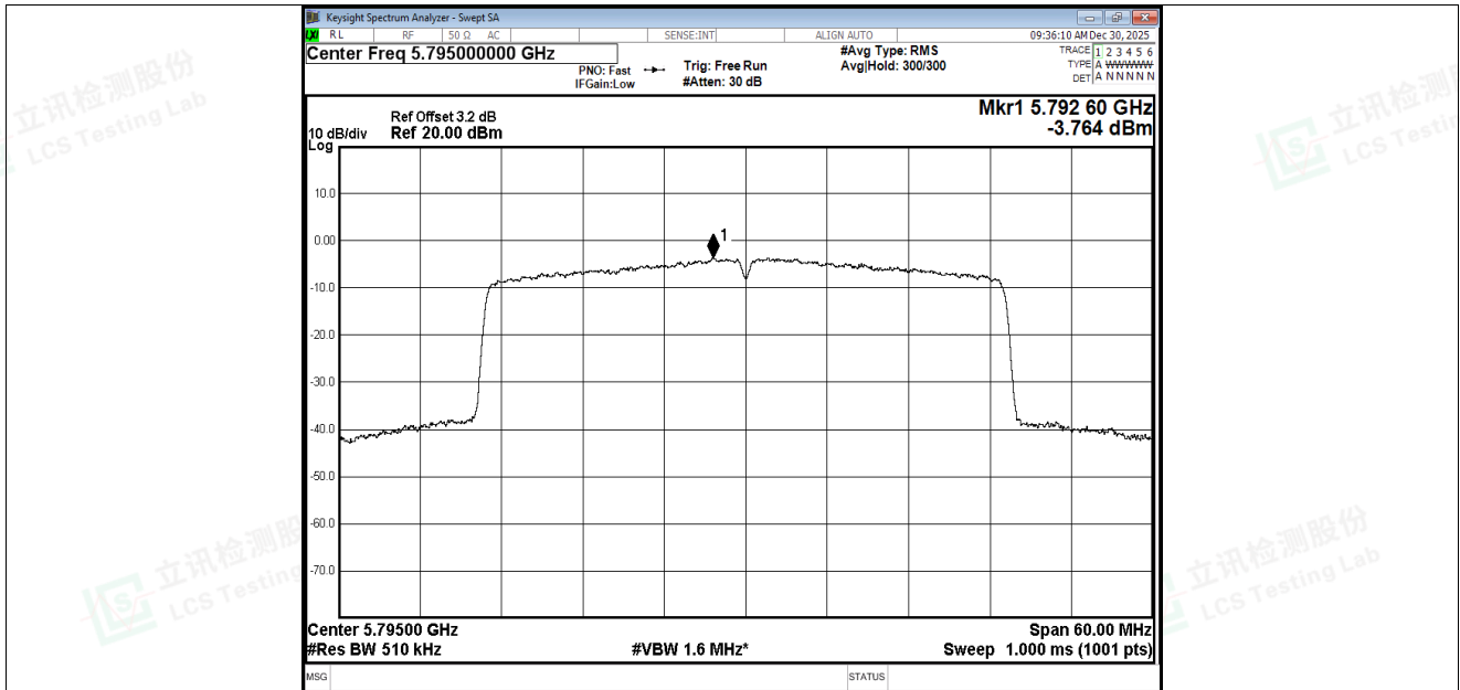
PSD NVNT be40 5795MHz Ant1
