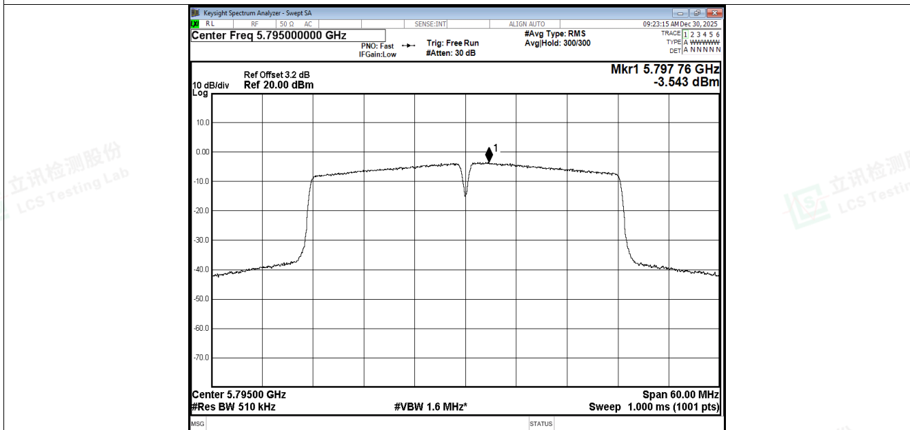
PSD NVNT n40 5795MHz Ant1
