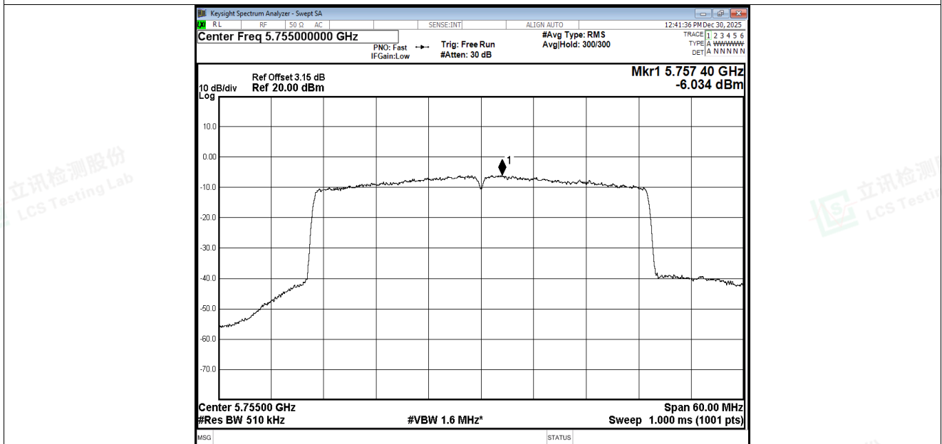
PSD NVNT be40 5755MHz Ant4
