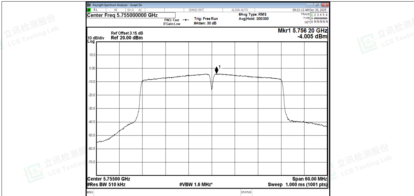
PSD NVNT n40 5755MHz Ant1
