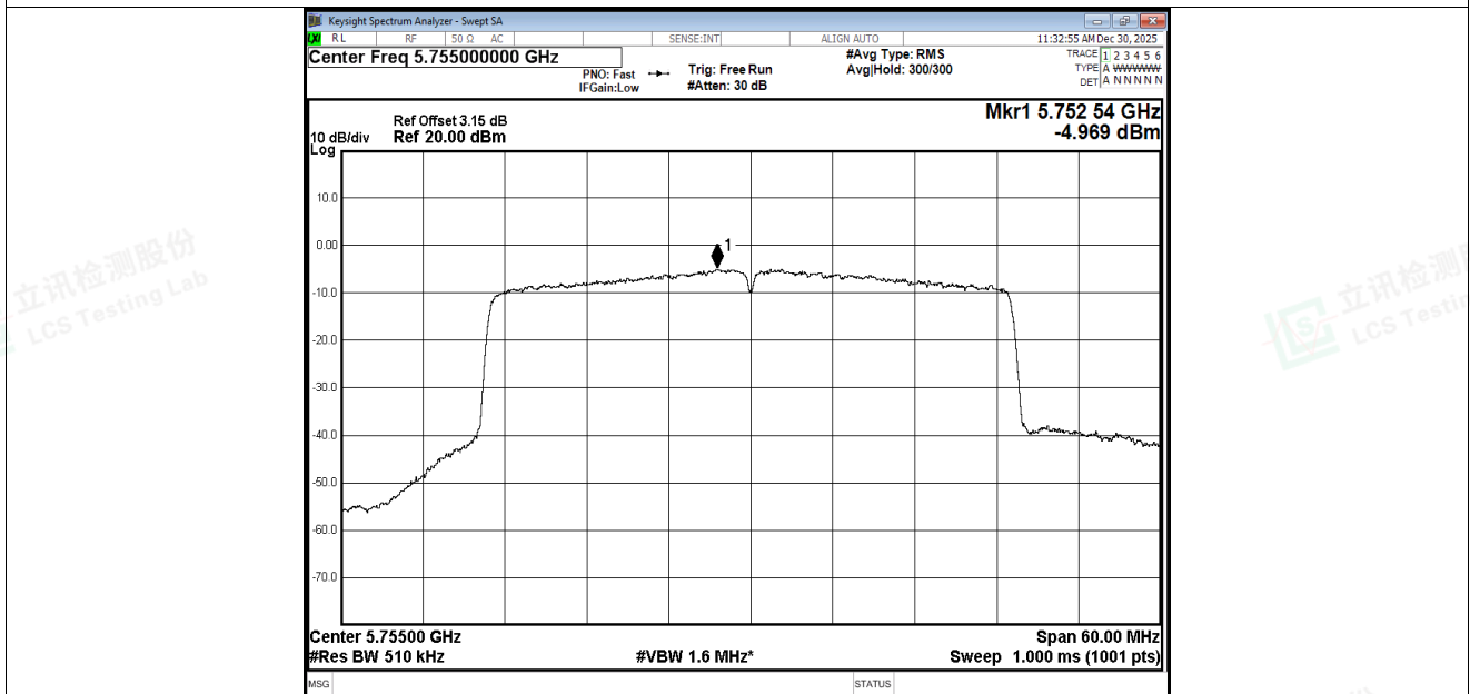
PSD NVNT be40 5755MHz Ant3
