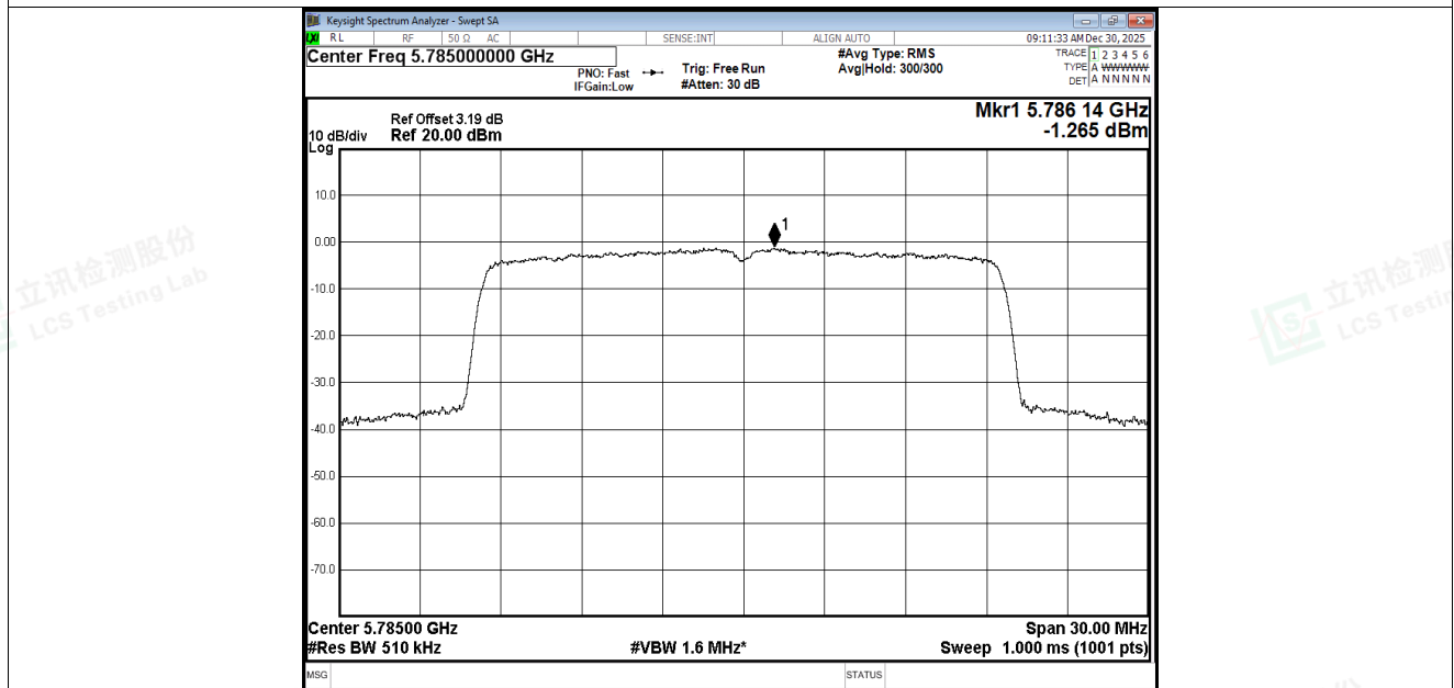
PSD NVNT ax20 5785MHz Ant1
