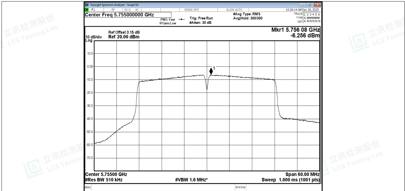
PSD NVNT n40 5755MHz Ant2
