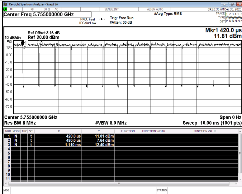
Duty Cycle NVNT n40 5755MHz Ant1
