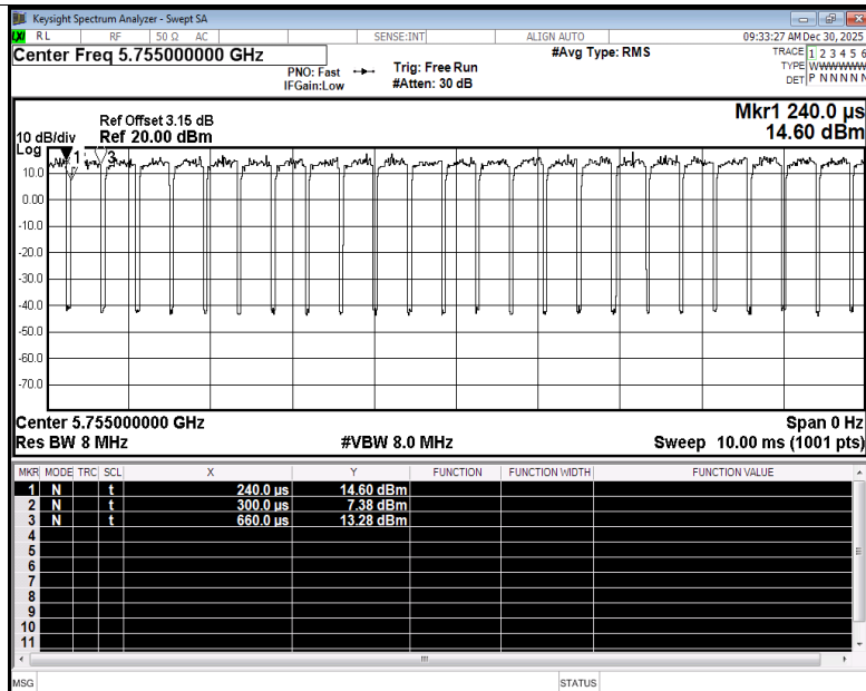
Duty Cycle NVNT be40 5755MHz Ant1
