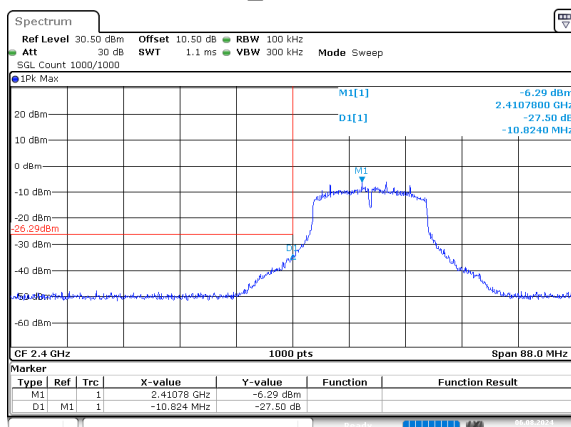
n20_2412MHz
