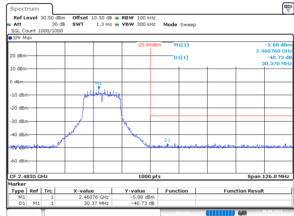
g_2462MHz
