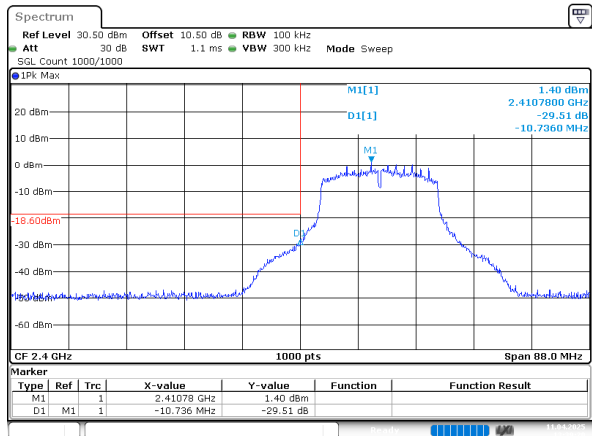
802.11n20_2412MHz
