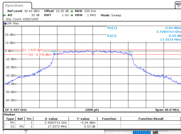
802.11n20_2437MHz
