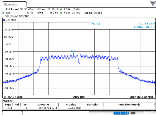
802.11g_2437MHz
