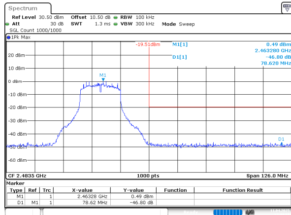
802.11n20_2462MHz
