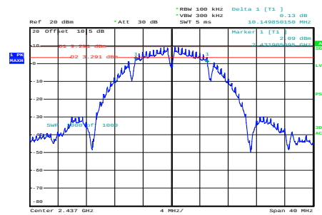
b_2437MHz_Chain 0
