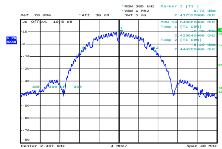
b_2437MHz_Chain 0
