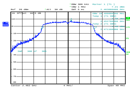
n20_2462MHz_Chain 0
