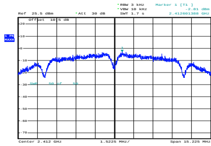
b_2412MHz_Chain 0
