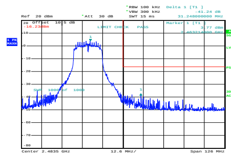
n20_2462MHz_Chain 0
