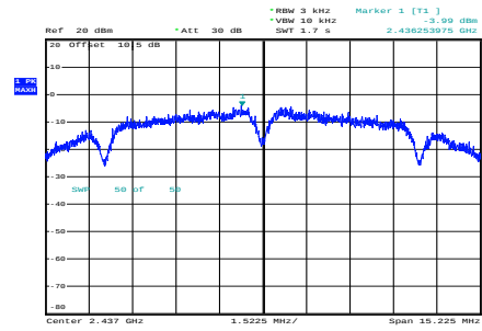
b_2437MHz_Chain 0
