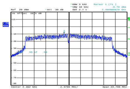
n20_2462MHz_Chain 0
