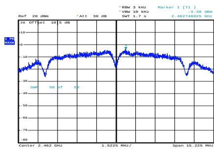
b_2462MHz_Chain 0
