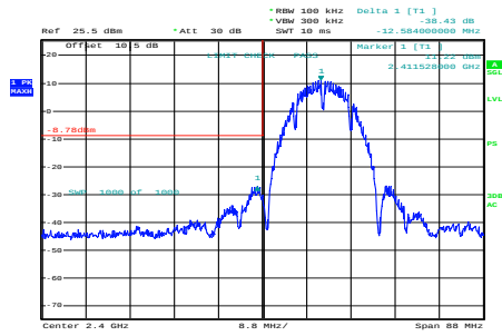
b_2412MHz_Chain 0
