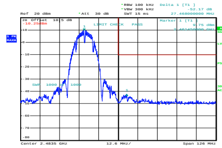
b_2462MHz_Chain 0
