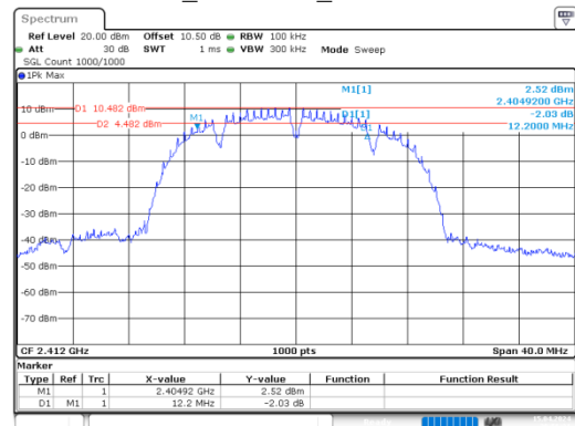
b_2412MHz_Chain 1
