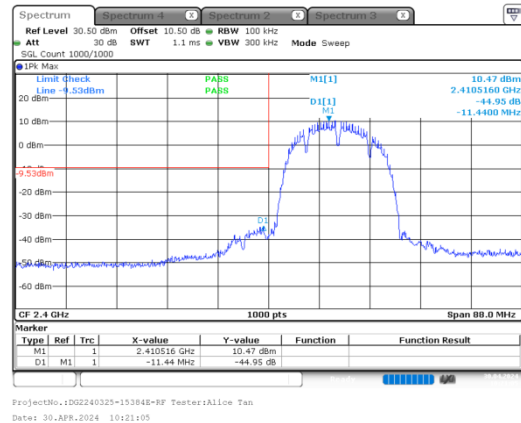
b_2412MHz_Chain 1
