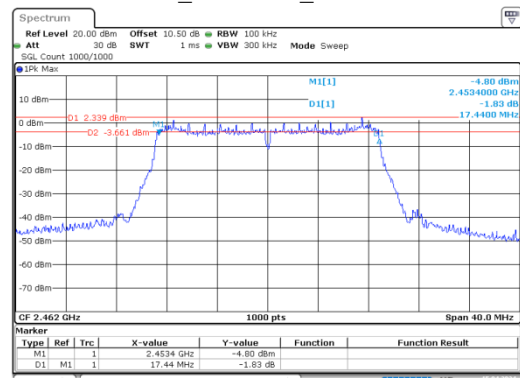
n20_2462MHz_Chain 1
