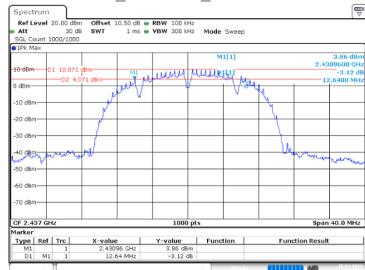
b_2437MHz_Chain 1
