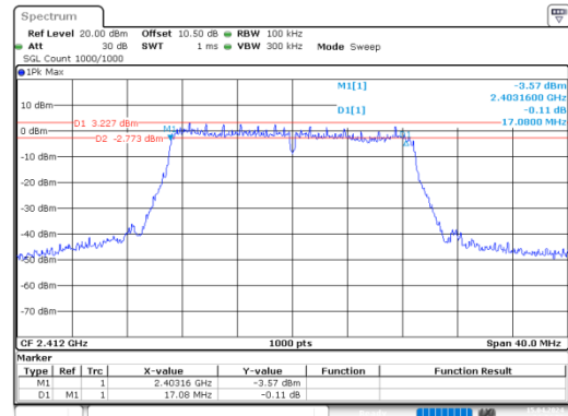
n20_2412MHz_Chain 1
