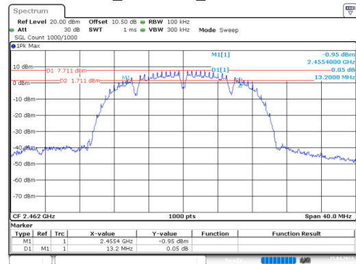
b_2462MHz_Chain 1
