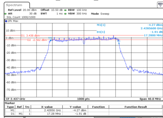
n20_2437MHz_Chain 1
