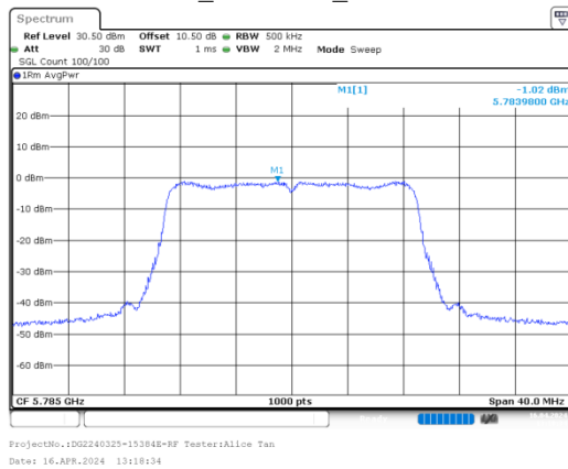
ac20_5785MHz_Chain 0
