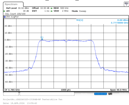
ac20_5785MHz_Chain 1
