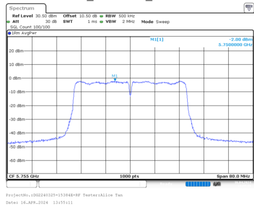
n40_5755MHz_Chain 1
