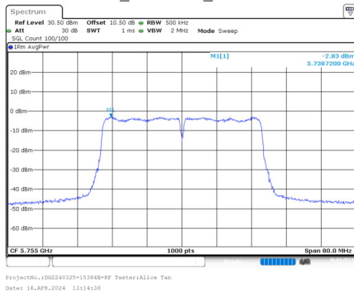
n40_5755MHz_Chain 0
