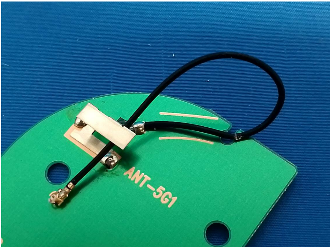
5GWifi Antenna(Chain 0)
