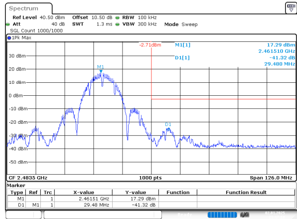
802.11b_2462MHz_Chain 0
