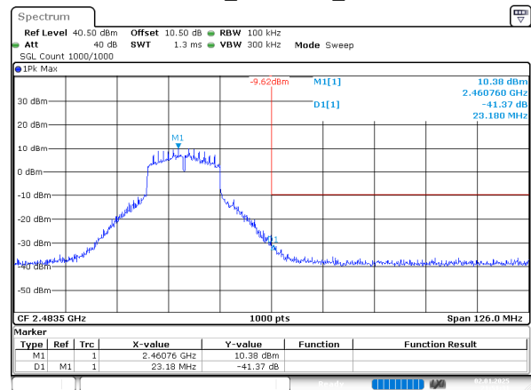
802.11n20_2462MHz_Chain 0
