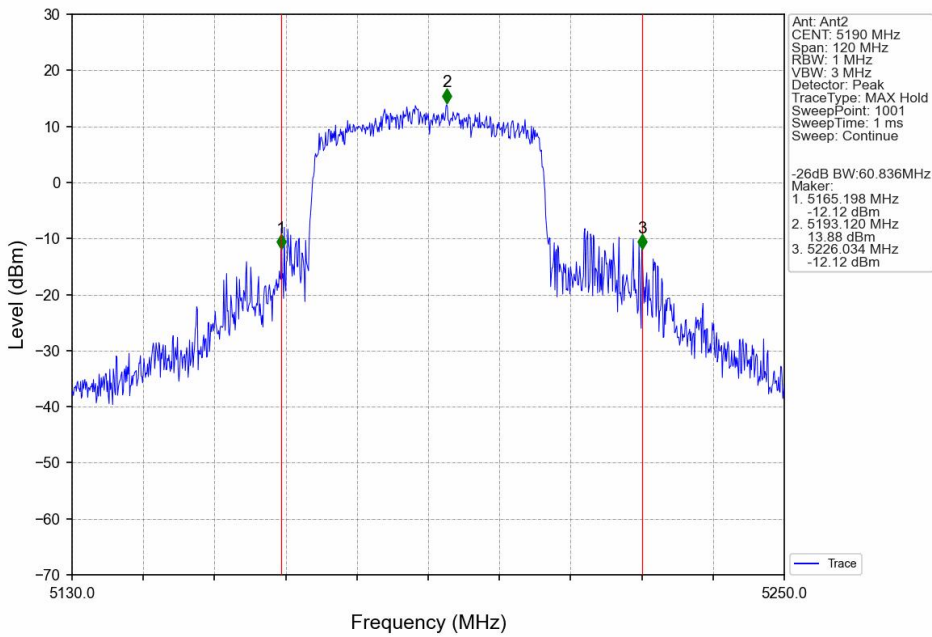
802.11be(EHT40)_LCH_5190MHz_SU_ / _Ant2_NTNV
