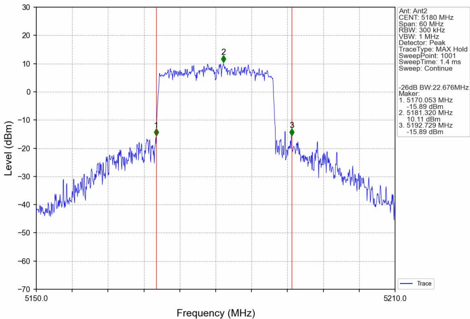
802.11be(EHT20)_LCH_5180MHz_SU_ / _Ant2_NTNV
