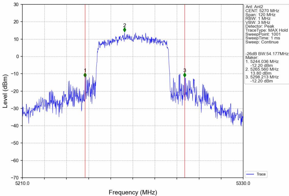
802.11be(EHT40)_LCH_5270MHz_SU_ / _Ant2_NTNV
